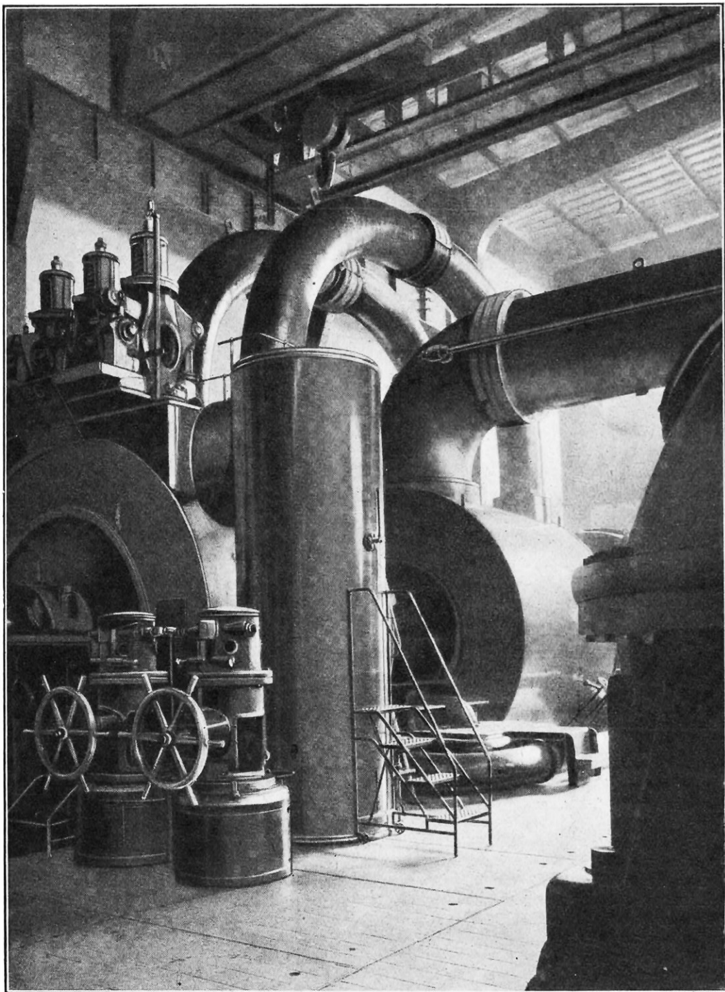
ENSEMBLE DES TURBINES HAUTE ET MOYENNE PRESSION D'UN GROUPE TURBO-GÉNÉRATEUR DE 80.000 KILOWATTS DE LA CENTRALE KLINGENBERG
