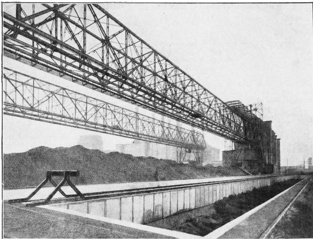
DE PUISSANTS ENGINS DE MANUTENTION MÉCANIQUE TRANSPORTENT CHAQUE HEURE LES 144 TONNES DE CHARBON NÉCESSAIRES AUX SEIZE CHAUDIÈRES DE LA CENTRALE
