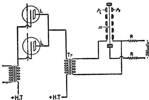
FIG. 13 ET 14. — L'OSZILLOPLAN, HAUT-PARLEUR ÉLECTROSTATIQUE DE GRANDE PUISSANCE (MAISON VOGT)
