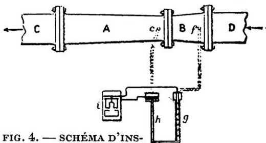
FIG. 4. — SCHÉMA D'INSTALLATION D'UN « TUBE VENTURI »
