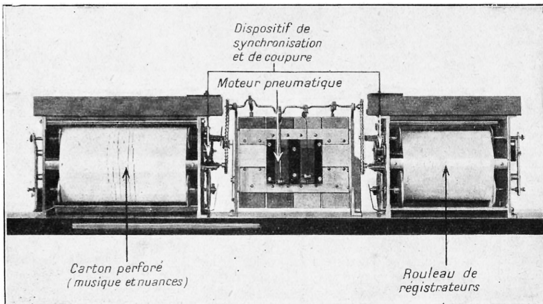
FIG. 9. — DÉTAIL DU MÉCANISME DE L'ORGUE AUTOMATIQUE
