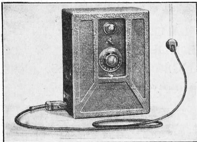
FIG. 1. — RÉCEPTEUR DEUX LAMPES DE LA COMPAGNIE « N ET K » ALIMENTÉ PAR LE SECTEUR
