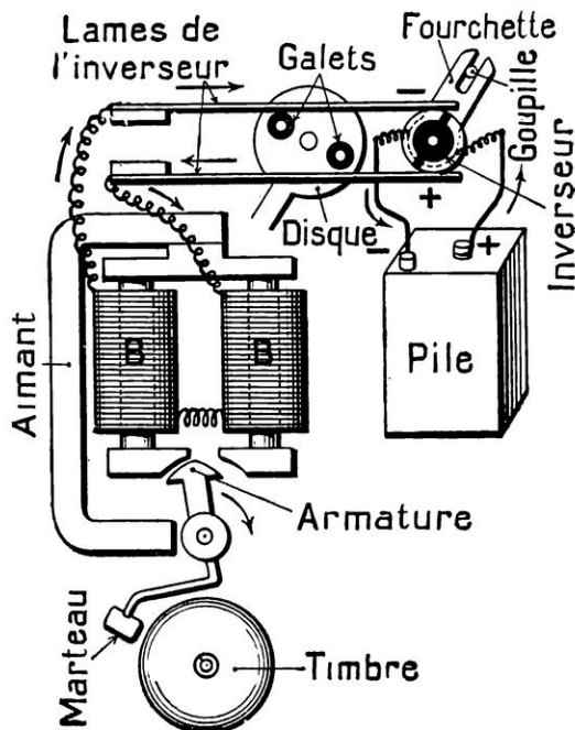
MÉCANISME DE LA SONNERIE
