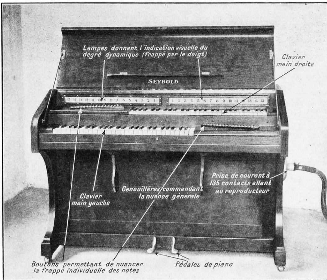
FIG. 10. — LE CLAVIER ANALYSEUR «SEYBOLD» PERMET DE PRÉPARER LES ROULEAUX PERFORÉS Le compositeur peut, grâce à cet appareil, tracer lui-même les perforations du papier et les nuancer pour chaque note en particulier, suivant des degrés que lui indiquent des lampes rangées au-dessus du clavier. Son jeu est inscrit automatiquement par un appareil enregistreur indépendant. Cet appareil, unique, est destiné à préparer les rouleaux du futur piano automatique du Conservatoire de Paris.
