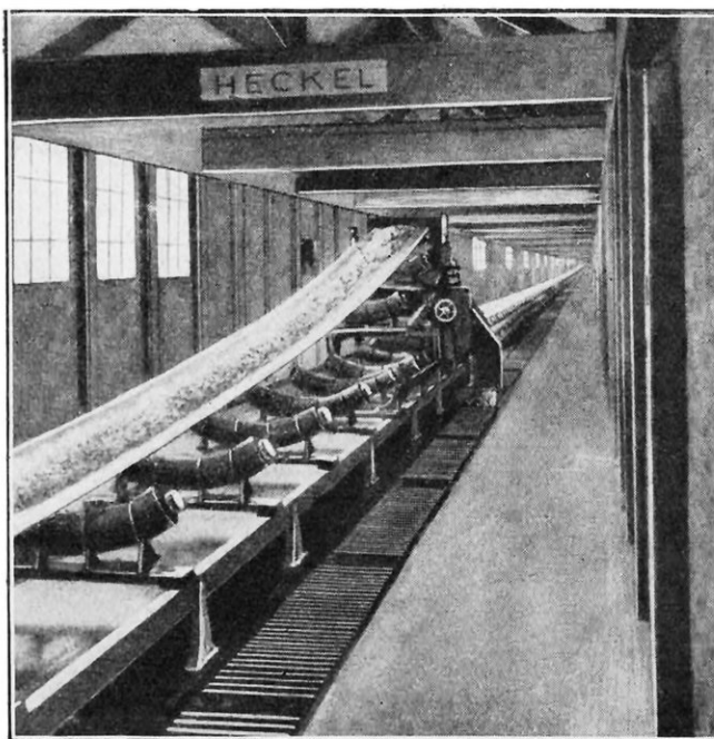
DES TAPIS ROULANTS TRANSPORTENT LA POTASSE VENANT DU CHALAND, SOIT VERS LES CARGOS DE MER, SOIT VERS LES MAGASINS DE STOCKAGE
