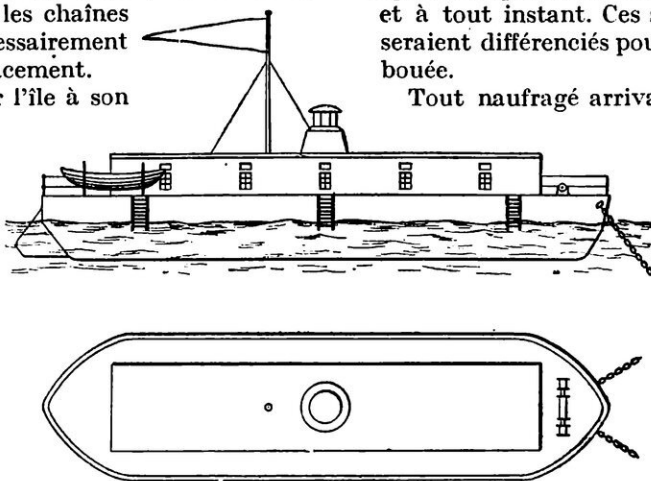
VUES EN PLAN ET ÉLEVATION D'UNE BOUÉE-RELAIS SUR UNE ROUTE AÉRIENNE MARITIME
