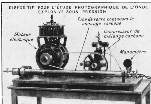
FIG. 3. — VUE D'ENSEMBLE DE L'APPAREIL UTILISÉ POUR ÉTUDIER PHOTOGRAPHIQUEMENT L'ONDE EXPLOSIVE SOUS PRESSION
