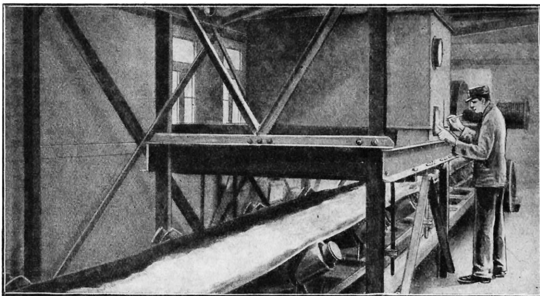
AUTOMATIQUEMENT ET D'UNE FAÇON CONTINUE, LA POTASSE CIRCULANT SUR LES BANDES TRANSPORTEUSES EST PESÉE SUR DES BASCULES, QUI TOTALISENT ET ENREGISTRENT LE POIDS DE SEL QUI EST PASSÉ SUR LA BANDE
