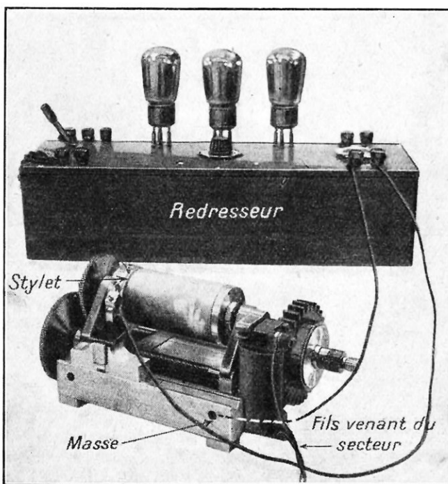
LE « BELINOGRAPHE » ET SON REDRESSEUR DE COURANT
