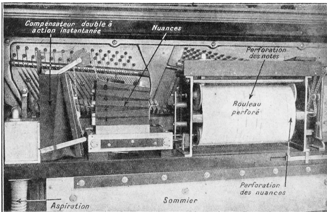
FIG. 5. — LA RÉALISATION DE L'APPAREIL DES NUANCES SCHÉMATISÉ PLUS HAUT (FIG. 2)
