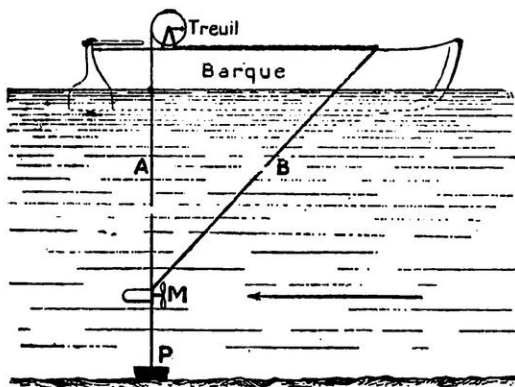
FIG. 2. - SCHÉMA D'INSTALLATION D'UN MOULINET DE JAUGEAGE SUR UN COURS D'EAU. Deux câbles, A et B, lestés par un saumon de plomb P, maintiennent en place le moulinet M à hélice. Des contacts à enregistrement électrique donnent les vitesses du courant, d'après un tirage effectué au préalable en traînant le moulinet à une vitesse connue dans une eau immobile.
