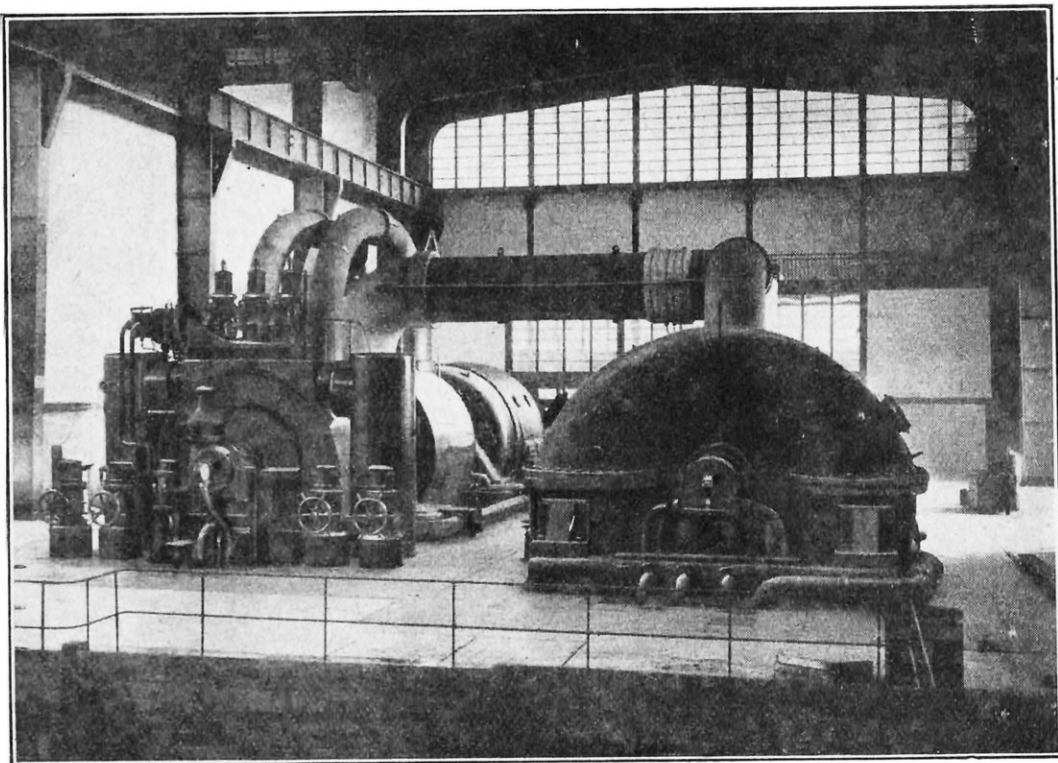
VUE EN BOUT D'UN GROUPE TURBO-GÉNÉRATEUR DE 80.000 kW
