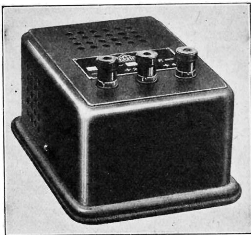
FIG. 9. — APPAREIL PERMETTANT L'ALIMENTATION D'UN POSTE SUR LE SECTEUR L'appareil fournit à la fois la tension de chauffage et la tension-plaque.
