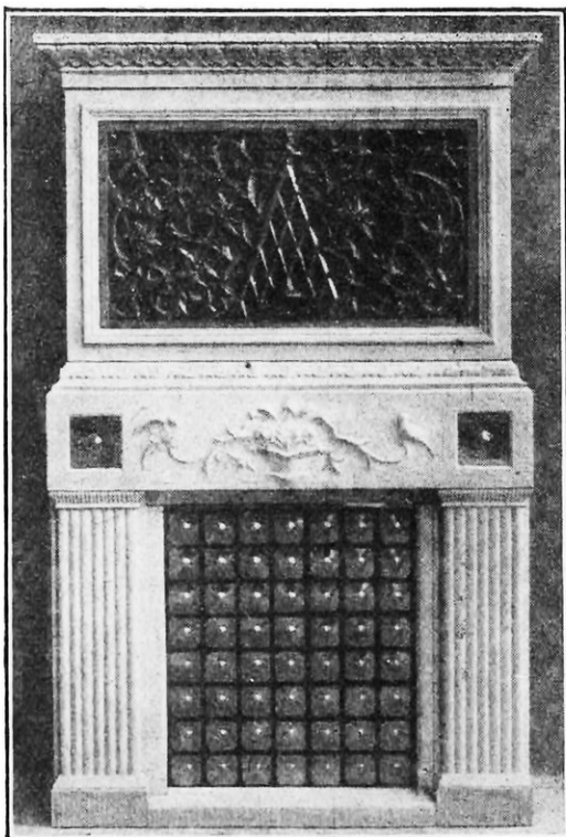
FIG. 10. — MODÈLE DE HAUT-PARLEUR DES ÉTABLISSEMENTS FUNCA, SPÉCIALEMENT ÉTUDIÉ POUR LES GRANDES SALLES
