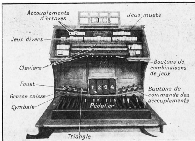
FIG. 8. - CONSOLE DES CLAVIERS D'UN ORGUE ÉLECTRIQUE
