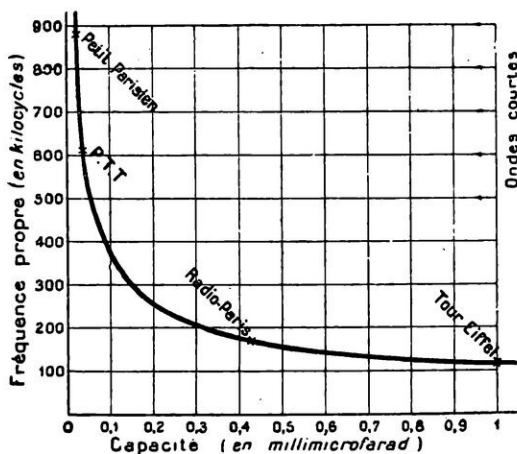
FIG. 14. — COMMENT VARIE LA FRÉQUENCE PROPRE D'UN CIRCUIT RÉCEPTEUR DE T. S. F. AVEC SA CAPACITÉ (LA SELF ÉTANT CONSTANTE) La courbe est identique à celle (fig. 5) qui donne la fréquence propre d'un fil à plomb en fonction de sa longueur.
