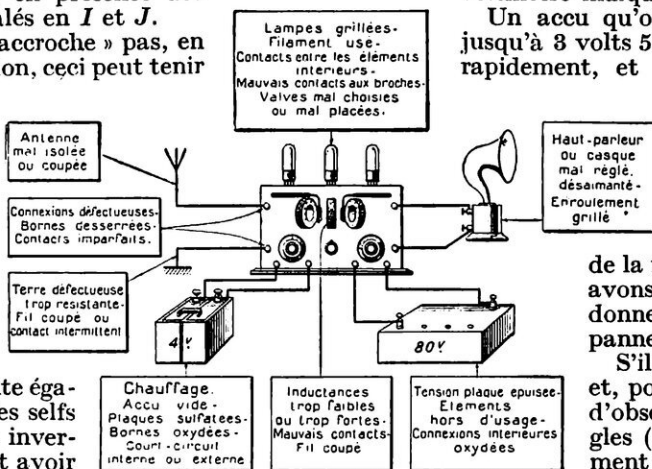
FIG. 1. — PANNES POUVANT SURVENIR DANS LES ORGANES EXTÉRIEURS D'UN POSTE DE T. S. F.
