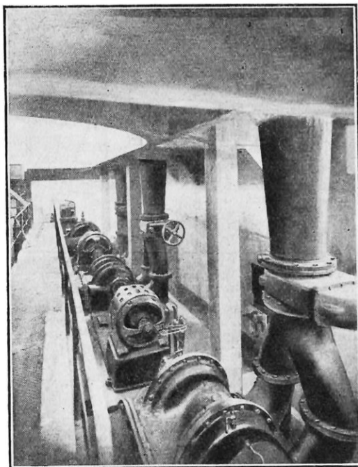
FIG. 6. — CETTE « STATION DE POMPAGE » COMPORTE DES POMPES CENTRIFUGES, DONT LA VITESSE DE ROTATION PERMET DE CRÉER DES PRESSIONS CORRESPONDANT A UNE CHUTE D'EAU DE 700 MÈTRES DE HAUTEUR
