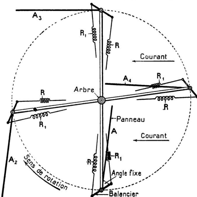
SCHÉMA DU FONCTIONNEMENT DES PALES
