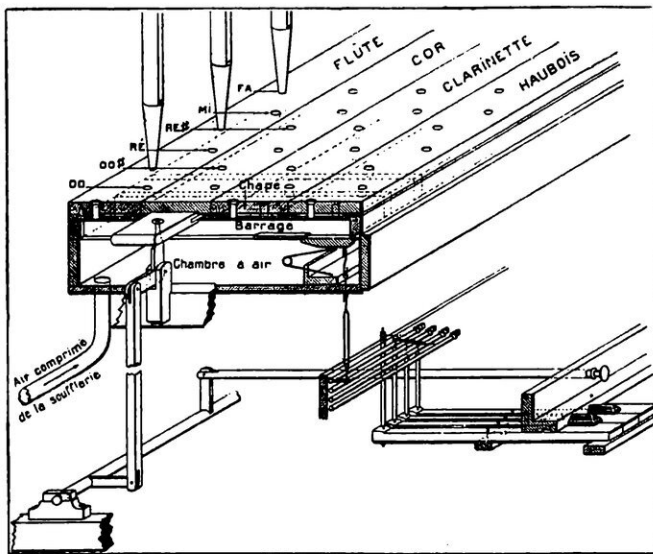
FIG. 6. — L'ANCIEN MÉCANISME DE L'ORGUE
