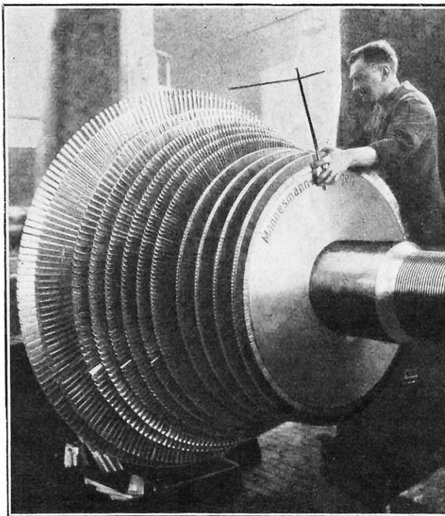
EN HAUT DE LA PAGE, AUBES FIXES DISTRIBUTRICES DE VAPEUR SUR LES AILETTES DE LA ROUE MOBILE DE LA PHOTOGRAPHIE DU BAS DE CETTE PAGE
