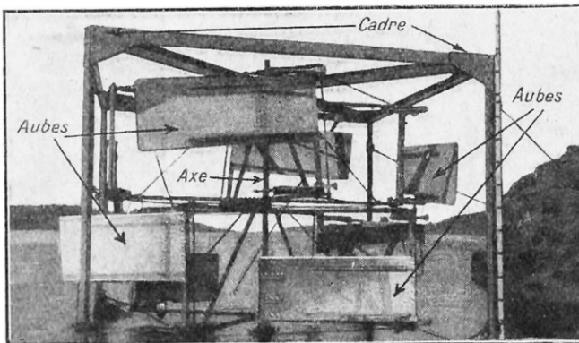
LA TURBINE MARINE AVANT SON IMMERSION
