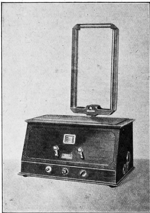
FIG. 8. — APPAREIL CHANGEUR DE FRÉQUENCE « DE TE WE » 8 LAMPES, QUI REÇOIT SUR CADRE LES POSTES EUROPÉENS
