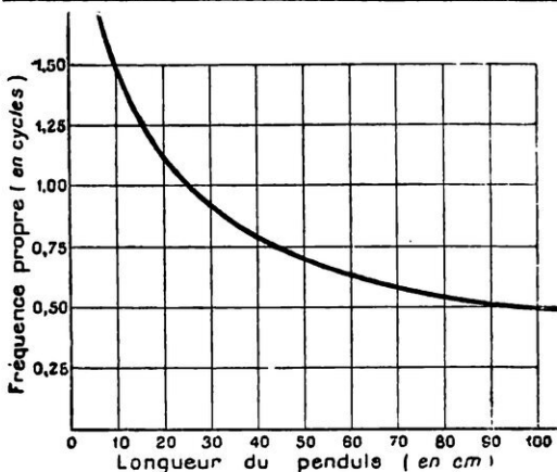
FIG. 5. — COMMENT VARIE LA FRÉQUENCE PROPRE D'UN FIL A PLOMB AVEC SA LONGUEUR
