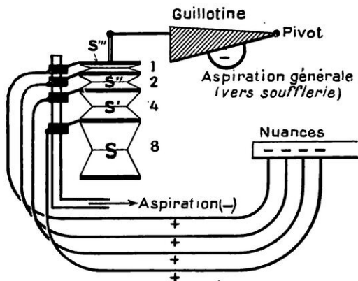
FIG. 2. — LE MÉCANISME DE L'APPAREIL PERMETTANT DE RÉALISER LES NUANCES
