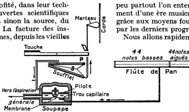
FIG. 1. — SCHÉMA DU PRINCIPE DU PIANO MÉCANIQUE
