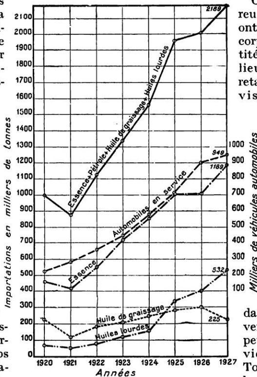
FIG. 1. — CE GRAPHIQUE MONTRE L'IMPORTANCE CROISSANTE DE LA CONSOMMATION FRANÇAISE DE COMBUSTIBLES LIQUIDES, EN RELATION ÉTROITE AVEC LE NOMBRE D'AUTOMOBILES EN SERVICE
