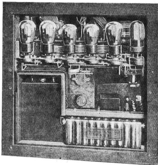
VUE INTÉRIEURE DU RÉCEPTEUR
