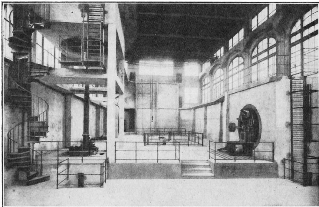
FIG. 5. - VUE INTÉRIEURE DE LA GRANDE SALLE DES ESSAIS DU LABORATOIRE, A BEAUVERT. On voit, à gauche, la tuyauterie utilisée pour les essais avec une chute de 8 mètres; à droite, une turbine est en essai sur la chute de 4 mètres de hauteur.
