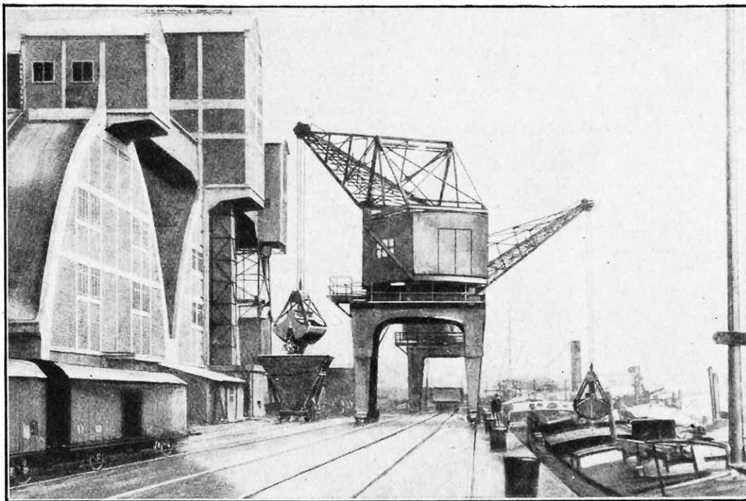
QUAI DE DÉCHARGEMENT OU LA POTASSE, PRISE DANS LES CHALANDS AU MOYEN DE BENNES PRENEUSES, EST DÉVERSÉE DANS DES TRÉMIES, D'OU, PAR DES TRANSPORTEURS A COURROIE ET DES ÉLÉVATEURS, ELLE EST AMENÉE AU FAITE DE L'INSTALLATION
