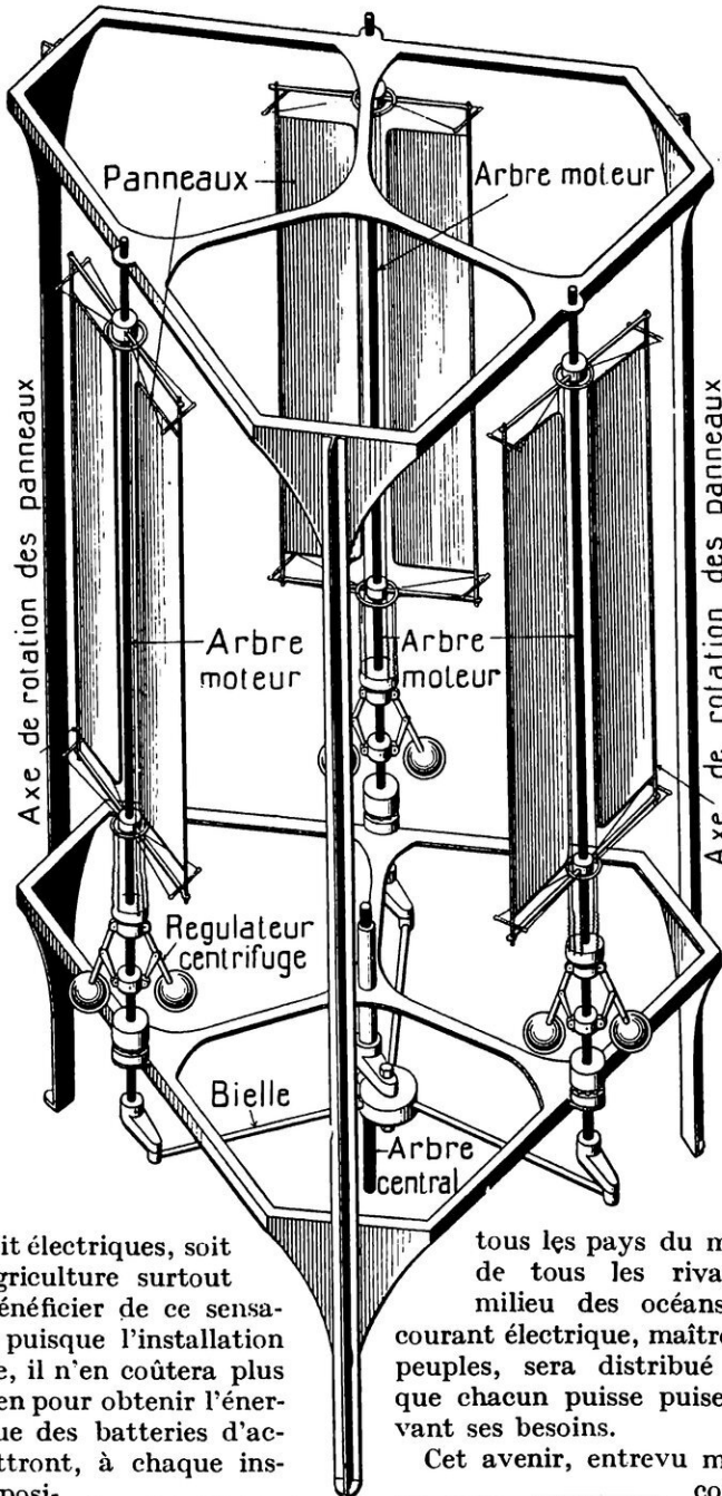
GROUPES DE TROIS TURBINES AÉRIENNES A UN SEUL ÉTAGE DESTINÉ À DES INSTALLATIONS PETITES ET MOYENNES
