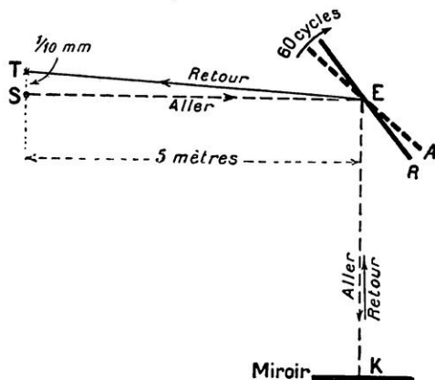
FIG. 16 ET 17. — UN FRÉQUENCÈMÈTRE EN DEUX MORCEAUX
