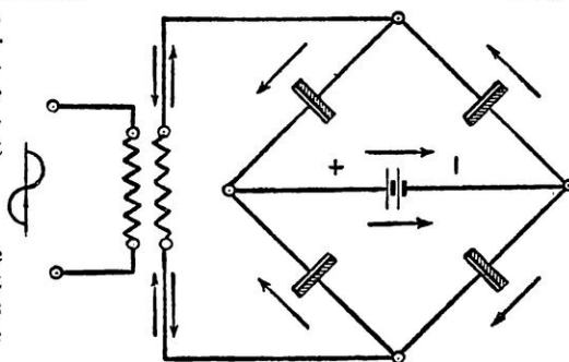
SCHEMA DE MONTAGE DU REDRESSEUR
