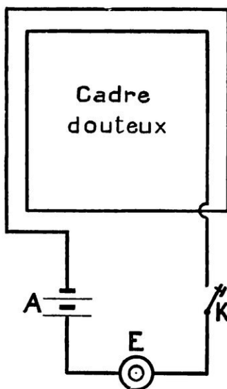
FIG. 2. — ESSAI D'UN CADRE OU D'UNE SELF
