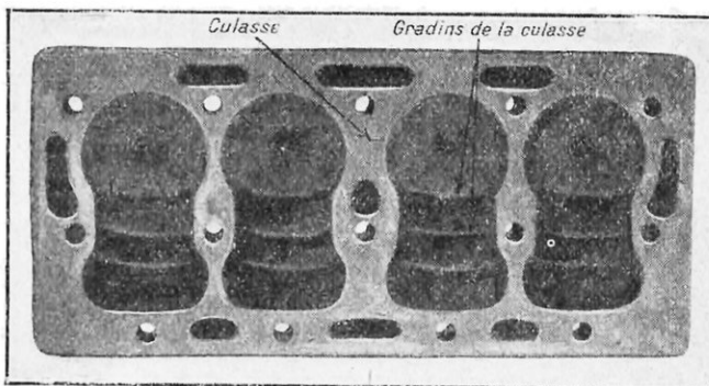
FIG. 4. — CULASSE DE MOTEUR A EXPLOSION DONT LE PIED EST EN FORME DE GRADINS SERVANT A BRISER L'ONDE EXPLOSIVE PAR DÉTENTE
