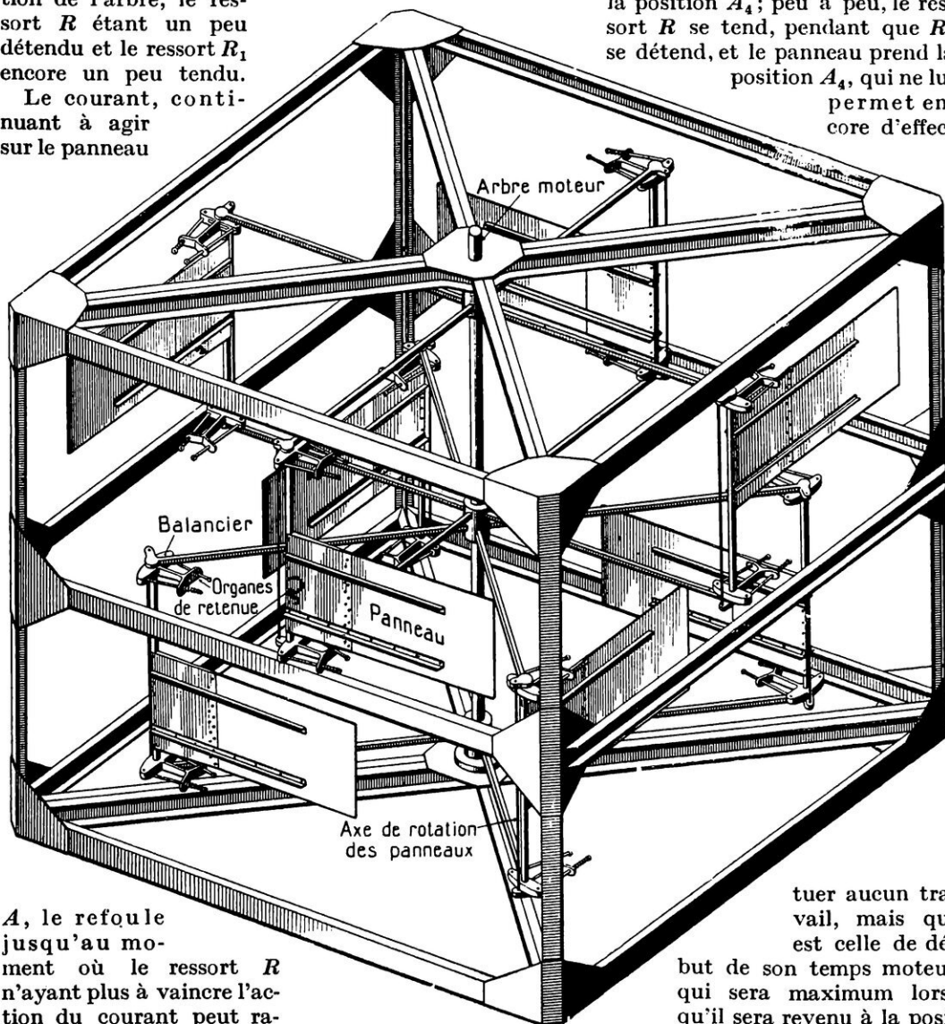
VUE PERSPECTIVE DE LA TURBINE HYDRAULIQUE ET MARÉMOTRICE Pour simplifier le dessin, les diverses commandes des pales ont été seulement amorcées.
