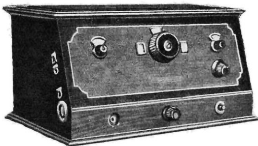
FIG. 7. — APPAREIL 6 LAMPES « DE TE WE », QUI PERMET D'ÉCOUTER EN HAUT-PARLEUR ET SUR ANTENNE LES POSTES EUROPÉENS
