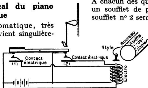
FIG. 11. — SCHÉMA DU MÉCANISME D'ENRE- GISTREMENT DES NUANCES
