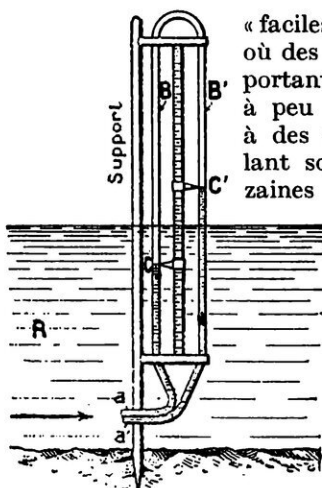
FIG. 3. - SCHÉMA D'UN TUBE DE PITOT-DARCY |
