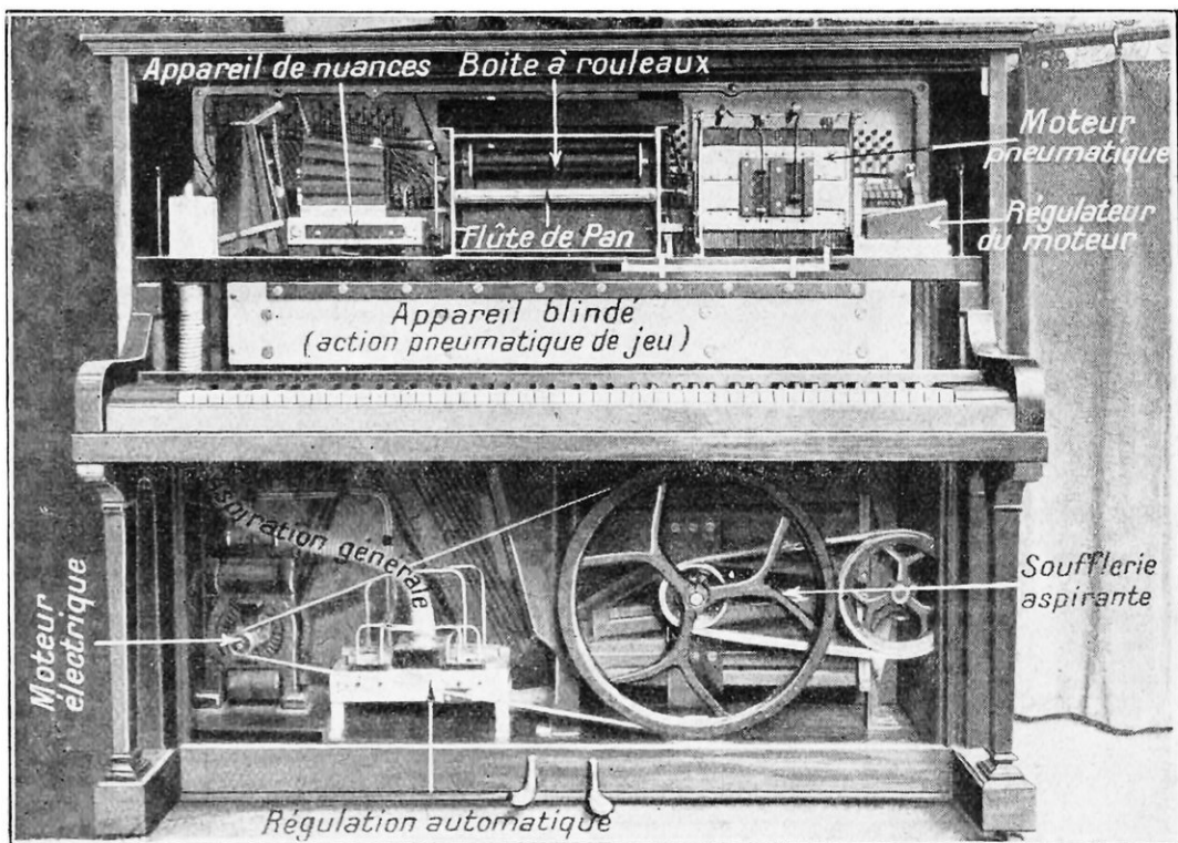
FIG. 4. — ENSEMBLE DU MÉCANISME D'UN PIANO MÉCANIQUE MODERNE
