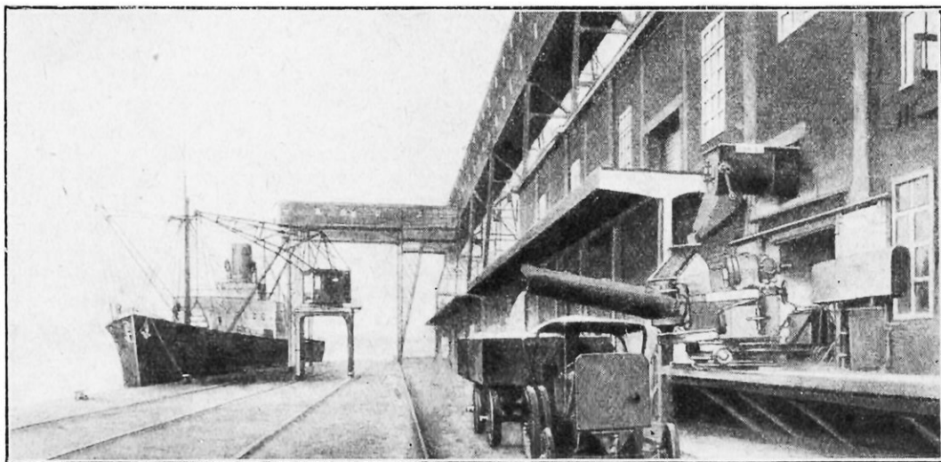
LORSQUE LA POTASSE DOIT ÊTRE CHARGÉE SUR WAGON, ELLE EST AMENÉE AU MOYEN D'UNE VIS SANS FIN, VISIBLE AU PREMIER PLAN, POUVANT S'ABAISSEUR OU SE RELEVER POUR REMPLIR UNIFORMÉMENT LE WAGON. AU FOND, CHARGEMENT D'UN CARGO (INSTALLATION HECKEL)
