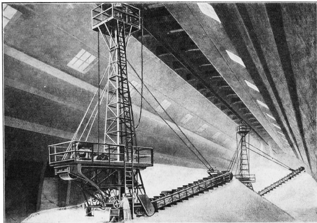
LE SEL POTASSIQUE EMMAGASINÉ ICI EST REPRIS AU MOYEN DE « GRATTEUSES », QUI LE FONT TOMBER SUR UNE BANDE TRANSPORTEUSE SITUÉE SOUS LE PLANCHER
