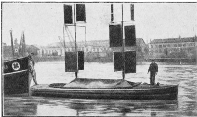
CE BATEAU A VOILES TOURNANTES A PU MARCHER CONTRE LE VENT GRACE AUX TURBINES AÉRIENNES THOMAS
