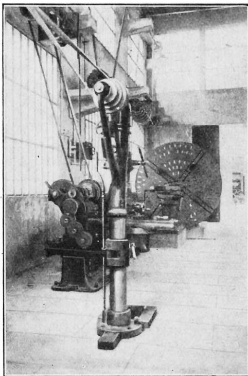
FIG. 7. — LE LABORATOIRE DE BEAUVERT COMPORTE UN ATELIER DE MÉCANIQUE ÉQUIPÉ DE MACHINES-OUTILS PERMETTANT DE FAIRE SUR PLACE LES RÉPARATIONS OU MODIFICATIONS NÉCESSAIRES AUX GROSSES TURBINES HYDRAULIQUES
