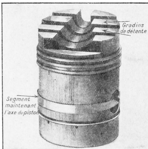
FIG. 5. — LE PISTON PRÉSENTE ÉGALEMENT UNE FORME EN GRADINS
