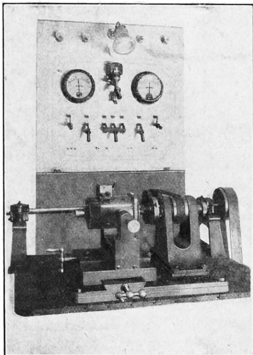
ENSEMBLE DU BANC D'ESSAIS POUR DYNAMOS D'AUTOMOBILES
