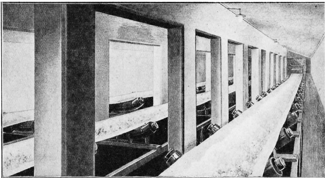
VOICI TROIS BANDES TRANSPORTEUSES QUI REÇOIVENT LA POTASSE « GRATTÉE » VENANT DES MAGASINS. CELLE-CI, REPRISSE PAR DES ÉLÉVATEURS ET DE NOUVEAUX TRANSPORTEURS A COURROIE, EST ENSUITE AMENÉE AUX CARGOS DE MER OU AUX WAGONS
