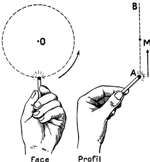
FIG. 3 ET 4. — RELATION ENTRE LES ROTATIONS ET LES VIBRATIONS
