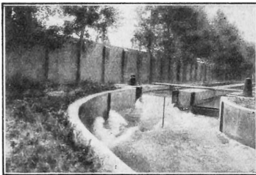
FIG. 8. — VUE DES DEUX CANAUX DE FUITE JUMELÉS POUR L'ÉVACUATION DES EAUX
