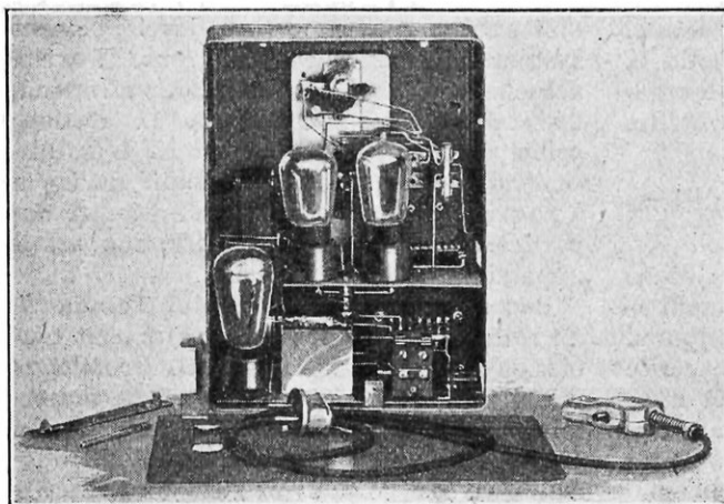
FIG. 2. — VUE INTÉRIEURE DU RÉCEPTEUR « N ET K » En bas et à gauche, la lampe redresseuse du courant.
