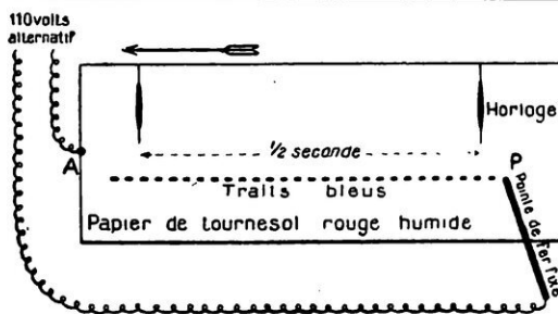
FIG. 12. — UN FRÉQUENCEMÈTRE POUR L'ALTERNATIF
