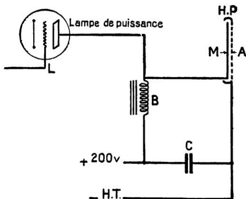
FIG. 15. — SCHÉMA DE HAUT-PARLEUR ÉLECTROSTATIQUE DE FAIBLE PUISSANCE
