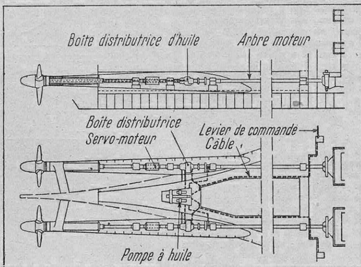
FIG. 2. — SCHÉMA DE PRINCIPE DE LA COMMANDE DE L'HÉLICE A PAS VARIABLE KAMOWA (GÖTAVERKEN)
