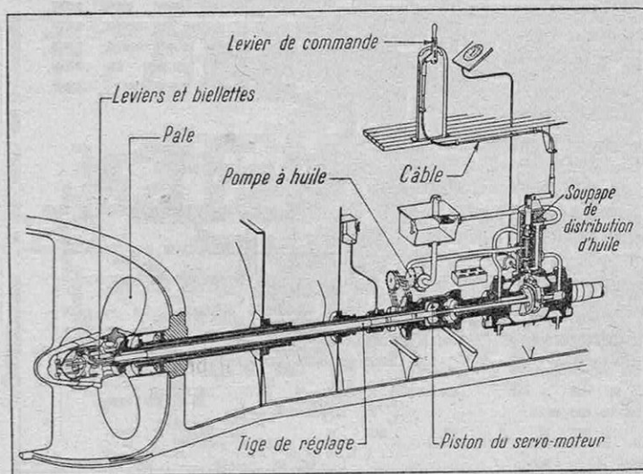
FIG. 1. — SCHÉMA DE PRINCIPE DE LA COMMANDE DE L'HÉLICE A PAS VARIABLE ESCHER WYSS
