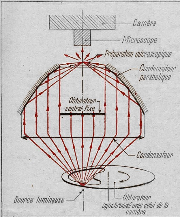
FIG. 3. — UN DES MONTAGES OPTIQUES PERMETTANT L'ÉCLAIRAGE LATÉRAL DES PRÉPARATIONS POUR L'ULTRAMICROSCOPIE
