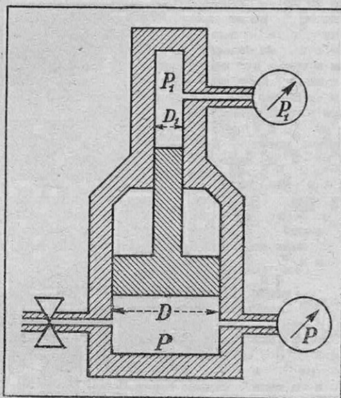
FIG. 3. — TARAGE DES MANOMÈTRES A ULTRAPRESSIONS
