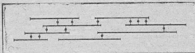
FIG. 8. — SCHÉMA DE LA VULCANISATION DU CAOUTCHOUC. Les traits allongés figurent les macromolécules, de longueurs d'atomes variables. Les points noirs représentent les atomes de soufre, formant des « ponts » entre macromolécules voisines.
