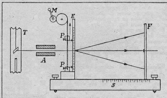
FIG. 2. — SCHÉMA D'UN SPECTROGRAPHE A ÉTIREMENT POUR L'ÉTUDE DU CAOUTCHOUC
