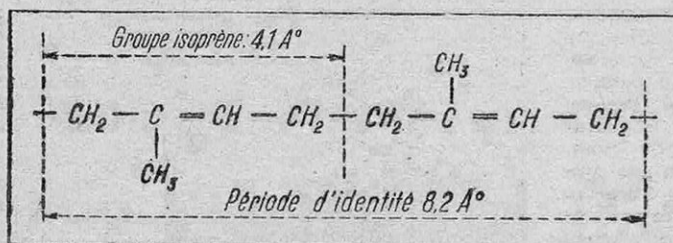
FIG. 5. — STRUCTURE SCHÉMATIQUE DE LA MOLÉCULE DE CAOUTCHOUC
