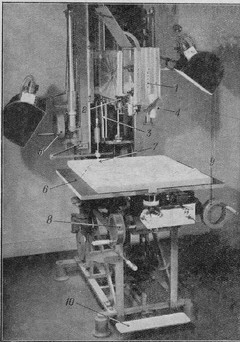
FIG. 12. — CAMÉRA SPÉCIALISÉE ET TABLE DE PRISE DE VUES SPÉCIALEMENT CONÇUE POUR LES FILMS SCIENTIFIQUES
