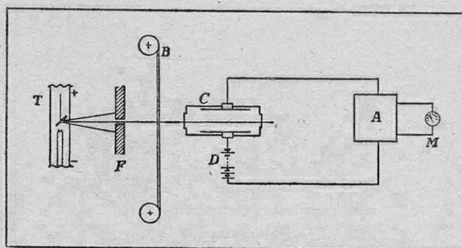
FIG. 9. — SCHÉMA DE LA MESURE DE L'HOMOGENÉITÉ D'UN CAOUTCHOUC INDUSTRIEL
