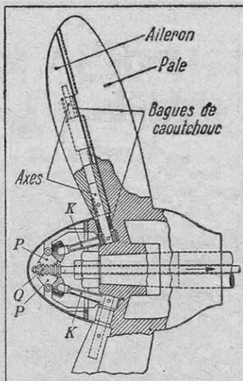
FIG. 3. — SCHÉMA DE L'HÉLICE STONE. K, BIELLETTES; P, SECTEUR DENTÉ; Q, CRÉMAILLÈRE.
