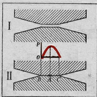
FIG. 2. — DISPOSITIF POUR L'OB- TENTION DE PRESSIONS DE L'OR- DRE DE 300 000 KG/CM 2
