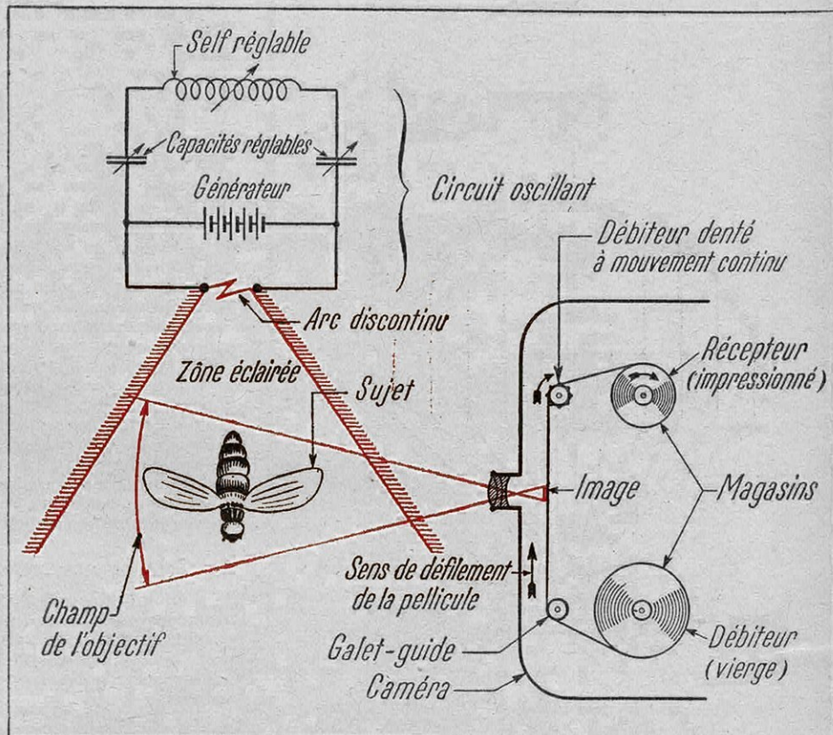
FIG. 2. — SCHÉMA DE PRINCIPE SIMPLIFIÉ D'UNE CAMÉRA POUR PRISES DE VUES ULTRARAPIDES
