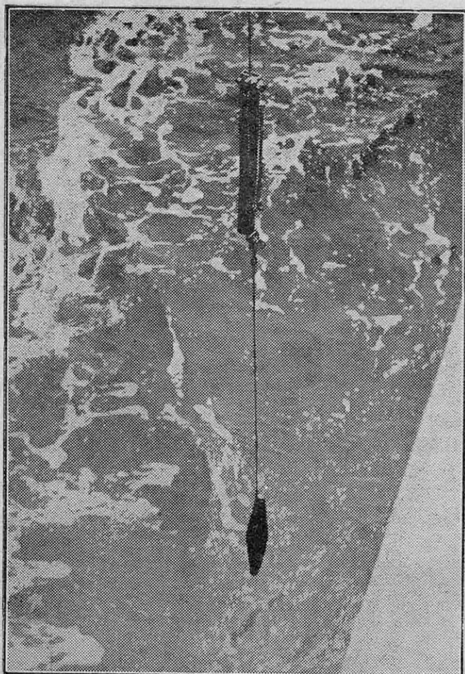
FIG. 4. — MISE A L'EAU D'UNE BOUTEILLE DE PRISE D'EAU AUTOMATIQUE POUR LE PRÉLEVEMENT D'ÉCHANTILLONS D'EAU A DIVERSES PROFONDEURS
