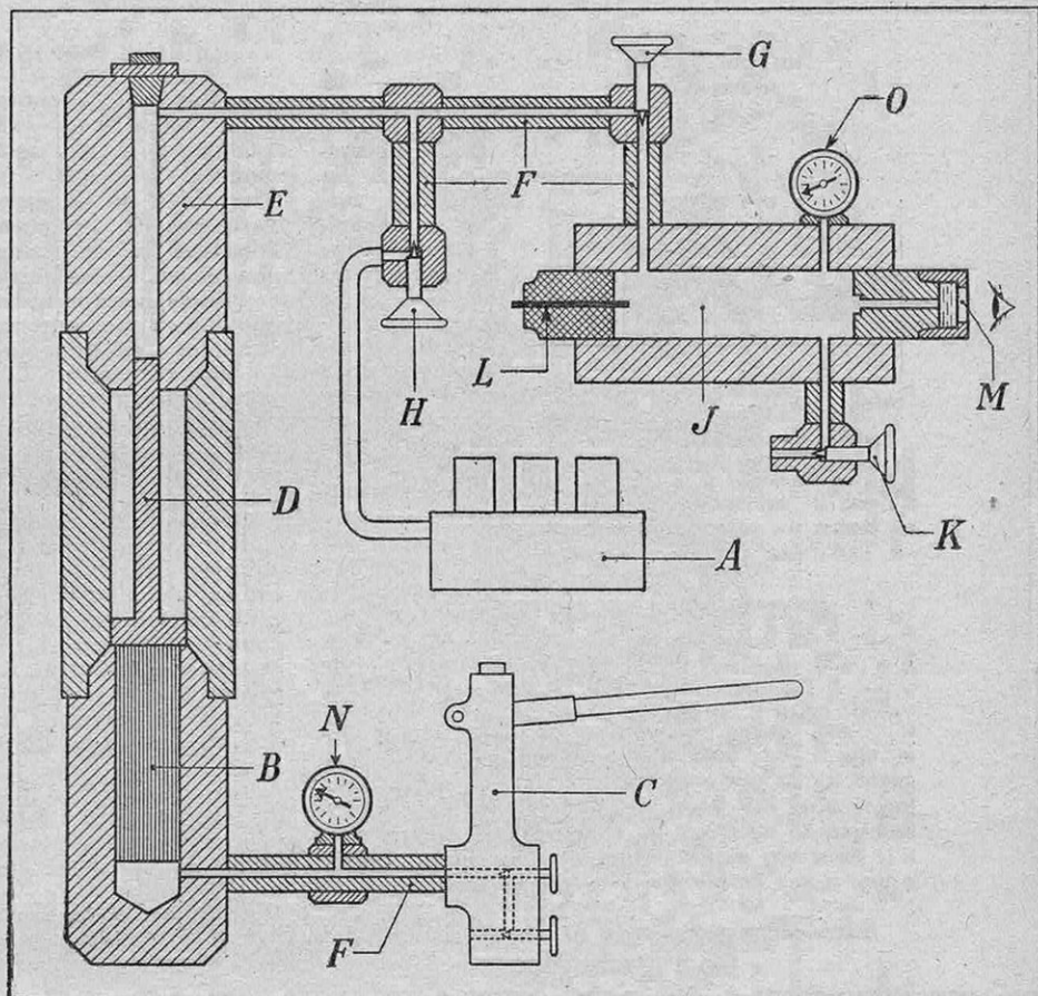
FIG. 1. — SCHEMA D'UN COMPRESSEUR DE GAZ POUR 25\,000\text{ kg/cm}^2
