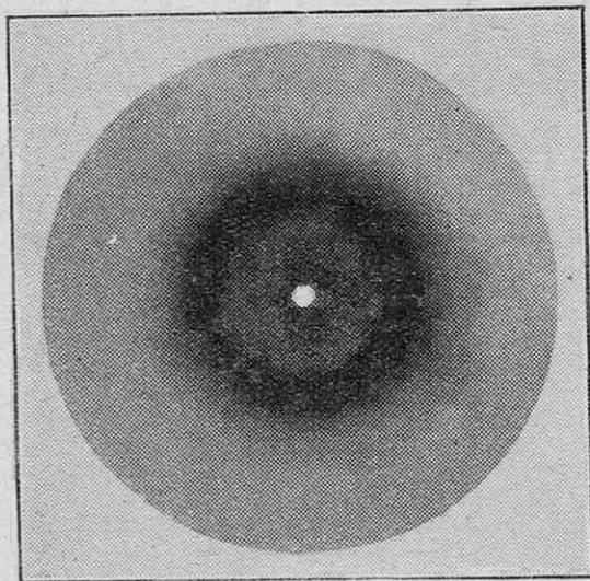
FIG. 3. — DIAGRAMME X DU CAOUTCHOUC NON ÉTIRÉ
