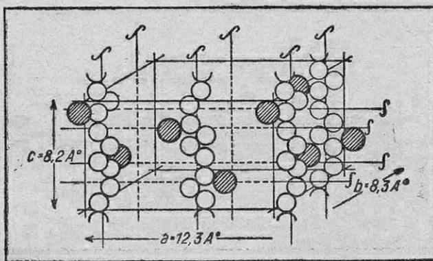
FIG. 7. — SCHÉMA DE LA CELLULE ÉLÉMENTAIRE DU CAOUTCHOUC. Ce serait une cellule orthorhombique (le système cristallin orthorhombique comporte trois axes de symétrie binaires; sa forme fondamentale est le prisme droit à base losange). L'axe C correspond à la direction de traction. La cellule contiendrait huit groupes isoprènes orientés parallèlement à cet axe et capables en outre de tourner autour de celui-ci. La densité calculée d'après ce modèle correspond bien à la densité réelle du caoutchouc, soit 0,92.
