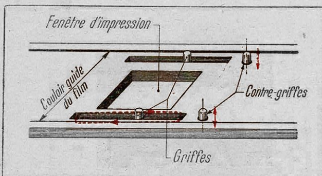
FIG. 7. — SCHEMA DU SYSTEME D'ENTRAINEMENT ET D'IMMOBILISATION DE LA PELLICULE DANS UNE CAMERA
