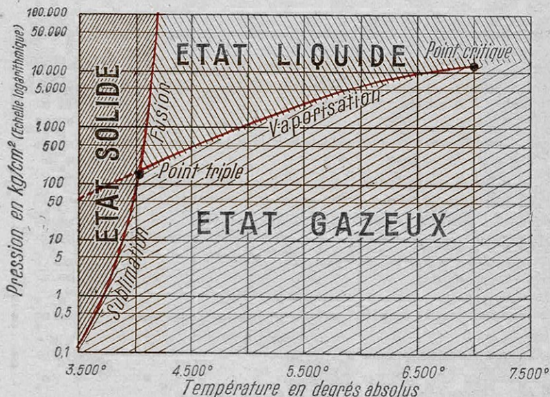
FIG. 4. — DIAGRAMME DES ÉTATS DU CARBONE (D'APRÈS BASSET)
