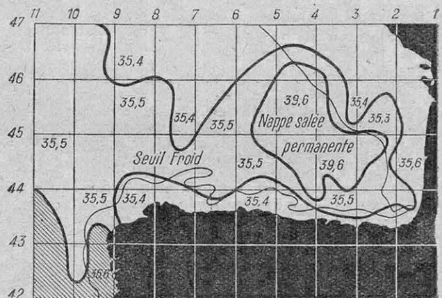
FIG. 2. — UNE NAPPE CHAUDE ET SALÉE FORME UNE PETITE MER AUTONOME DANS LE GOLFE DE GASCOGNE
