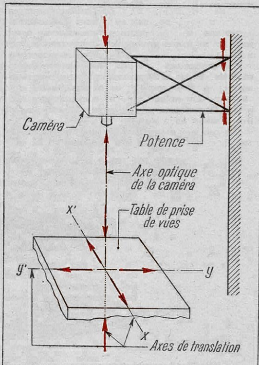
FIG. 9. — LES MOUVEMENTS QUE DOIT POUVOIR EFFECTUER LE MATÉRIEL DE PRISE DE VUES POUR L'ANIMATION DES DESSINS
