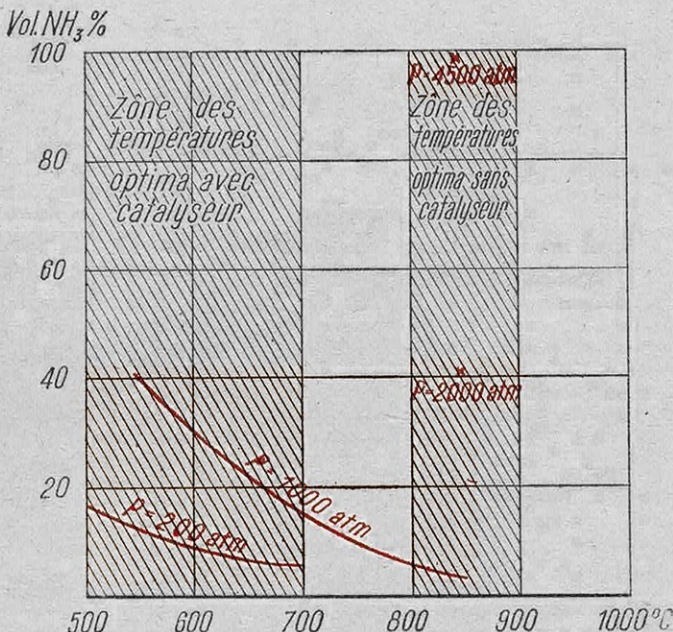
FIG. 5. — CONCENTRATIONS D'AMMONIAC RÉALISÉES A DIVERSES PRESSIONS ET TEMPÉRATURES
