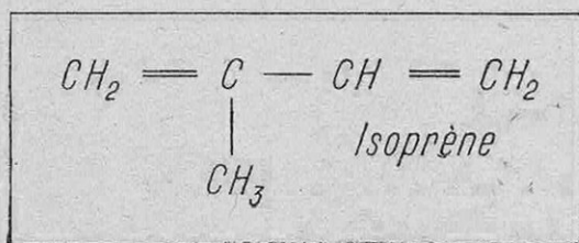
FIG. 1. — LA MOLÉCULE D'ISOPRÈNE, QUI SE SOUDE A D'AUTRES MOLÉCULES IDENTIQUES POUR FORMER LA LONGUE CHAÎNE DE LA MOLÉCULE GÉANTE DE CAOUTCHOUC
