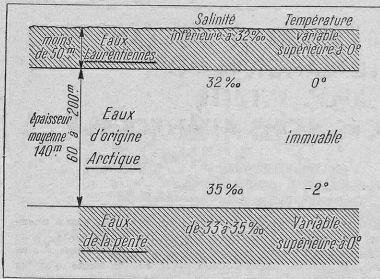
FIG. 1. — RÉPARTITION DE DIFFÉRENTES EAUX EN COUCHES SUPERPOSÉES DANS LE GOLFE DU SAINT-LAURENT
