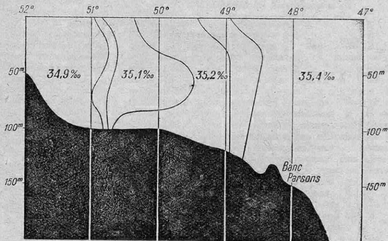
FIG. 5. — RÉPARTITION DES EAUX DE DIFFÉRENTES SALURES EN MURAILLES SUCCESSIVES QUASI VERTICALES AU BORD DU PLATEAU CONTINENTAL, EN HIVER, A PROXIMITÉ DE LA COTE D'ISLANDE
