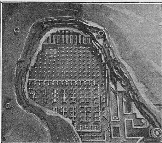
FIG. 1. — MAQUETTE DE LA SALLE SOUTERRAINE DE LA BANQUE DE FRANCE, COUPÉE À DIVERSES HAUTEURS. Cette salle de 1 hectare de superficie a été construite à environ 20 mètres de profondeur dans le calcaire et sous l'eau.
