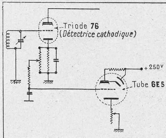
FIG. 7. — INDICATEUR VISUEL TYPE 6 E 5 SUIVANT UNE DÉTECTION CATHODIQUE
