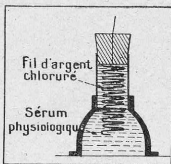
FIG. 15. — COUPE D'UNE ÉLECTRODE LIQUIDE DE MM. BAUDOIN, FISCHGOLD ET LERIQUE
