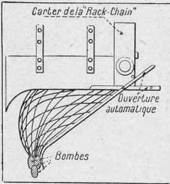
FIG. 5. — SCHÉMA MONTRANT COMMENT LE FILET SORT DE SON COFFRE DONT L'OUVERTURE EST DÉCLENCHÉE PAR LE PILOTE
