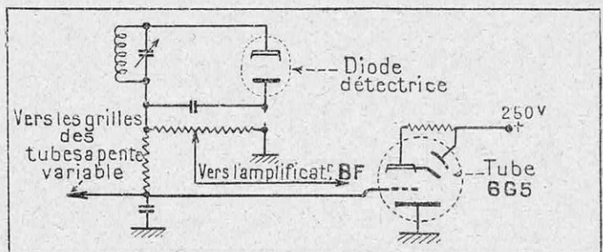
FIG. 4. — MONTAGE CLASSIQUE D'UN INDICATEUR VISUEL D'ACCORD TYPE 6 E 5 OU 6 G 5
