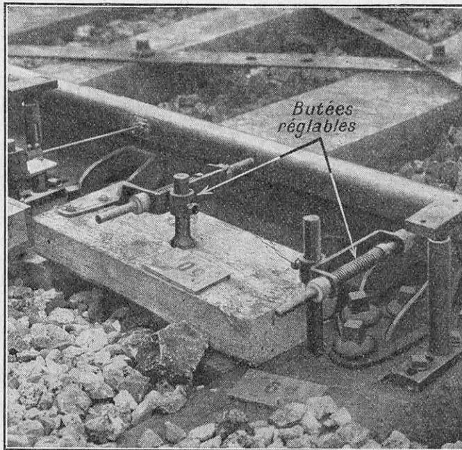
FIG. 9. — DÉTAIL DES BUTÉES RÉGLABLES DESTINÉES À LA MESURE DE LA DÉFORMATION DU RAIL
