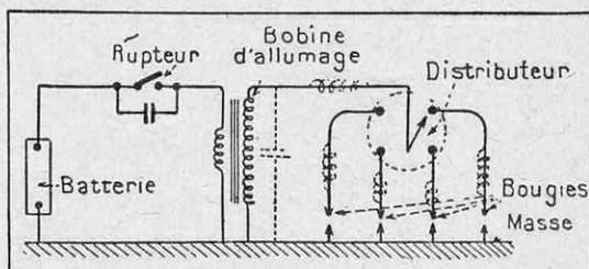
FIG. 1 ET 2. — SCHÉMAS DE PRINCIPE D'UN OSCILLATEUR HAUTE FRÉQUENCE A ÉTINCELLES (A GAUCHE) ET DU CIRCUIT D'ALLUMAGE D'UN MOTEUR A EXPLOSIONS (A DROITE)
