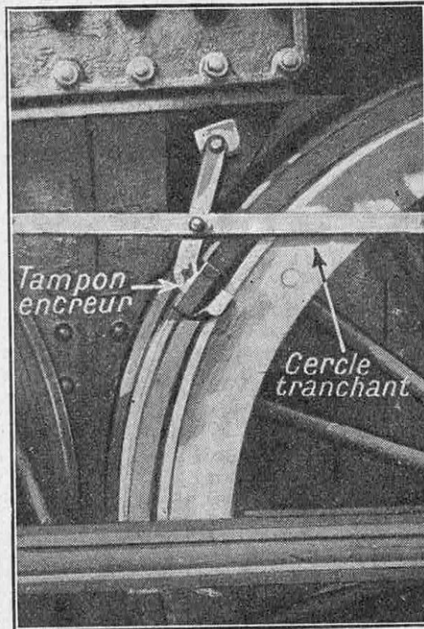
FIG. 10. — CERCLE TRANCHANT FIXÉ CONTRE UNE ROUE DE « MOUNTAIN » ET TAMPON ENCREUR POUR LA DÉTERMINATION DES POSITIONS EXACTES DES ROUES LORS DU PASSAGE D'UNE MACHINE EN COURBE
