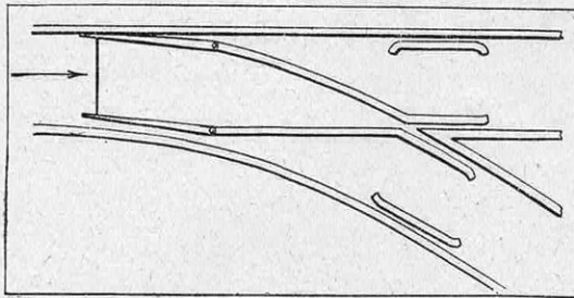
FIG. 1. — SCHEMA D'AIGUILLAGE SIMPLE Au droit du « cœur » de l'aiguille, le rail opposé est muni d'un contre-rail. Le boudin de la roue extérieure prend appui à revers sur ce contre-rail, pendant que la roue intérieure franchit le point où le rail intérieur est interrompu.
