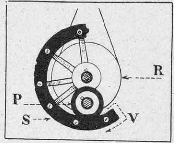
FIG. 4. — DÉTAIL DU DISPOSITIF DE RÉGLAGE
