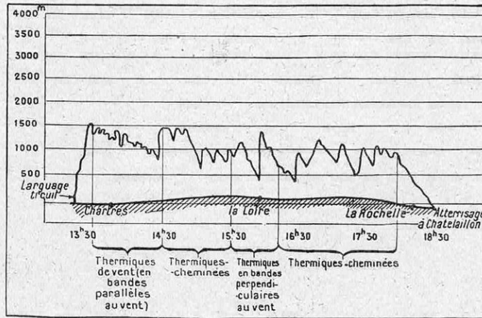
FIG. 11. — REPRODUCTION DU BAROGRAMME DU VOL DE RECORD DE NESSLER
