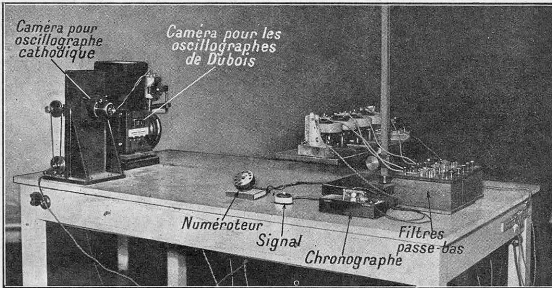
FIG. 2. — ENREGISTREMENT DES ÉLECTROENCÉPHALOGRAMMES MULTIPLES SUR UN FILM Un faisceau lumineux éclaire les miroirs des oscillographes qui renvoient chacun son spot particulier sur le film unique qui se déroule derrière la fente de la chambre noire.
