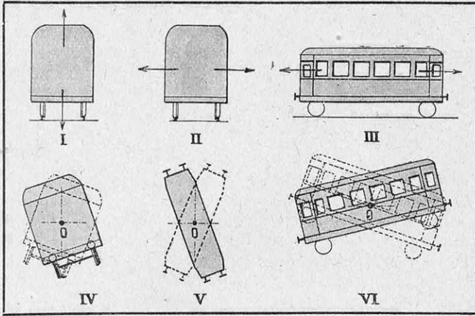
FIG. 3. — LES SIX OSCILLATIONS PRINCIPALES DU MATÉRIEL ROULANT DE CHEMIN DE FER
