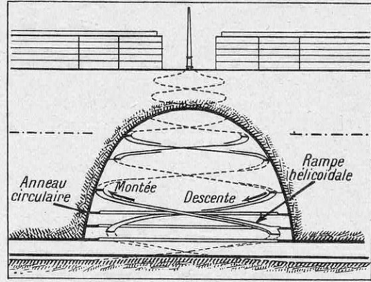
FIG. 9. — PROJET DE M. TCHUMI POUR ASSURER LA LIAISON ENTRE LES VOIES SOUTERRAINES DE PARIS ET LA SURFACE DU SOL. Cette liaison serait assurée par rampes hélicoïdales et pourrait être installée à toutes les places et grands carrefours de la capitale.
