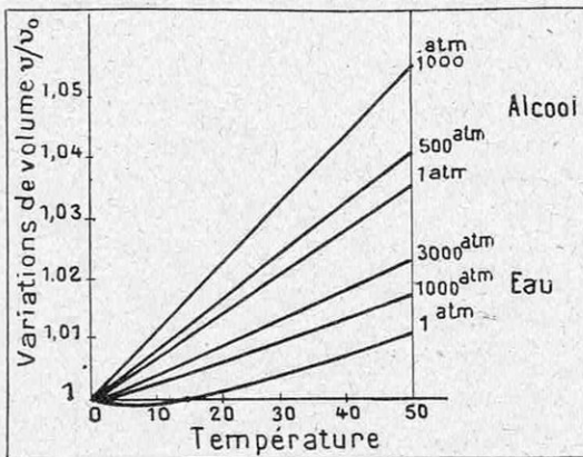
FIG. 2. — VARIATIONS DE VOLUME COMPARÉES DE L'EAU ET DE L'ALCOOL AVEC LA TEMPÉRATURE A DIVERSES PRESSIONS
