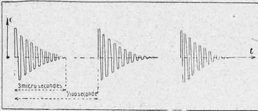
FIG. 3 — ALLURE GÉNÉRALE DES ONDES AMORTIES QUI PRENNENT NAISSANCE DANS LE CIRCUIT D'ALLUMAGE DES MOTEURS
