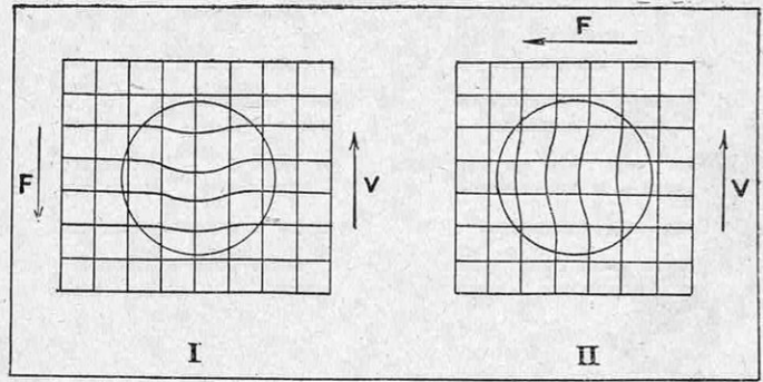
FIG. 5. — DÉFORMATION SUPERFICIELLE DU RAIL AU PASSAGE D'UNE ROUE MOTRICE (I) ET SOUS L'ACTION DE LA FORCE CENTRIFUGE (II)
