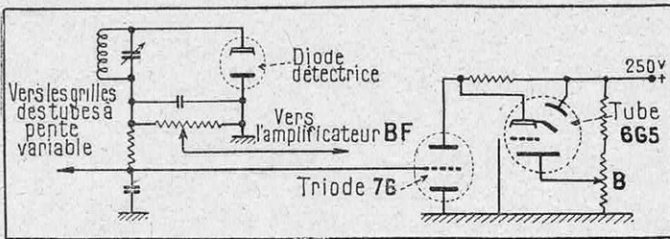
FIG. 5. — MONTAGE D'UN INDICATEUR VISUEL D'ACCORD TYPE 6 E 5 OU 6 G 5 AVEC SECTEUR D'OMBRE DE 180°
