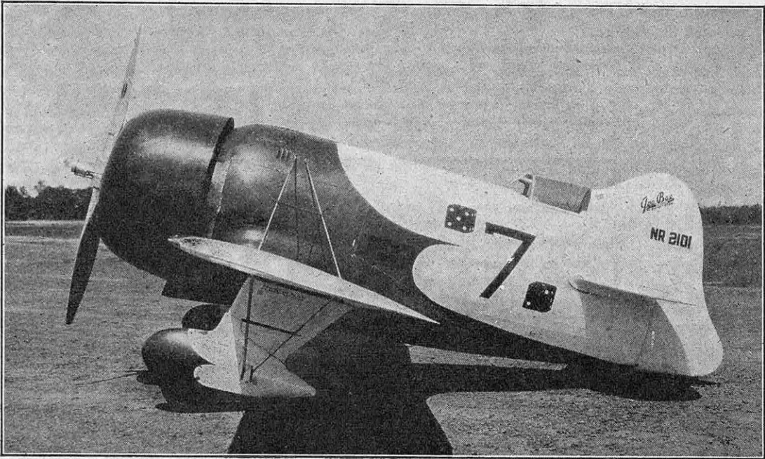
FIG. 7. — LE GEE BEE « SUPER SPORSTER » DE DOOLITTLE (1932)
