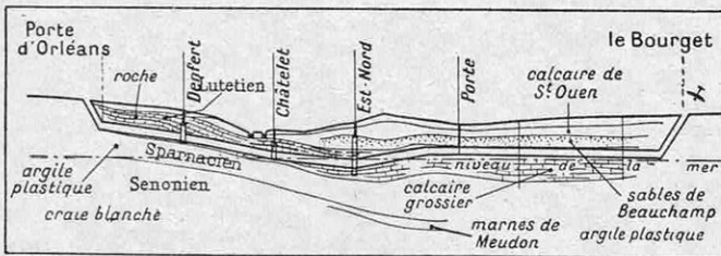
FIG. 8. — COUPE DU SOUS-SOL PARISIEN ENTRE LE BOURGET ET LA PORTE D'ORLÉANS (SUD DE PARIS)
