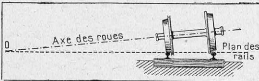
FIG. 4. — POSITION DU « CENTRE INSTANTANÉ DE ROTATION » D'UN ESSIEU QUI N'EST PAS EXACTEMENT AU MILIEU DE LA VOIE
