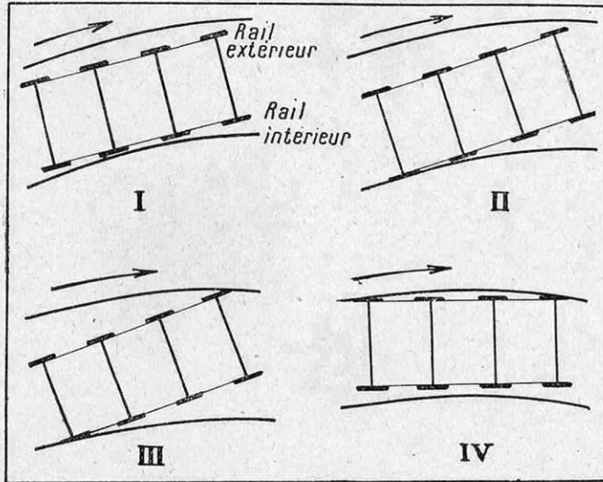
FIG. 11. — POSITIONS CARACTÉRISTIQUES D'UNE « MOUNTAIN » LORS D'UN PASSAGE EN COURBE
