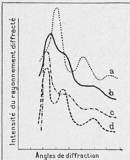
FIG. 4. — COURBES DE DIFFRACTION POUR LES RAYONS X DU TÉTRACHLORURE DE CARBONE (a), DE L'EAU (b), DU QUARTZ (c) ET DE LA TRIDYMITE (d)
