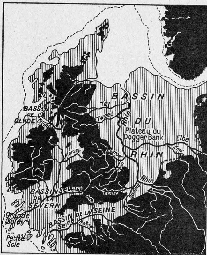
FIG. 4. — LA CARTE SOUS-MARINE DU BLOC « FRANCO-BRITANNIQUE » A L'ÉPOQUE PLÉISTOCÈNE
