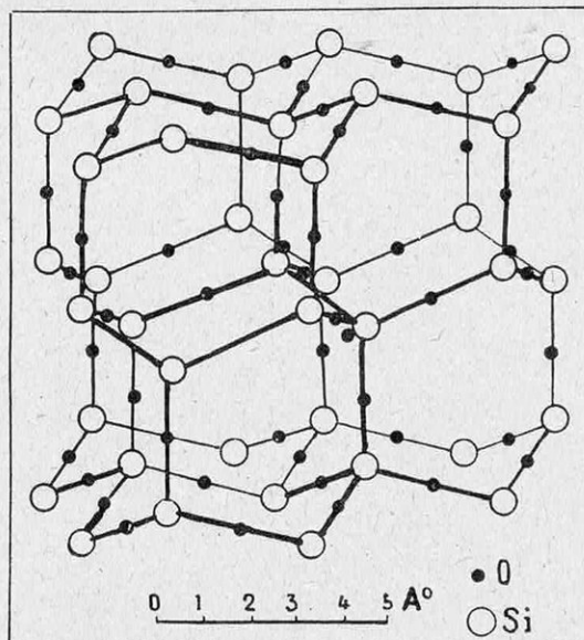
FIG. 5. — STRUCTURE DE LA TRIDYMITE, VARIÉTÉ DE SILICE CRISTALLISÉE
