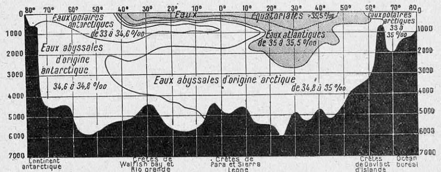
FIG. 8. — COUPE TRANSVERSALE DE L'Océan ATLANTIQUE MONTRANT LA RÉPARTITION DES EAUX D'ORIGINES DIFFÉRENTES
