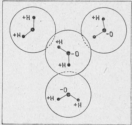
FIG. 7. — FORME TÉTRAÉDRIQUE DE L'ASSOCIATION DE MOLÉCULES D'EAU
