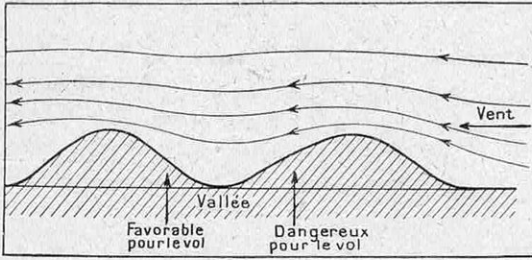
FIG. 4. — SCHÉMA DE LA STRUCTURE DU VENT AU PASSAGE D'UN OBSTACLE COMPORTANT UNE VALLÉE
