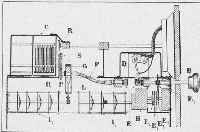
FIG. 3. — SCHÉMA DU DISPOSITIF DE RÉGLAGE UNIQUE
