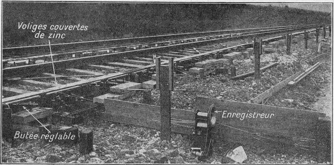
FIG. 8. — VUE D'ENSEMBLE DE L'ÉQUIPEMENT DE LA VOIE POUR L'ÉTUDE DU COMPORTEMENT DES LOCOMOTIVES « MOUNTAIN » EN COURBE
