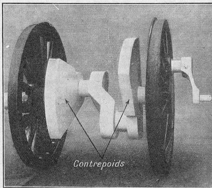
FIG. 2. — ESSIEU COUDÉ DE LOCOMOTIVE « ATLANTIC » DE FORME CLASSIQUE (EN HAUT), ET AUTO-ÉQUILIBRÉ, TYPE « CHAN » (EN BAS)
