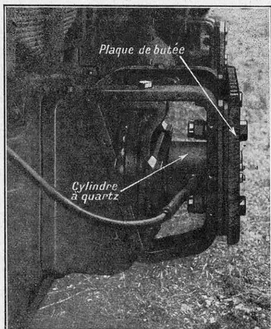
FIG. 6. — QUARTZ PIÉZOÉLECTRIQUE INSTALLÉ DANS LE PROLONGEMENT D'UN ESSIEU POUR LA MESURE DES EFFORTS EXERCÉS SUR LES ROUES PAR LES RAILS
