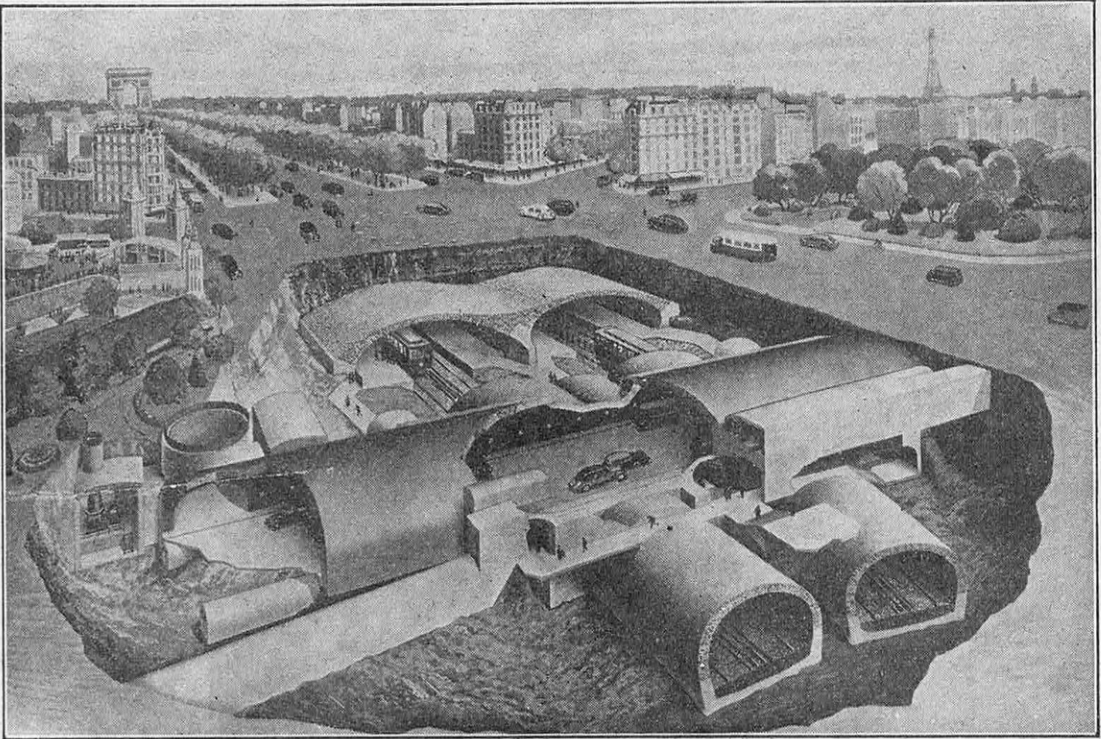
FIG. 2. — L'AMÉNAGEMENT SOUTERRAIN DE LA PORTE MAILLOT A PARIS
