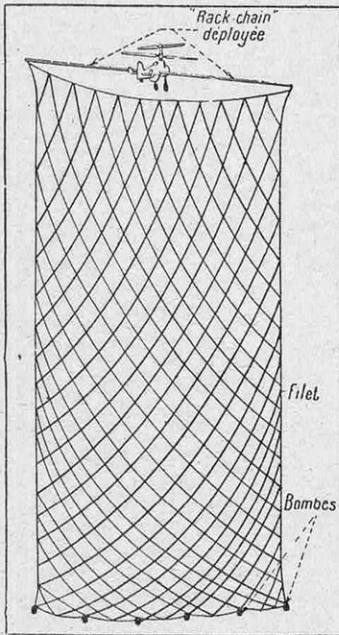
FIG. 6. — VOICI LE FILET DÉPLOYÉ MAINTENU PAR LES BRAS TRÈS RIGIDES DE LA « RACK-CHAIN »
