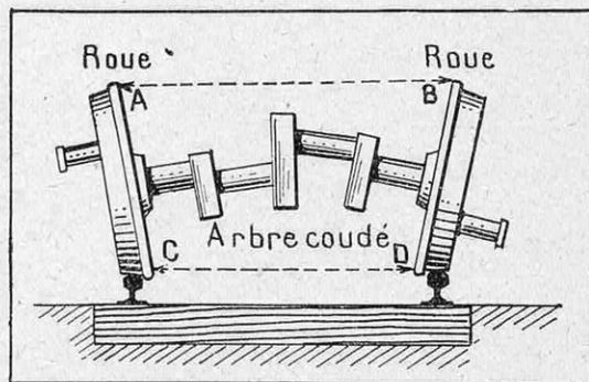
FIG. 7. — ESSIEU COUDÉ D'« ATLANTIC » OU DE « MOUNTAIN » DÉFORMÉ SOUS L'ACTION DES EFFORTS CENTRIFUGES AB peut arriver à surpasser CD de 18 mm.
