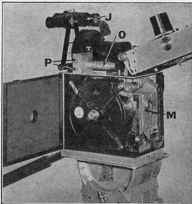
FIG. 5. — L'APPAREIL CINÉMATOGRAPHIQUE « ASKANIA » QUI A ÉTÉ UTILISÉ POUR LE CONTRÔLE DES RÉCENTS RECORDS DE VITESSE ÉTABLIS EN ALLEMAGNE
