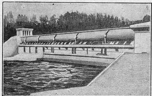
FIG. 2. — VUE DE LA CENTRALE HYDROÉLECTRIQUE SOUS-FLUVIALE INSTALLÉE A STEINBACH (ALLEMAGNE), D'UNE PUISSANCE DE 10 000 CHEVAUX, SOUS 9 MÈTRES DE CHUTE
