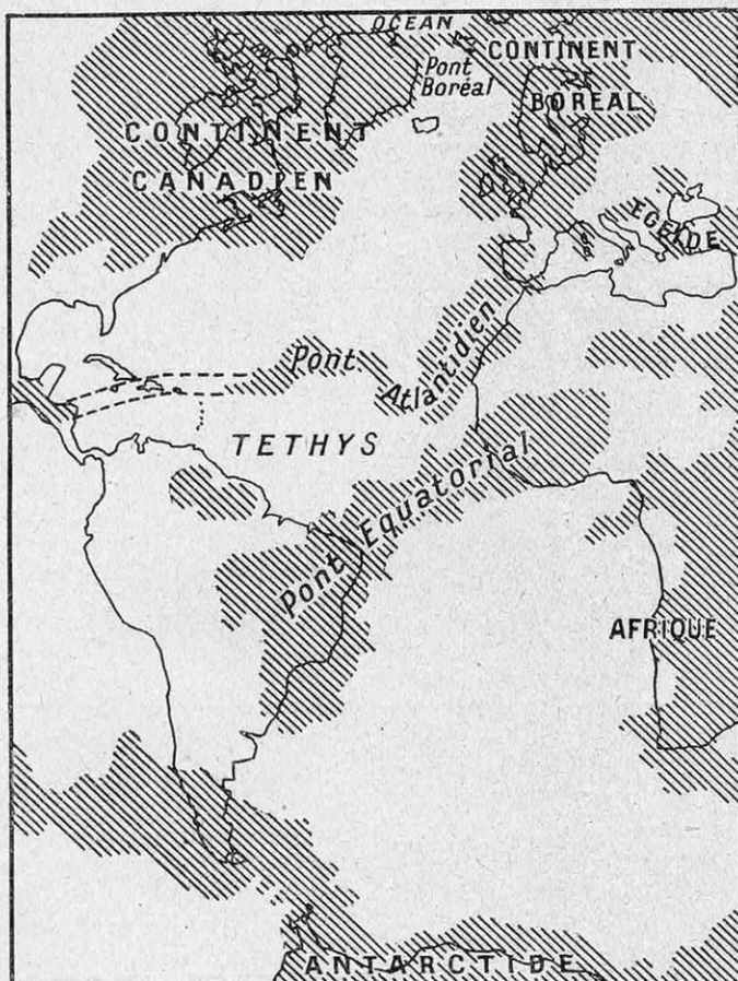
FIG. 5. — LES « PONTS » CONTINENTAUX A TRAVERS L'ATLANTIQUE A LA FIN DE L'ÈRE PRIMAIRE
