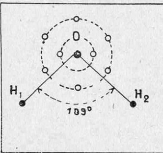
FIG. 6. — REPRÉSENTATION DE LA MOLÉCULE D'EAU
