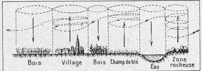
FIG. 5. — DISPOSITION DES COURANTS ASCENDANTS ET DESCENDANTS D'ORIGINE THERMIQUE
