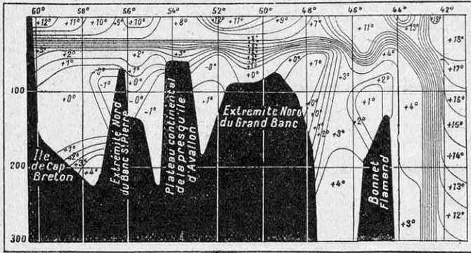
FIG. 7. — L'IMMIXIBILITÉ DES EAUX
