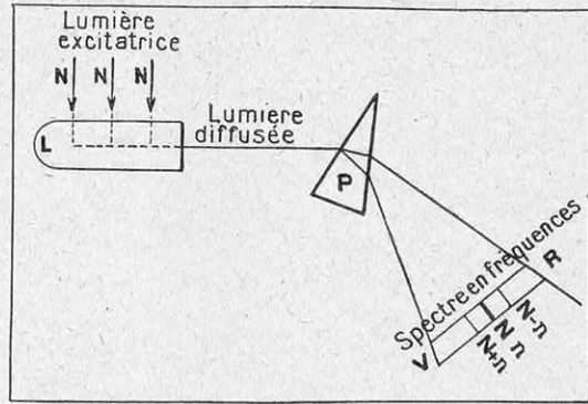
FIG. 3. — COMMENT ON MET EN ÉVIDENCE L'EFFET RAMAN
