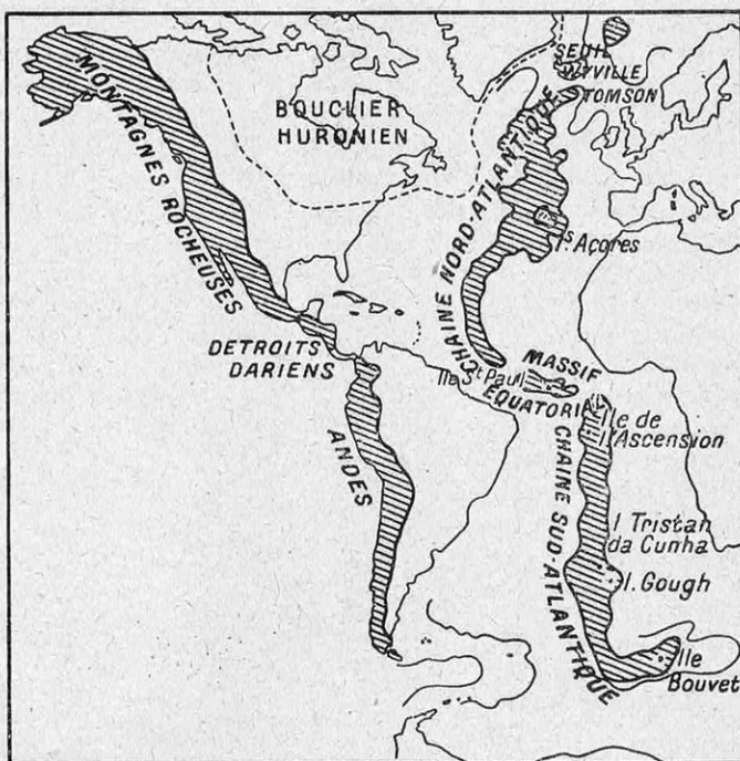
FIG. 3. — CARTE DU RELIEF SOUS-ATLANTIQUE
