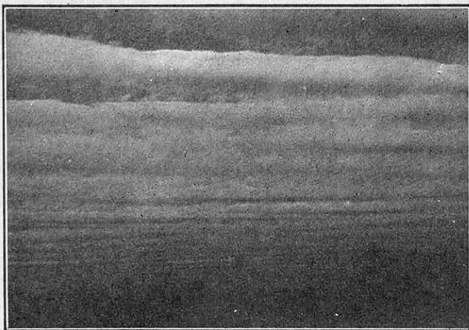
FIG. 10. — NUAGES EN BANDES PARALLÈLES FORMANT DES « RUES DE NUAGES »
