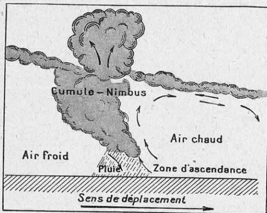
FIG. 8. — DISPOSITION SCHÉMATIQUE DES NOMBREUX COURANTS AÉRIENS QUI CIRCULENT DEVANT LES FRONTS D'ORAGE
