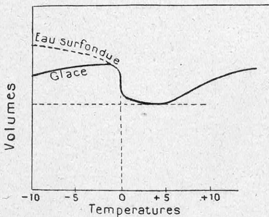
FIG. 1 — VARIATIONS DU VOLUME DE L'EAU AU VOISINAGE DU POINT DE FUSION
