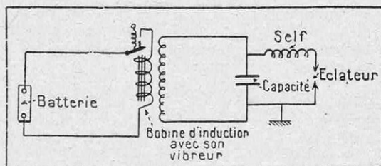
FIG. 1 ET 2. — SCHÉMAS DE PRINCIPE D'UN OSCILLATEUR HAUTE FRÉQUENCE A ÉTINCELLES (A GAUCHE) ET DU CIRCUIT D'ALLUMAGE D'UN MOTEUR A EXPLOSIONS (A DROITE)
