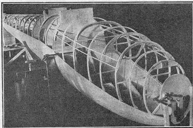
FIG. 12. — LE FUSELAGE DU PLANEUR MONOTYPE OLYMPIQUE « MEISE », SUR SON BÂTI DE MONTAGE
