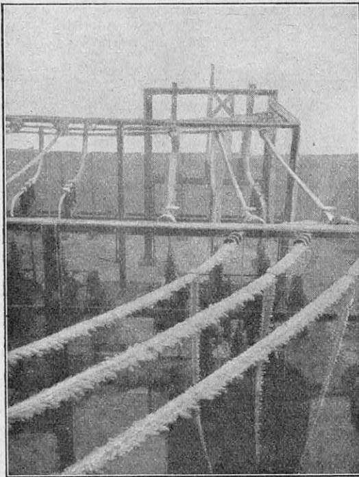
FIG. 3. — CETTE PHOTOGRAPHIE MONTRE L'IMPORTANCE DE LA SURCHARGE MÉCANIQUE QU'IMPOSE PARFOIS LE GIVRE AUX CONDUCTEURS DES LIGNES DE TRANSPORT DE FORCE
