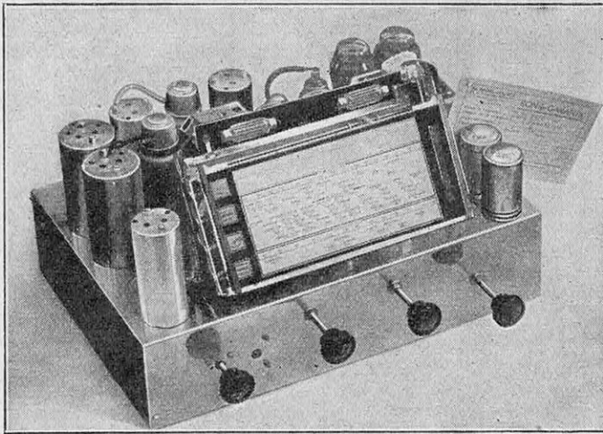
LE « P. B. 1936 », TYPE SALON, DE RADIO-SOURCE
