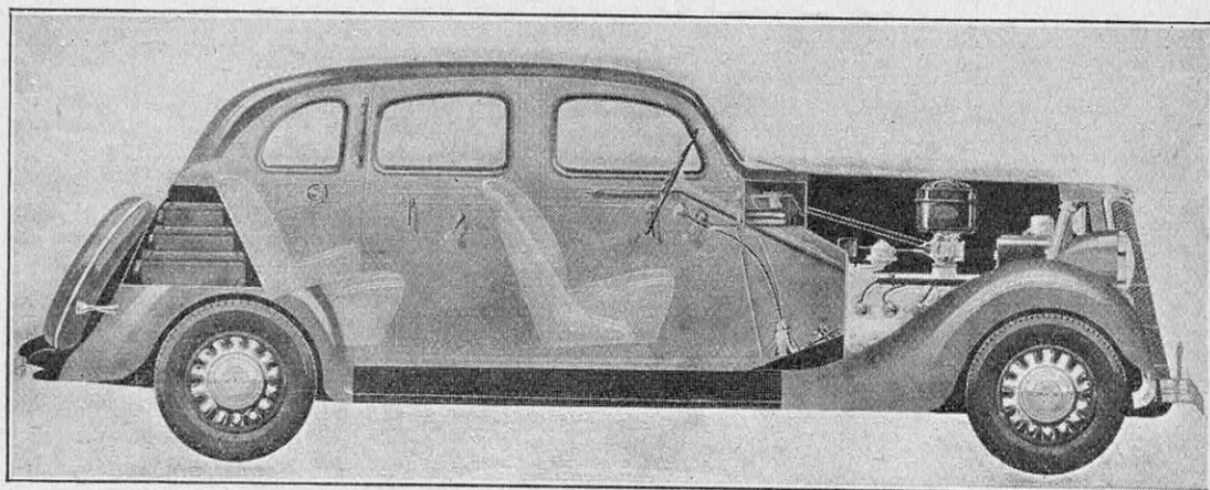
FIG. 5. — VOICI UN EXEMPLE DE « CENTRAGE AMÉRICAIN » QUI PERMET, AVEC UNE EXCELLENTE TENUE DE ROUTE, D'OBTENIR LE MAXIMUM DE CONFORT POUR LES PASSAGERS. Sur cette voiture vue en coupe (Ford V 8), on remarque la disposition des passagers entre les essieux, le moteur étant reporté le plus en avant possible et l'arrière pouvant loger les malles et la roue de secours. Grâce à cette heureuse répartition des masses, l'avant et l'arrière de la voiture sont à peu près également chargés, d'où une excellente tenue de route, en même temps qu'un plus grand confort de la suspension.
