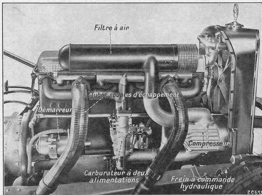
FIG. 1. — VOICI UN MOTEUR TRÈS PUISSANT (5 LITRES DE CYLINDRÉE) DESTINÉ A ÉQUIPER DES VOITURES DE GRAND SPORT CAPABLES DE DÉPASSER 150 KILOMÈTRES A L'HEURE. Aux hautes allures, l'alimentation de ce moteur se fait par l'intermédiaire d'un compresseur mis en mouvement à partir d'une certaine vitesse. On remarquera, en outre, la disposition des soupapes en tête et le filtre à air de très grand volume. Une voiture de grand sport munie d'un tel moteur (Mercedes-Benz) est capable d'atteindre aisément une vitesse de 180 kilomètres à l'heure.
