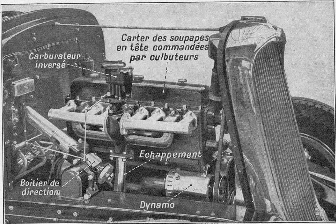
FIG. 4. — CE MOTEUR A TRÈS HAUT RENDEMENT EST DESTINÉ A ÉQUIPER DES VOITURES PUISSANTES, CAPABLES DE SOUTENIR DE GRANDES VITESSES
