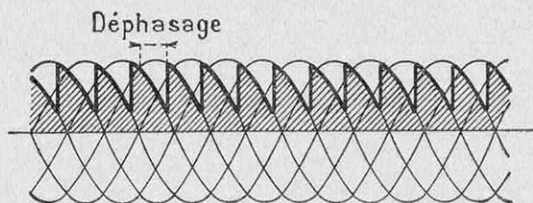
FIG. 7. — COURANT CONTINU LIVRÉ PAR UN REDRESSEUR HEXAPHASÉ COMMANDÉ PAR LE DÉPHASAGE DE LA TENSION-GRILLE
