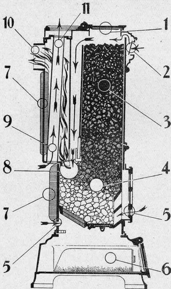
COUPE D'UN POËLE « CINEY »
