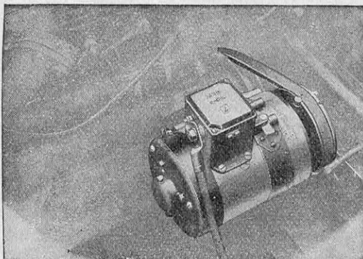
LE DYNAMOTEUR A COMMANDE PAR COURROIE SUR CHASSIS BERLIET « DAUPHINE »
