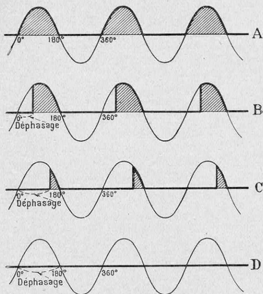
FIG. 6. — COMMENT LE DÉPHASAGE DE LA TENSION-GRILLE PERMET DE RÉGLER LE DÉBIT D'UN REDRESSEUR
