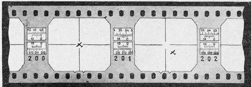
FIG. 8. — FRAGMENT DE FILM PRIS PAR UN « CINÉTHÉODOLITE »
