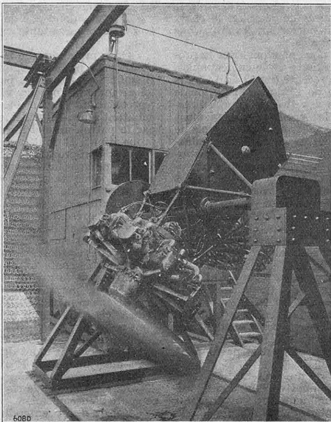
MOTEUR D'AVIATION BRISTOL TYPE « PÉGASUS » INSTALLÉ SUR LE BANC D'ESSAIS SPÉCIAL POUR LES ÉPREUVES DE FONCTIONNEMENT SOUS INCLINAISON VARIABLE
