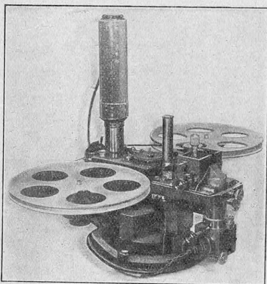
FIG. 2. — APPAREIL ENREGISTREUR SÉLÉNOPHON UTILISÉ EN PARTICULIER A « RADIO-TOULOUSE » ET A BORD DU CAR DE RADIO-REPORTAGE
