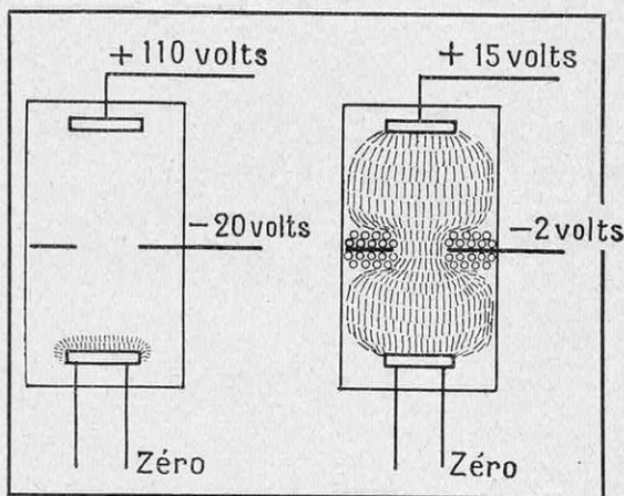
FIG. 5. — PRINCIPE DE LA COMMANDE DE LA DÉCHARGE DANS UN GAZ RARÉFIÉ PAR UNE GRILLE D'ANODE
