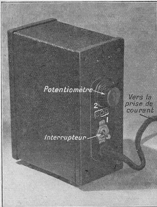
FIG. 3. — L'AMPLIFICATEUR PORTATIF, INTERMÉDIAIRE INÉVITABLE ENTRE LE VIBREUR ET LE MICROPHONE
