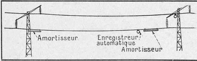
FIG. 5. — COMMENT SONT DISPOSÉS, EN PRATIQUE, LES AMORTISSEURS ET L'ENREGISTREUR AUTOMATIQUE DE VIBRATIONS SUR UN TRONÇON DE LIGNE
