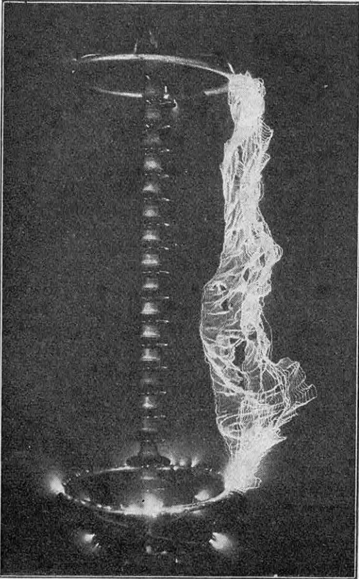
FIG. 8. — UNE FORME CURIEUSE D'ÉTINCELLE D'AMORÇAGE D'UN COURT-CIRCUIT DE 1.000.000 DE VOLTS, CONTOURNANT UNE CHAÎNE DE 18 ÉLÉMENTS ISOLATEURS
