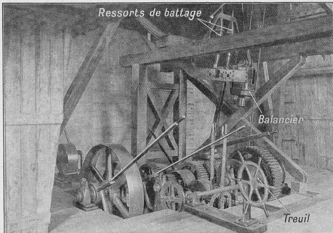
FIG. 3. — VOICI UNE INSTALLATION MODERNE POUR LE FORAGE DES PUIITS PROFONDS
