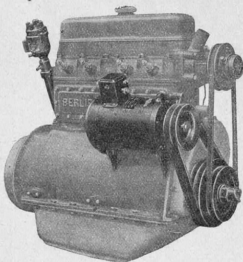
LE DYNAMOTEUR A COMMANDE PAR COURROIE MONTÉ SUR UN MOTEUR DE 5 A 6 CH
