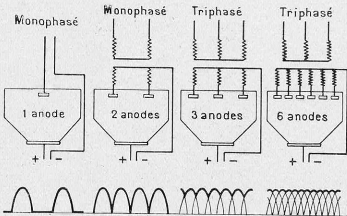
FIG. 4. — COMMENT S'EFFECTUE, EN PRINCIPE, LE REDRESSEMENT DU COURANT ALTERNATIF, MONOPHASÉ OU TRIPHASÉ, PAR LES VALVES A GAZ IONISÉ
