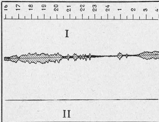
FIG. 6. — DIAGRAMME DE VIBRATIONS MÉCANIQUES ENREGISTRÉES AUTOMATIQUÉMENT SUR LE CÂBLE ENTRE DEUX PYLONES
