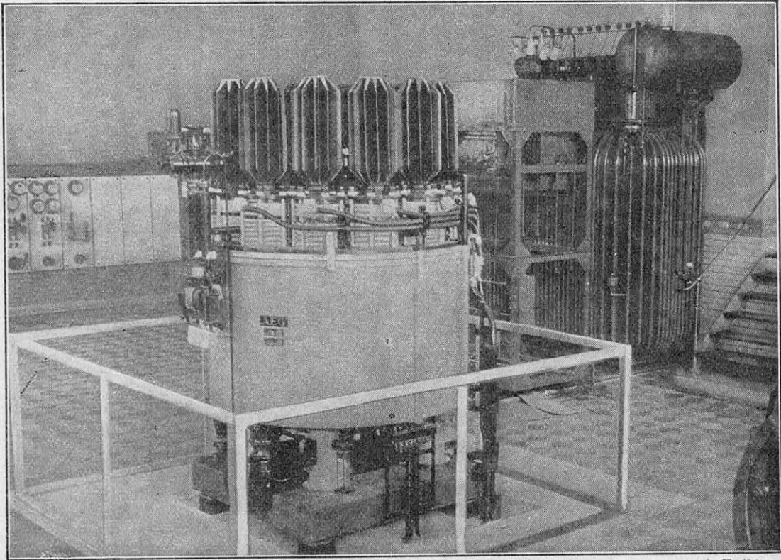
FIG. 8. — REDRESSEUR A VAPEUR DE MERCURE A CUVE MÉTALLIQUE INSTALLÉ A LA CENTRALE ÉLECTRIQUE DE NORDKÖPING (SUÈDE)
