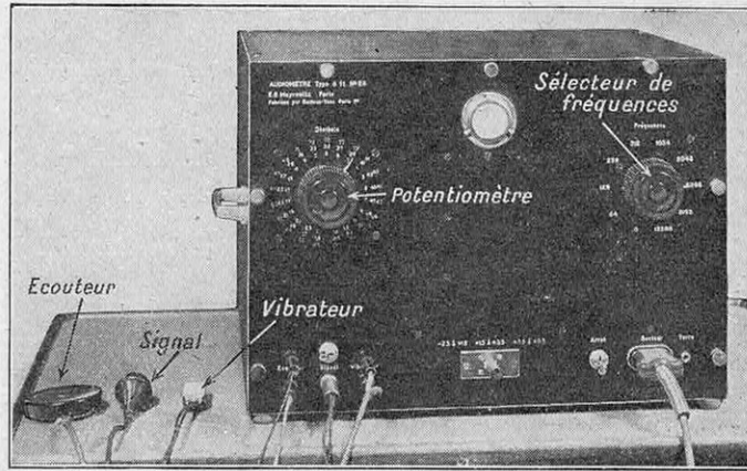
FIG. 4. — L'AUDIOMÈTRE AU MOYEN DUQUEL SONT ÉTABLIS EXPÉRIMENTALEMENT, POINT PAR POINT, LES « AUDIOPROGRAMMES » RELATIFS A CHAQUE SUJET SOURD-MUET. Le problème à résoudre est de mesurer exactement toute une série d'intensités sonores pour chaque fréquence musicale. Sans entrer dans le montage de l'appareil, nous voyons que l'échelle des intensités dépend d'un potentiomètre de précision et la gamme des fréquences d'un sélecteur spécial. A gauche : l'écouteur et le vibreur (appareils de l'audition) et le signal que le sujet déclenche chaque fois qu'il parvient au « seuil » de la sensation auditive. (Voir schéma suivant.)
