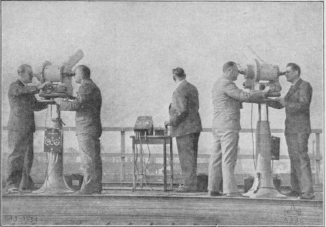
FIG. 9. — PHOTOGRAPHIE MONTRANT DEUX STATIONS DE « CINÉTHÉODOLITES » COOPÉRANT POUR SUIVRE LES ÉVOLUTIONS RAPIDES D'UN AVION DANS L'ESPACE
