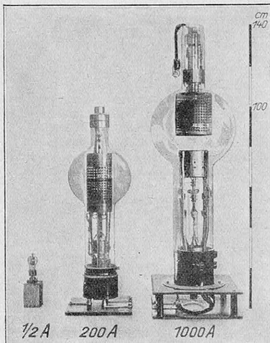
FIG. 2. — TYPES DE REDRESSEURS A VAPEUR DE MERCURE ET A CATHODE INCANDESCENTE MUNIS DE LA COMMANDE PAR GRILLE
