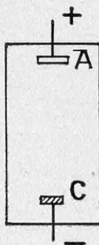
FIG. 1. — DISPOSITION SCHÉMATIQUE D'UN TUBE A DÉCHARGE DANS LES GAZ
