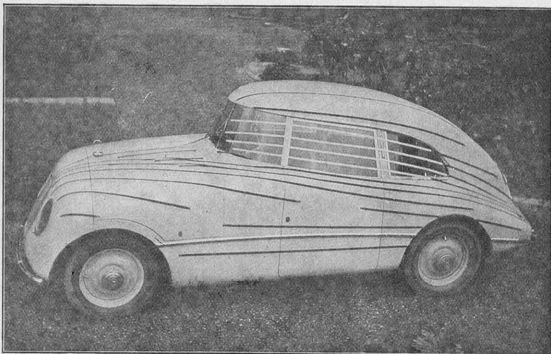
FIG. 1. — COMMENT SE RÉPARTISSENT LES FILETS D'AIR AUTOUR D'UNE CARROSSERIE AÉRODYNAMIQUE CONÇUE PAR L'INGÉNIEUR JARAY
