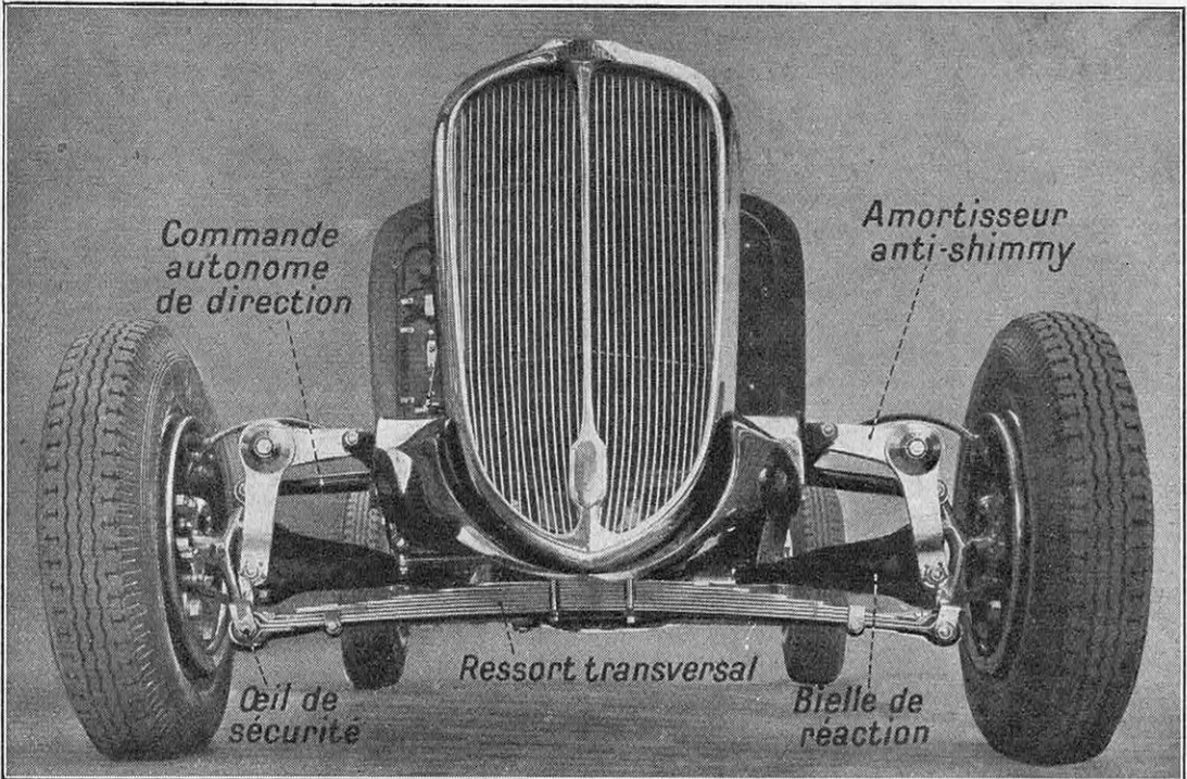
FIG. 3. — VOICI UN EXEMPLE DE SUSPENSION PAR ROUES AVANT INDÉPENDANTES SUR UNE VOITURE RAPIDE ET DE GRANDE PUISSANCE (DELAHAYE 18 CH)
