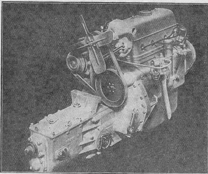
FIG. 1. — LE MOTEUR DE LA « 7 CH CITROËN » FAIT UNE LARGE PART AUX ALLIAGES LÉGERS. LES PIÈCES EN ALLIAGES D'ALUMINIUM (BOÎTE DE VITESSE, CARTER DE VOLANT, POMPE À EAU, ETC.) SE DÉTACHENT EN CLAIR AU PREMIER PLAN SUR L'ENSEMBLE
