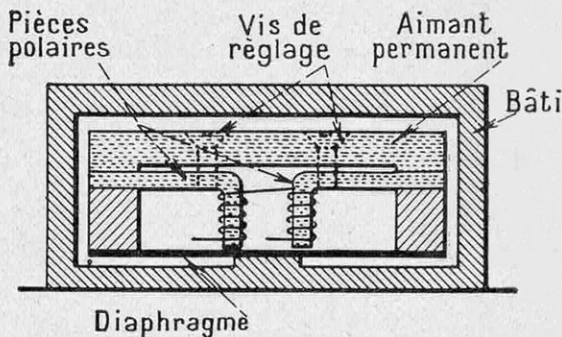
FIG. 2. — SCHÉMA DE FONCTIONNEMENT DU VIBRATEUR « LIEBER »
