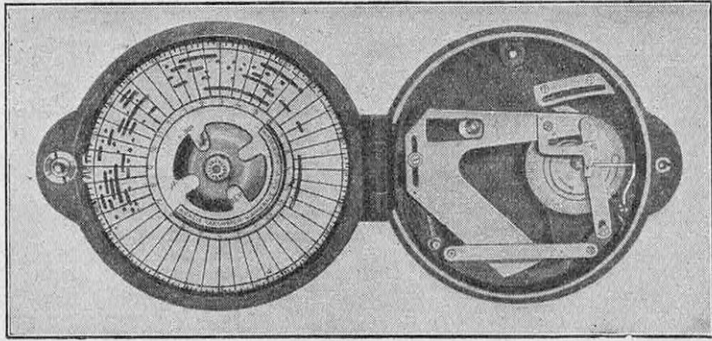
FIG. 4. — APPAREIL ENREGISTREUR AUTOMATIQUE DES VIBRATIONS MÉCANIQUES D'UN CONDUCTEUR DE LIGNE
