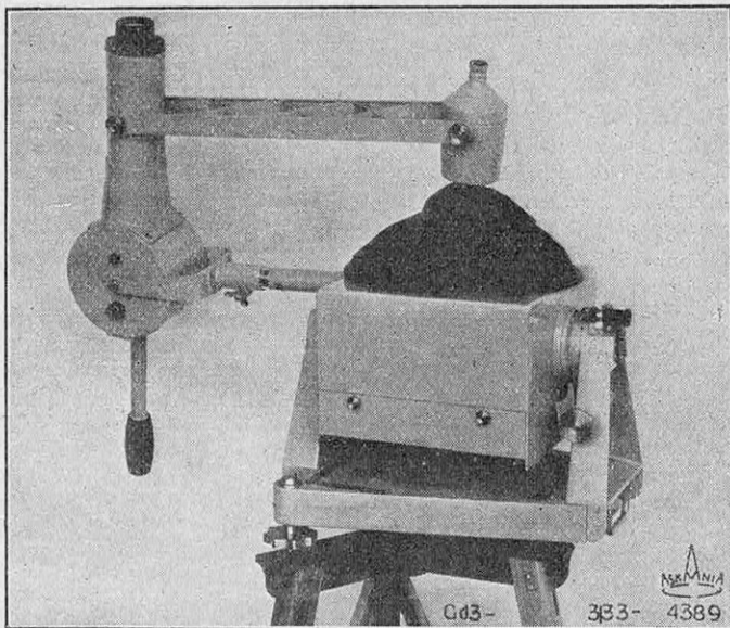
FIG. 4. — ENSEMBLE DE L'APPAREIL PHOTOGRAMMÉTRIQUE ÉTABLI D'APRÈS LE SCHÉMA DE LA FIGURE 3
