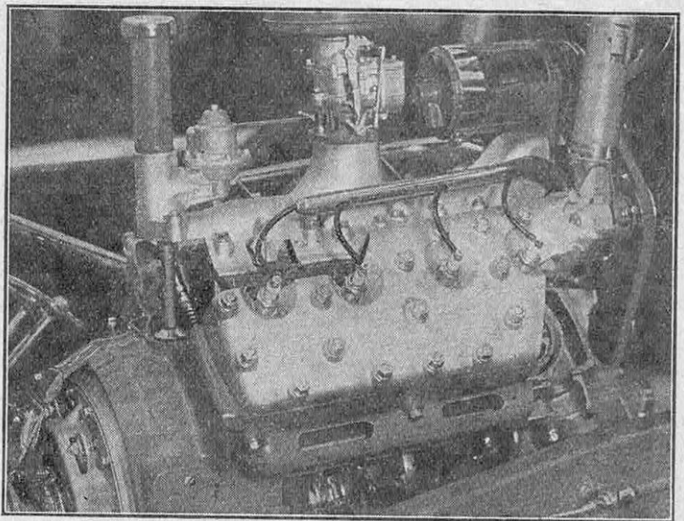
FIG. 2. — VOICI UNE DES DEUX CULASSES EN ALUMINIUM DE LA « FORD V 8-40 » QUI APPARAÎT ICI PLUS CLAIRE QUE LES AUTRES PIÈCES EN FONTE OU EN TOLE
