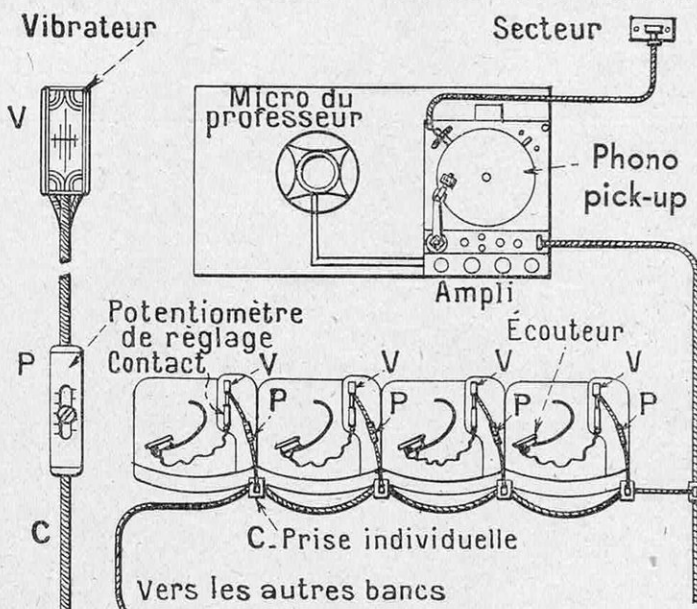
FIG. 7. - SCHÉMA D'INSTALLATION DE LA CLASSE D'ÉDUCATION POUR SOURDS-MUETS PAR AUDITION AMPLIFIÉE
