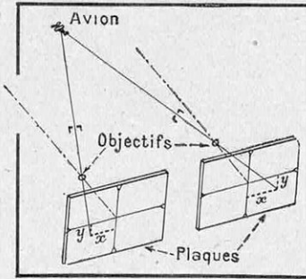
FIG. 6. — COMMENT ON PEUT UTILISER DEUX PLAQUES PHOTOGRAPHIQUES POUR MESURER LA VITESSE D'UN AVION
