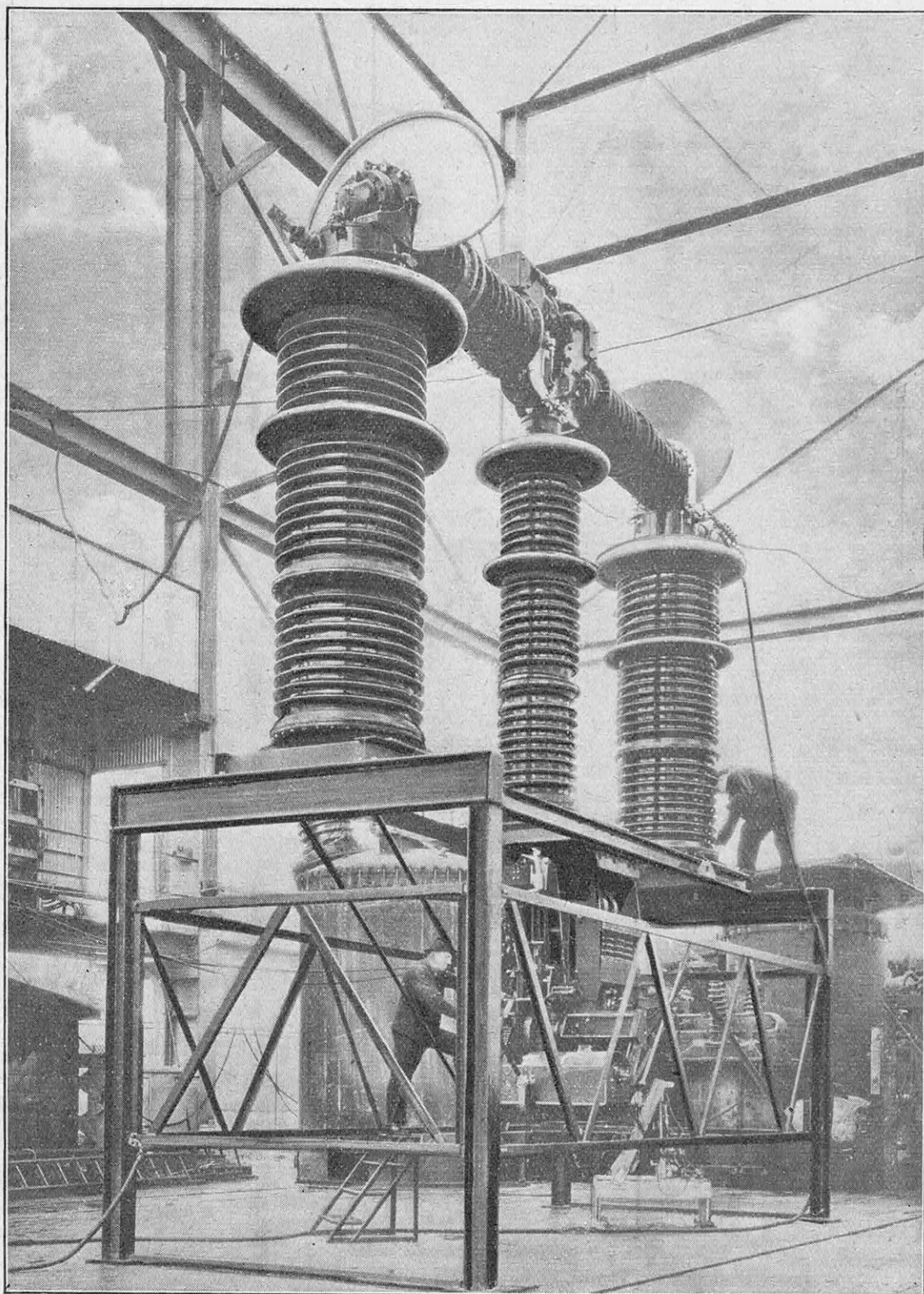
FIG. 1. — VOICI L'UN DES NOUVEAUX TYPES D'INTERRUPTEURS A HUILE LES PLUS IMPRESSIONNANTS, POUVANT COUPER UN COURANT DE 5.000 AMPÈRES SOUS UNE TENSION DE 287.000 VOLTS, SOIT 1.435.000 KILOWATTS
