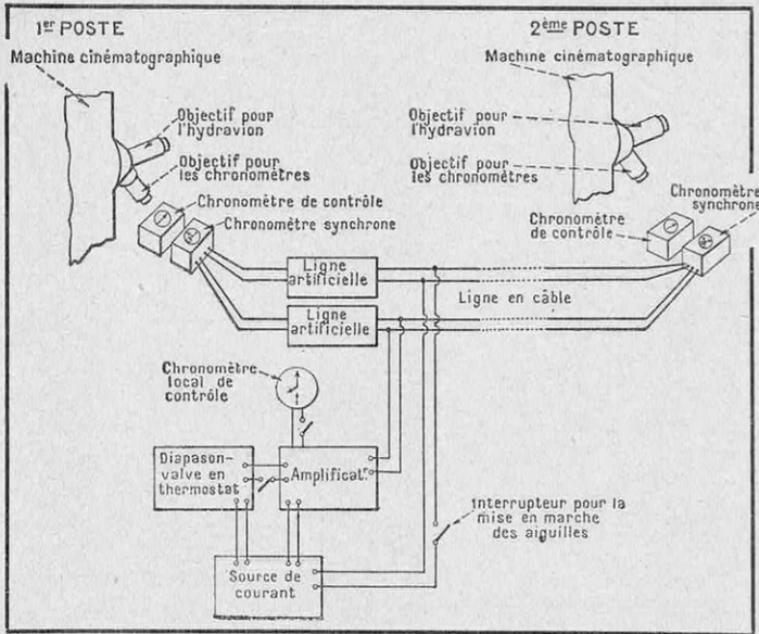
FIG. 1. — SCHEMA D'INSTALLATION DU DISPOSITIF DE CHRONOMETRAGE DES AVIONS DE GRANDE VITESSE SUR BASE, UTILISÉ PAR L'AÉRONAUTIQUE ITALIENNE
