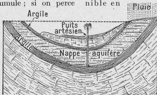
FIG. 2. — SCHÉMA DU PRINCIPE DE FONCTIONNEMENT D'UN PUIT ARTÉSIEN CLASSIQUE
