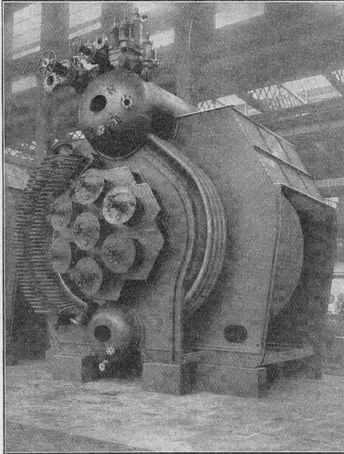
FIG. 3. — CHAUDIÈRE TUBULAIRE DU TYPE « JOHNSON » A HAUTE PRESSION, UTILISÉE A BORD DE CERTAINS PAQUEBOTS ANGLAIS EN SERVICE SUR L'AMÉRIQUE DU SUD Dans ces chaudières, la chambre de combustion est complètement entourée de tubes, ce qui réduit au minimum la surface des parois recouvertes de produits réfractaires, et assure une proportion beaucoup plus considérable que dans les chaudières à tubes d'eau ordinaires, des surfaces exposées au rayonnement direct du foyer. Le timbre des chaudières en question a atteint, à bord de l'Asturias, 31 kg 500 et la température maximum est de 400 degrés. Le taux de vaporisation est de l'ordre de 90 kilogrammes de vapeur par mètre carré de surface de chauffe et par heure.
