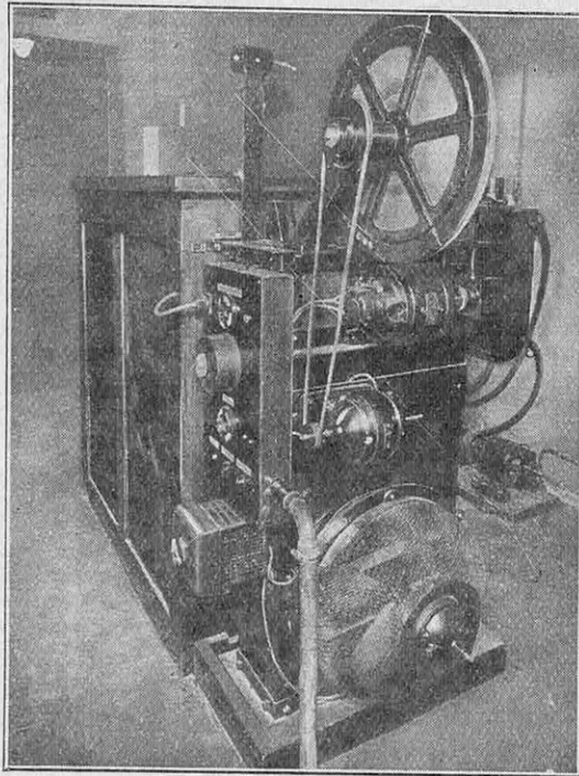
FIG. 4. — MACHINE AUTOMATIQUE A DÉVELOPPER LES FILMS, SYSTÈME SÉLÉNOPHON
