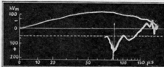
FIG. 9. — LA COURBE DES « SURTENSIONS » (EN ORDONNÉE) SE DÉVELOPPANT DANS UN COURT-CIRCUIT AU COURS DE L'ÉCLATEMENT DE L'ÉTINCELLE
