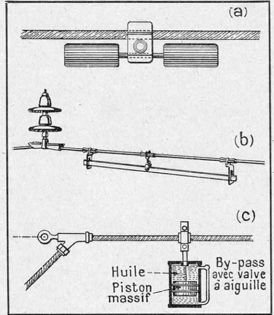
FIG. 7. — LES DIFFÉRENTS TYPES D'AMORTISSEURS ESSAYÉS EN VUE DE NEUTRALISER LES VIBRATIONS MÉCANIQUES DES CÂBLES
