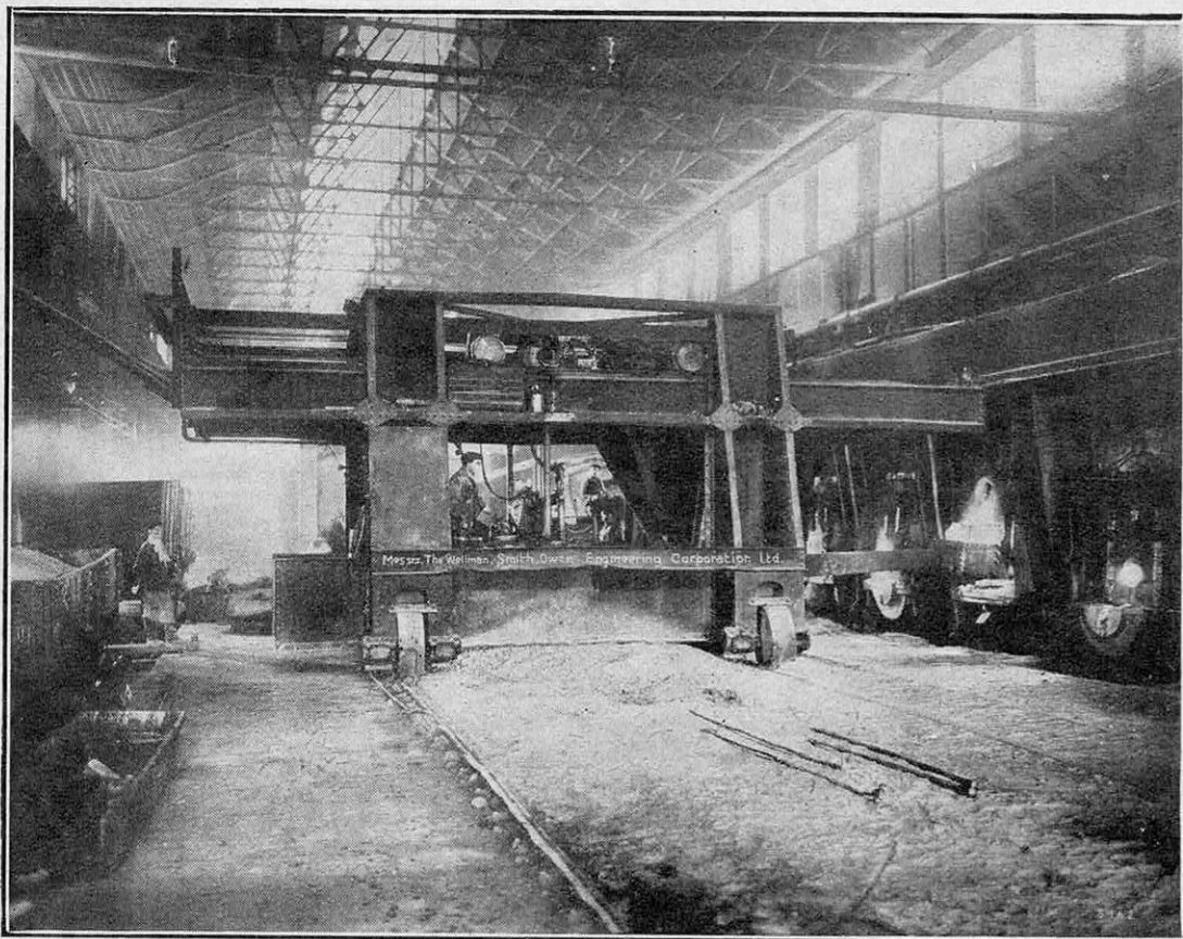
CHARGEUSE D'ACIÉRIE TYPE HAUT, SYSTÈME WELLMAN, MONTÉE SUR CHARIOT ET PERMETTANT LE TRANSPORT RAPIDE DES LINGOTS INCANDESCENTS
