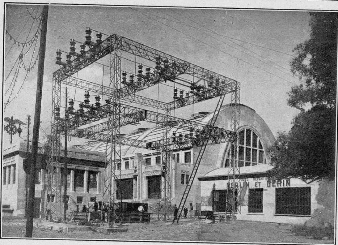
FIG. 16. — POSTE DE TRANSFORMATION EXTÉRIEUR, CONSTRUIT DANS L'ENCEINTE DE L'EXPOSITION DE GRENOBLE PAR LES ÉTABLISSEMENTS MERLIN ET GERIN
