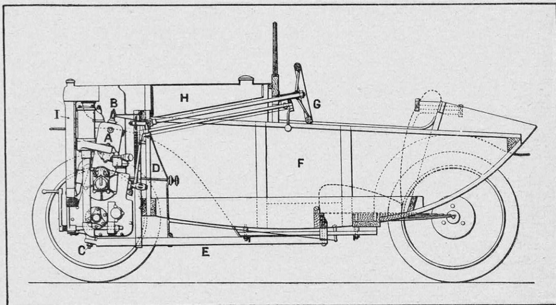
FIG. 7. — DÉTAILS DU MÉCANISME ET DE L'INSTALLATION DE LA CARROSSERIE DU VÉHICULE MONOPLACE DÉCRIT AU COURS DE LA CAUSERIE
