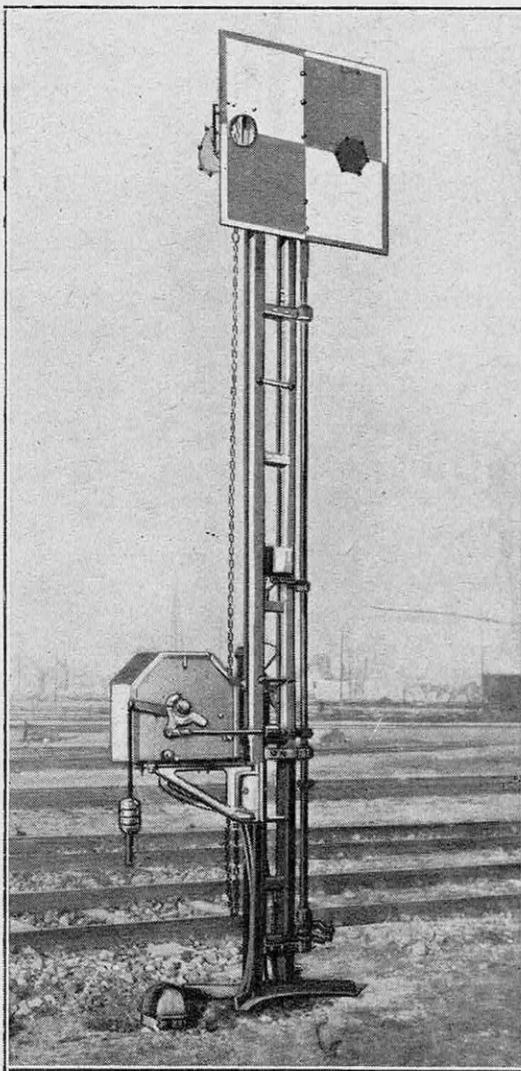
FIG. 2. - SIGNAL COMMANDÉ PAR UN MOTEUR ÉLECTRIQUE A DÉCLENCHEMENT
