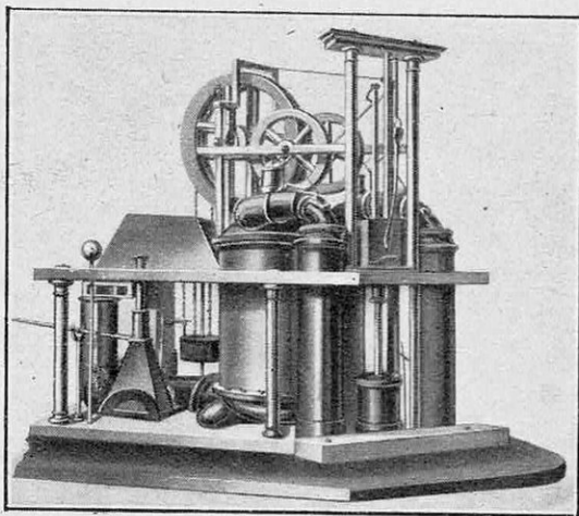
ENSEMBLE DU MOTEUR NIEPCE
