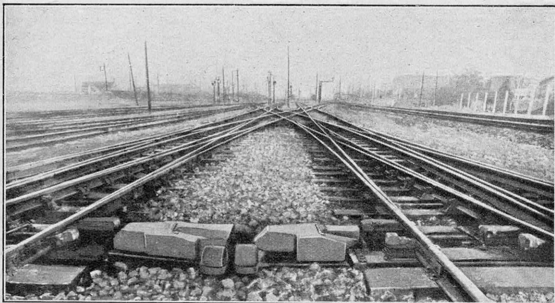
FIG. 1. — MOTEURS ÉLECTRIQUES DE MANŒUVRE D'AIGUILLES COMMANDÉS A DISTANCE
