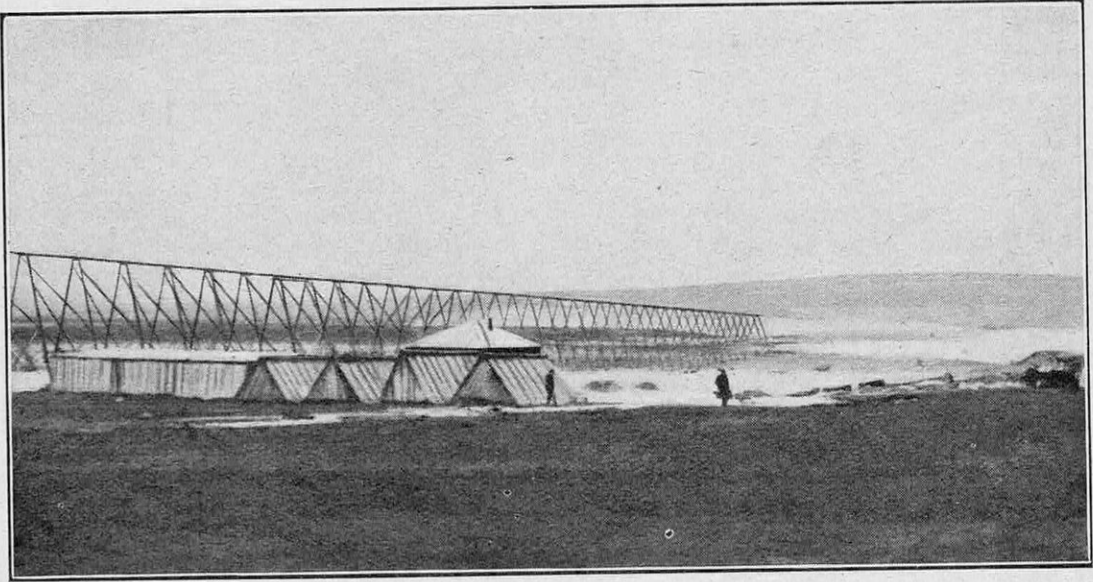
CANAL D'AMENÉE DES « TAILINGS » A LA MINE WEMMER (TRANSVAAL)
