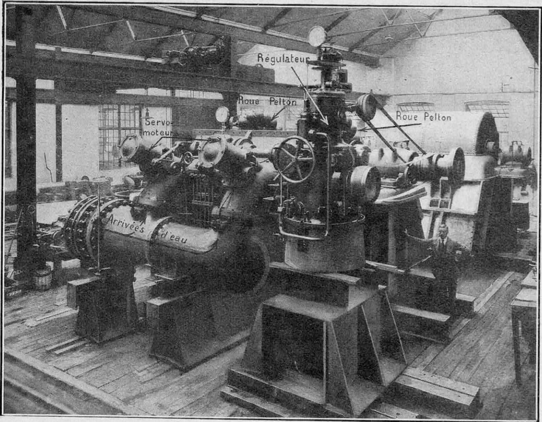
FIG. 9. — USINE DE NISHIKADOHARA (JAPON). — Ateliers de Kristinehamn (Suède)
