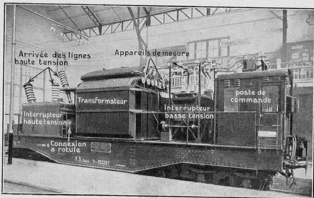
FIG. 17. — SOUS-STATION MOBILE DE TRANSFORMATION DES CHEMINS DE FER DE L'ÉTAT ITALIEN CAPABLE DE CIRCULER SUR LES VOIES FERRÉES POUR REMPLACER UNE SOUS-STATION FIXE ARRÊTÉE ACCIDENTELLEMENT
