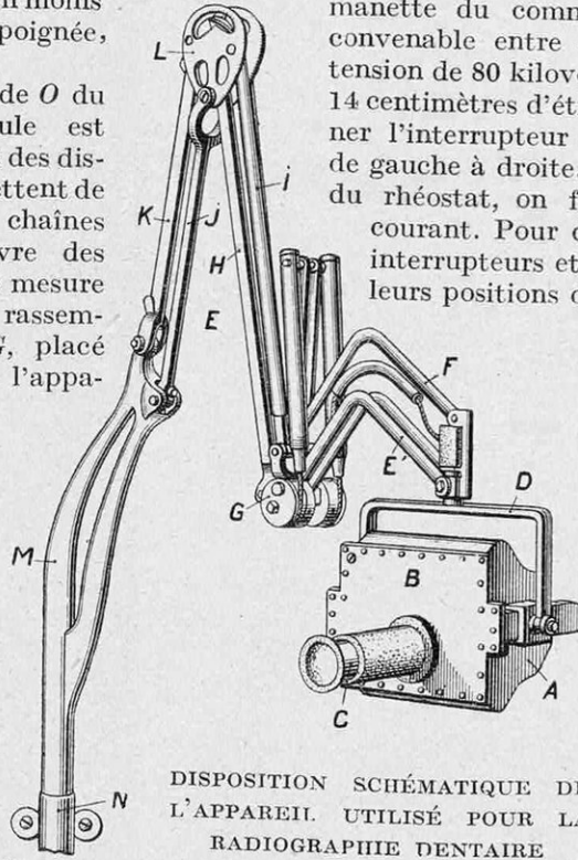
DISPOSITION SCHÉMATIQUE DE L'APPAREIL UTILISÉ POUR LA RADIOGRAPHIE DENTAIRE A, boîte métallique contenant le transformateur et l'ampoule ; B, couvercle ; C, tube localisant le faisceau de rayons X ; D, étrier de support ; E E' F H I J K, arbres ou bras articulés formant support ; G L, articulations ; M, ressort compensateur équilibrant la suspension ; N, partie se fixant au mur.
