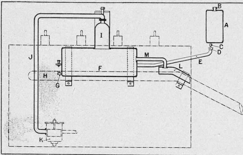
SCHÉMA D'INSTALLATION DU DISPOSITIF SAINT-PÉ SUR UN MOTEUR
