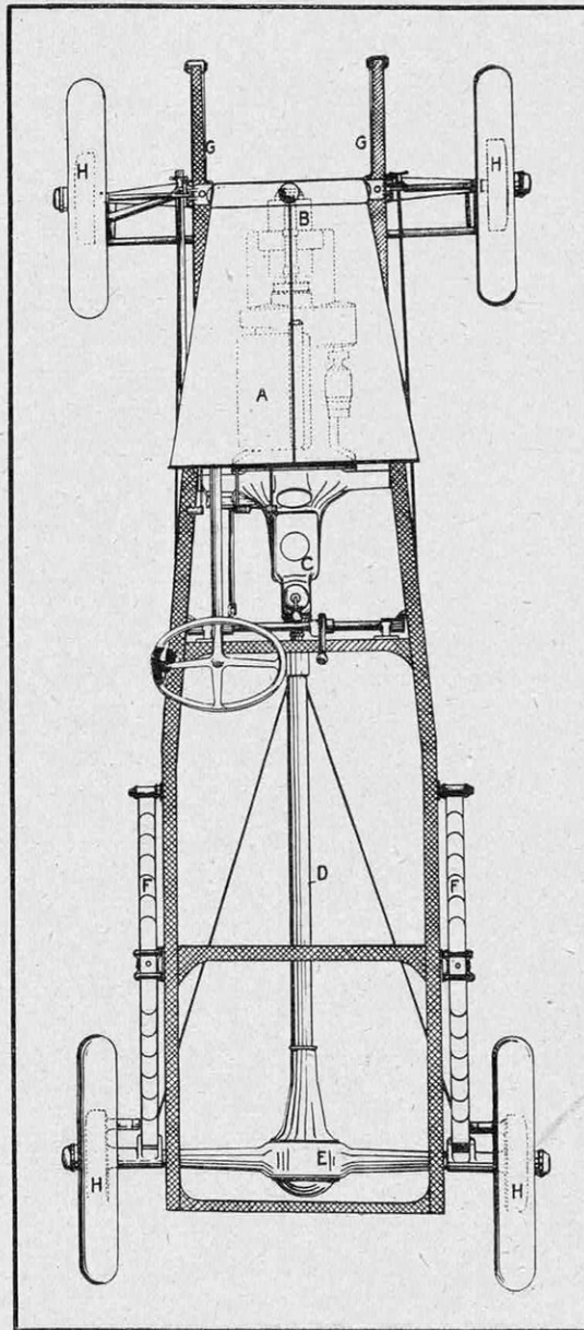
FIG. 2. — PLAN D'UN CHASSIS 8 CV, DE FACTURE TRÈS MODERNE
