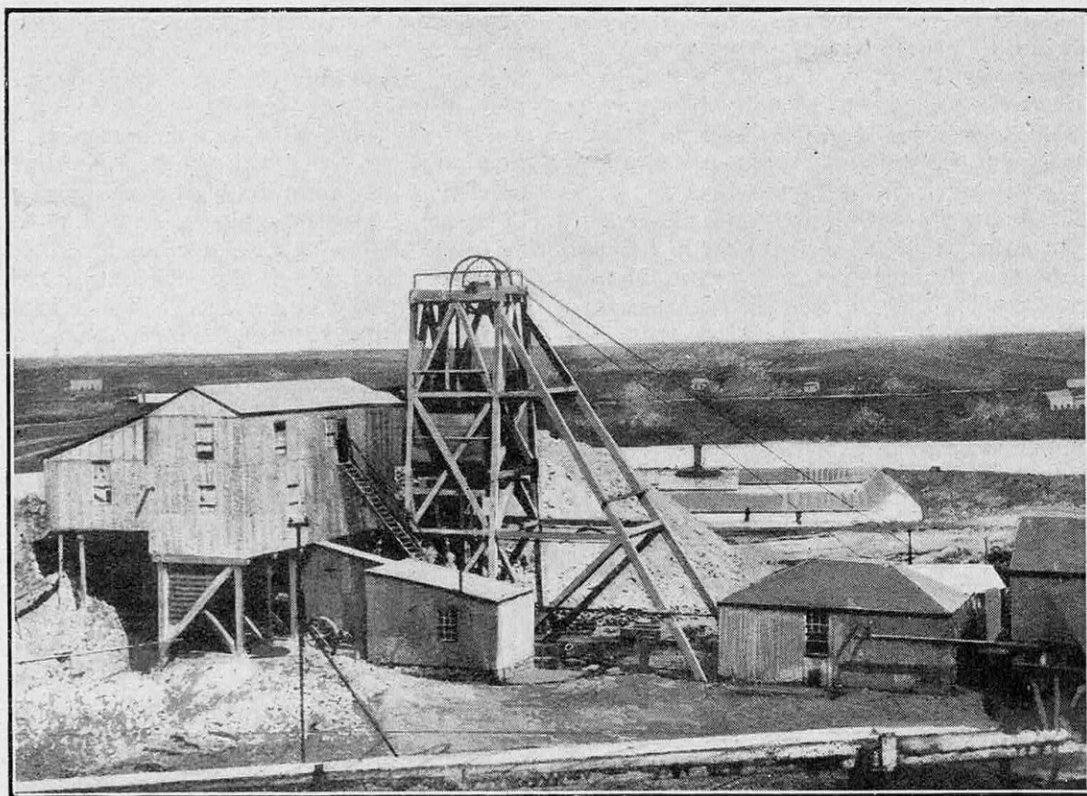
VUE D'ENSEMBLE DES INSTALLATIONS EXTÉRIEURES DE LA « CHIMES »
