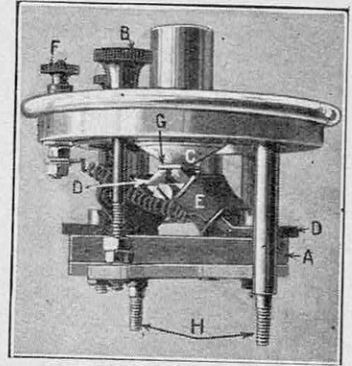
FIG. 2. — DISPOSITIF INTÉRIEUR DU HAUT-PARLEUR
