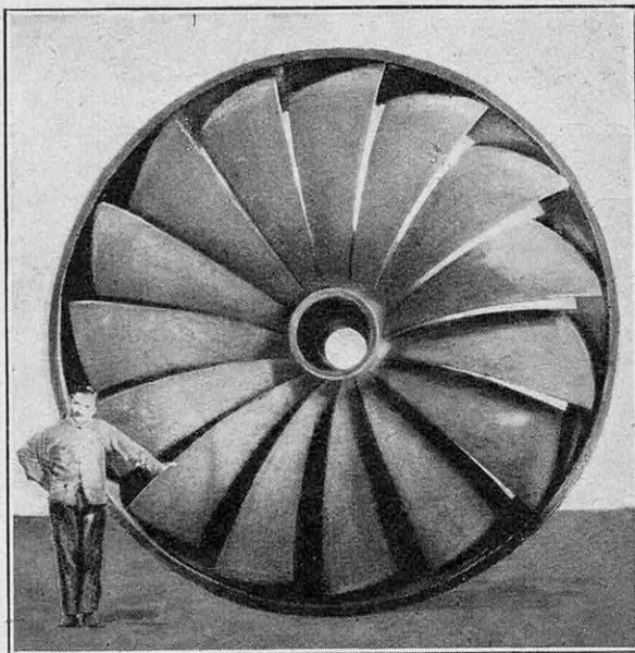
FIG. 6. — ROUE MOBILE D'UNE TURBINE AMÉRICAINNE FRANCIS (Neyret-Beylier constructeur.)
