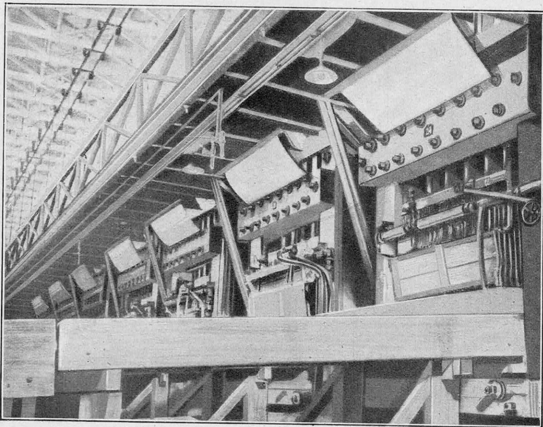
BATTERIE DE PILONS MÉCANIQUES DE LA « GELDENHUIS ESTATE »
