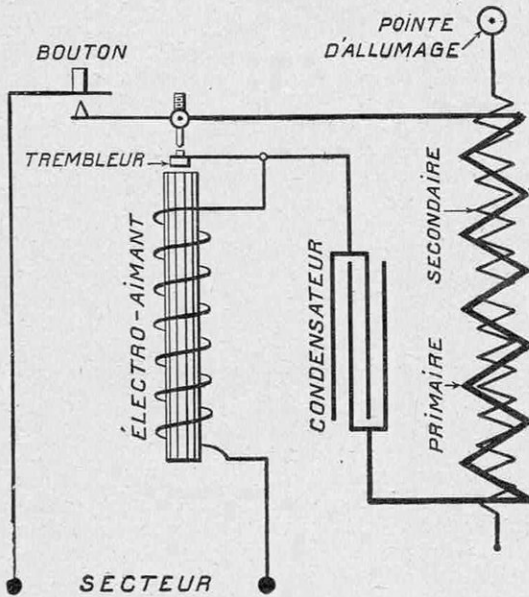
SCHÉMA DE MONTAGE DE L'ALLUMEUR ÉLECTRIQUE A HAUTE FRÉQUENCE
