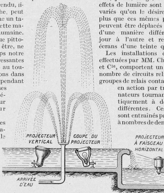
FIG. 1. — COUPE PAR UN BASSIN DES FONTAINES LUMINEUSES DE L'EXPOSITION DE GRENOBLE
