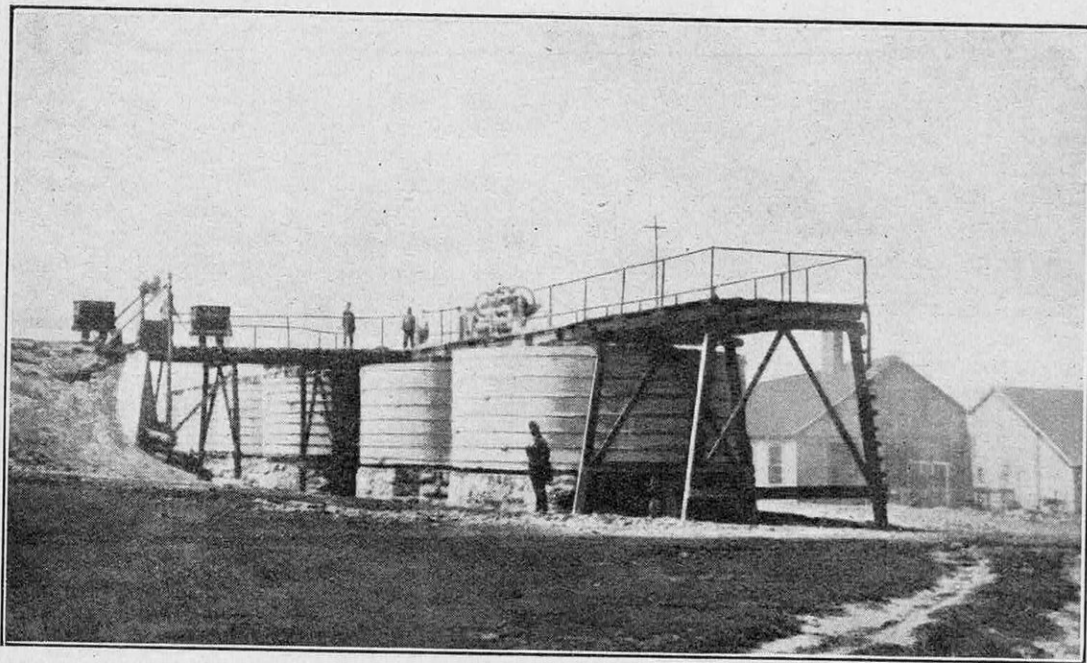
GRUPE DE CUVES DE CYANURATION DE LA « WEMMER »
