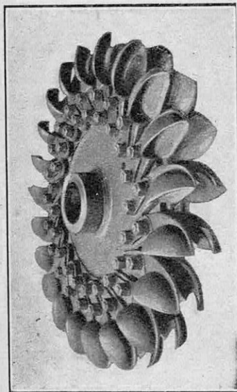
FIG. 5. — LA ROUE PELTON (Neyret-Beylier constructeur.)
