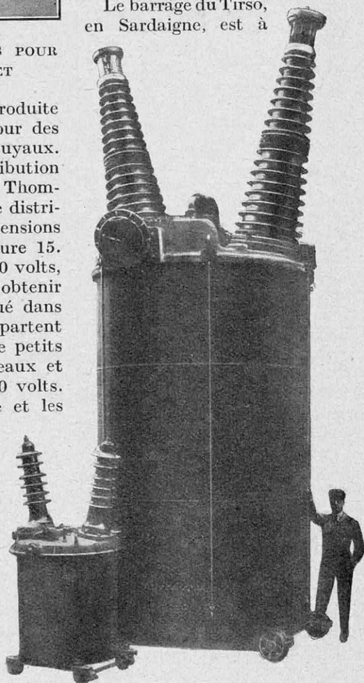
FIG. 19. — DISJONCTEUR DE 220.000 VOLTS. A GAUCHE, DISJONCTEUR DE 75.000 VOLTS (Ateliers de constructions électriques de Delle.)
