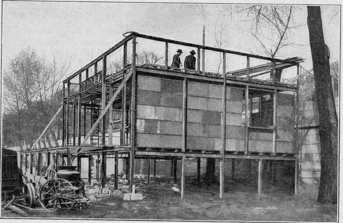
LE PAVILLON DECOURT PENDANT LA CONSTRUCTION
