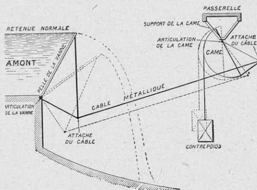
FIG. 12. — SCHEMA DE LA VANNE AUTOMATIQUE JOYA-BATICLE
