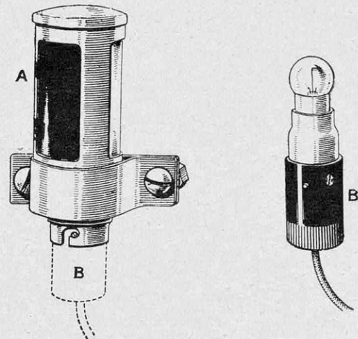
UNE LANTERNE ARRIÈRE ÉLECTRIQUE AVEC DOUILLE AMOVIBLE
