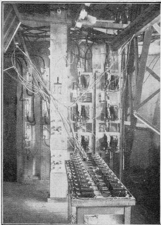
LES VINGT-QUATRE RELAIS QUI PERMETTENT DE MODIFIER LES MOTIFS LUMINEUX
