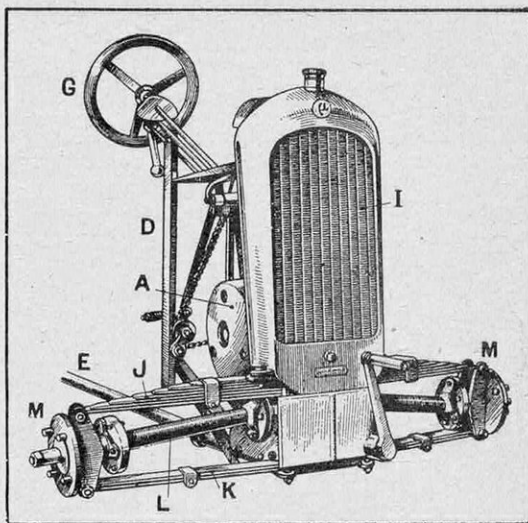
FIG. 6. — UN INTÉRESSANT GROUPE RÉUNISSANT MOTEUR ET TRANSMISSION, CELLE-CI ATTAQUANT DIRECTEMENT LES ROUES AVANT A, moteur ; D, cadre soutenant le moteur ; E, tube entretoisé conjugué avec le cadre D ; G, volant de direction ; I, radiateur à grande surface ; J et K, ressorts transversaux, aux extrémités desquels sont montés les plateaux supportant les moyeux des roues ; L, arbres latéraux d'entraînement des roues, garnis de joints souples sans graissage à chacune de leurs extrémités ; M, supports sur lesquels sont montées les roues amovibles.
