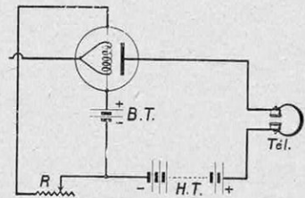
FIG. 5. — MONTAGE SUSCEPTIBLE DE DÉSAIMANTER LES AIMANTS D'UN HAUT-PARLEUR OU D'UN CASQUE
