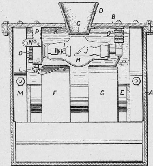
VUE EN COUPE DE LA BOÎTE
