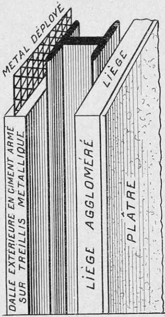
DESSIN MONTRANT LA CONSTITUTION D'UN MUR DU PAVILLON DECOURT
