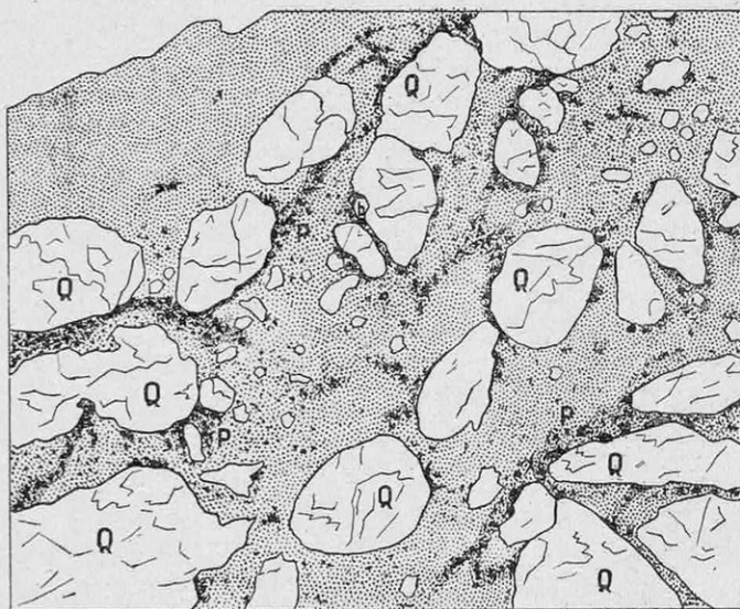
STRUCTURE DU CONGLOMÉRAT AURIFÈRE DU TRANSVAAL Les galets de quartz blanc Q sont stériles. L'or est renfermé avec de la pyrite de fer P dans le ciment gris qui les entoure.
