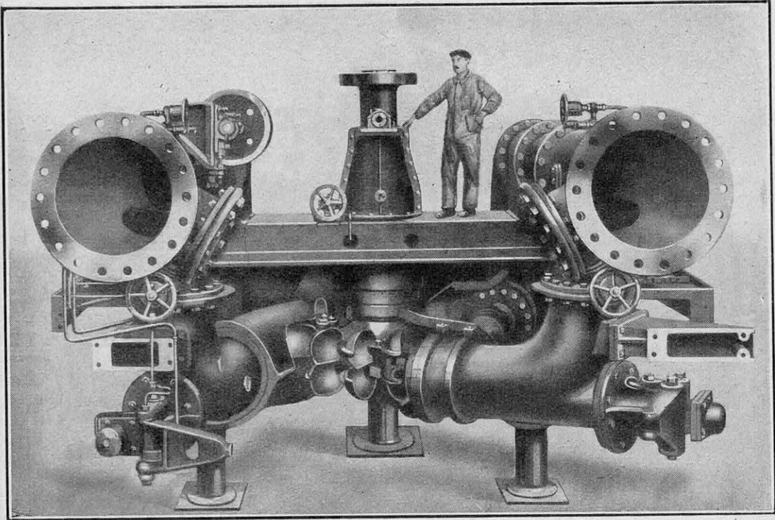
FIG. 11. — TURBINE TANGENTIELLE DE 15.000 C. V. A AXE VERTICALE, A LA CENTRALE DE BIAS-CHINA, A BODIO (SUISSE) (TURBINE ESCHER WYSS ET C ie )
