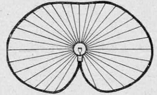
FIG. 3. — COURBE POLAIRE D'UNE LAMPE NUE
