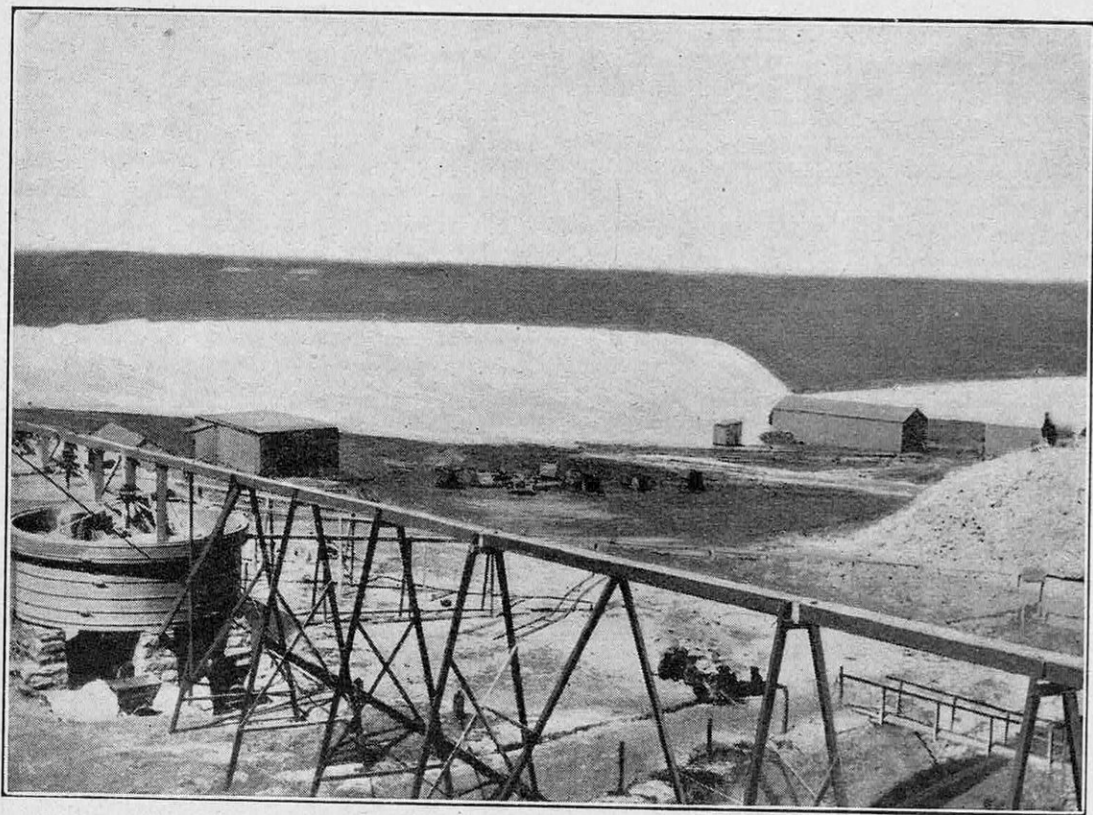
VUE GÉNÉRALE DE L'INSTALLATION DE LA « CHIMES » (TRANSVAAL)
