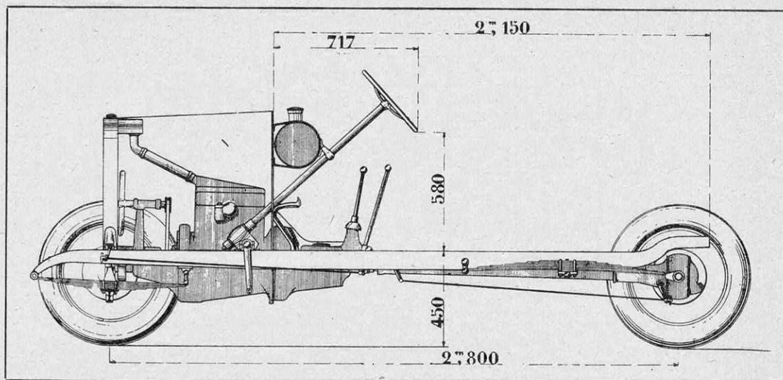
FIG. 3. — UN CHASSIS 8 CV DESTINÉ A RECEVOIR DES CARROSSERIES A QUATRE PLACES
