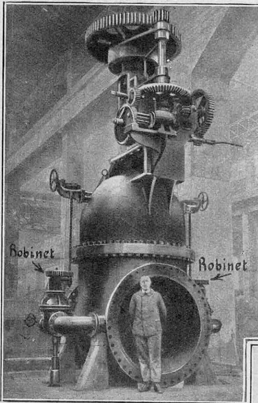
FIG. 13. — ROBINET-VANNE DE L'USINE DU HOURAT, DE LA COMPAGNIE DES CHEMINS DE FER DU MIDI (Neyret-Beylier et Piccard-Pictet, constructeurs.)
