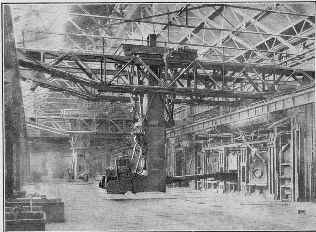
PONT ROULANT CHARGEUR POUR FOUR MARTIN (PUISSANCE : 2,500 KILOS)
