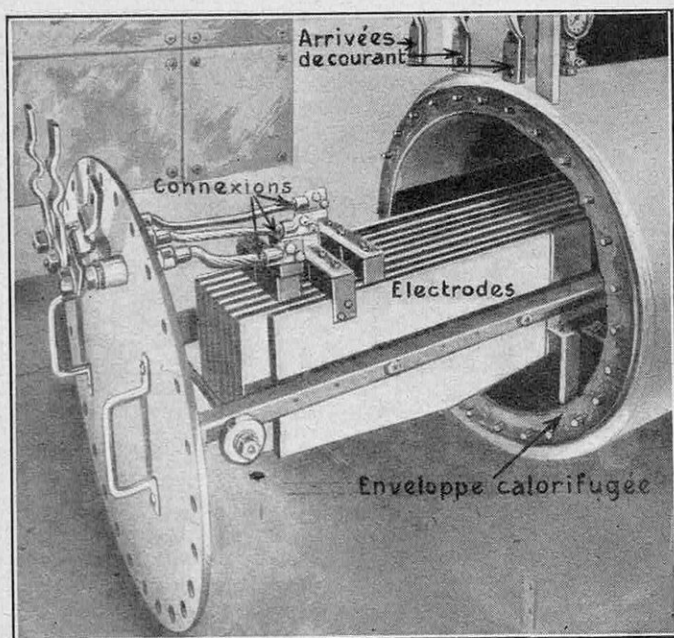
FIG. 18. — DÉTAILS D'UN BLOC ÉLECTRODES POUR CHAUDIÈRES ÉLECTRIQUES BERGEON-FREDET
