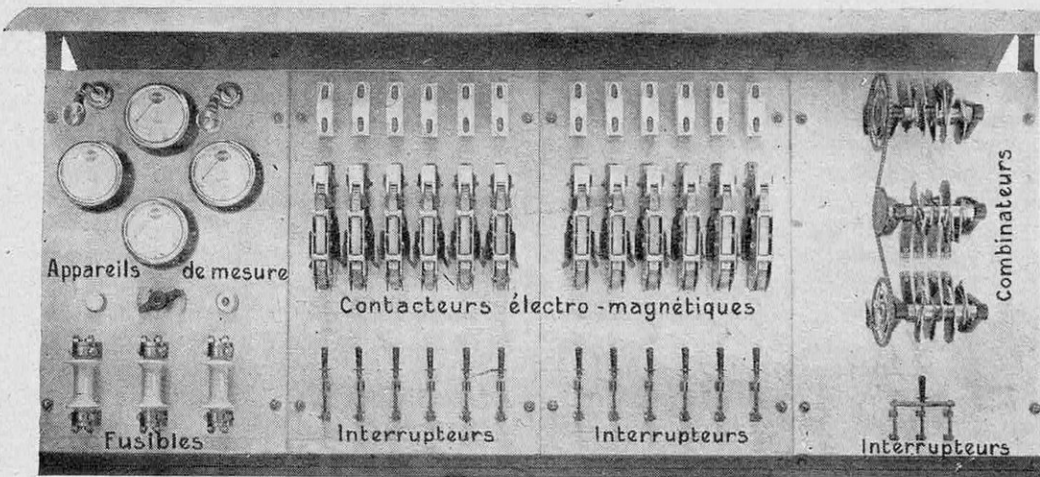
FIG. 4. — JEU D'ORGUE AUTOMATIQUE POUR LE CONTROLE DES CIRCUITS ÉLECTRIQUES DES PROJECTEURS DES FONTAINES LUMINEUSES
