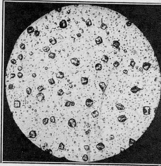
FIG. 5. — LE RÉSIDU SALIN LAISSÉ SUR UNE LAME DE VERRE PAR L'ÉVAPORATION DE QUELQUES GOUTTES D'EAU DE MER
