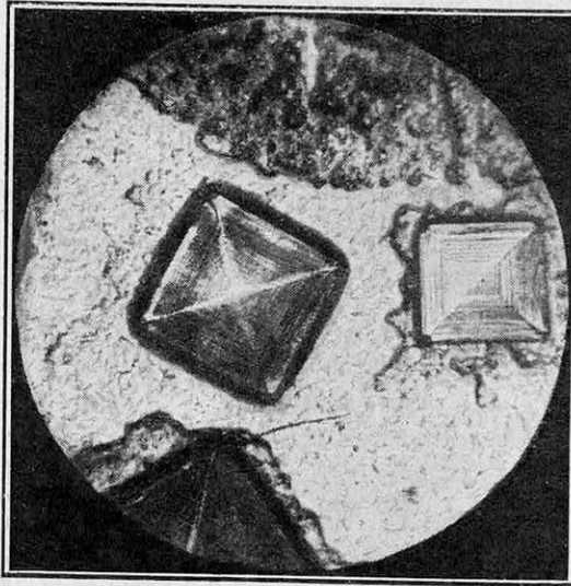
FIG. 6. — CRISTAUX DE SEL MARIN, GROUPÉS EN PYRAMIDES QUADRANGULAIRES (OU « TRÉMIÉS »), PROVENANT DE L'ÉVAPORATION DE L'EAU DE MER
