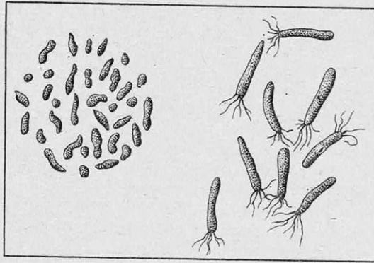
FIG. 2. — A GAUCHE, MICROBES LUMINEUX OU PHOTOBACTÉRIES NON MOBILES; A DROITE, PHOTOBACTÉRIES MUES PAR DES CILS VIBRATILES (TRÈS FORT GROSSISSEMENT)
