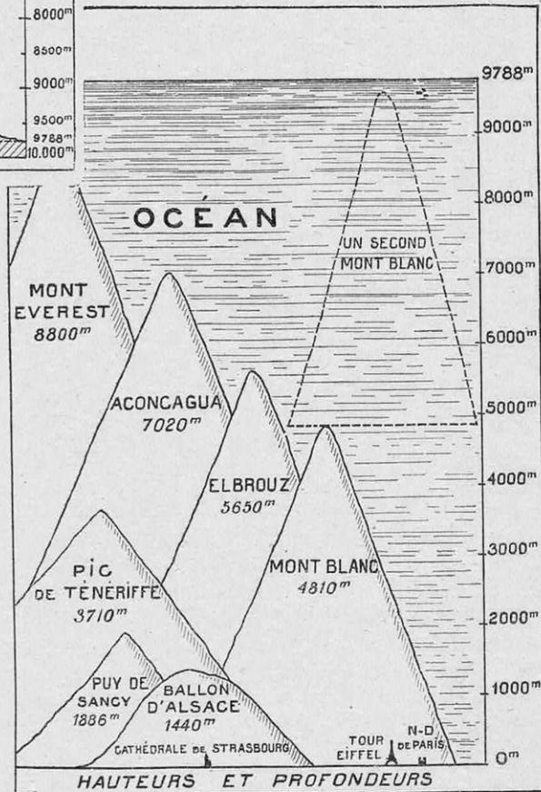
FIG. 4. - COMPARAISON DE LA PLUS GRANDE PROFONDEUR OCÉANIQUE ET DES HAUTEURS DE QUELQUES MONTAGNES ET DE QUELQUES MONUMENTS
