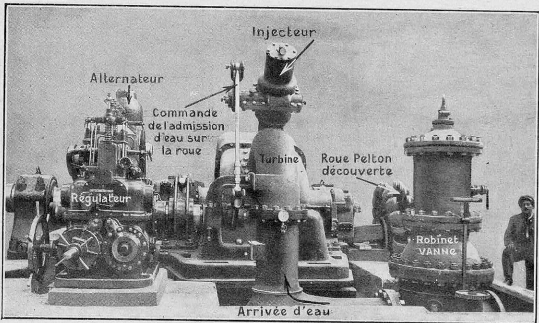
FIG. 10. — GROUPE TURBINE-ALTERNATEUR DE L'USINE HYDRO-ÉLECTRIQUE DE MIÉGEBAT, DE LA COMPAGNIE DES CHEMINS DE FER DU MIDI. PUISSANCE, 10.000 C.V. (Construit par les Ateliers de Constructions Électriques de France.)
