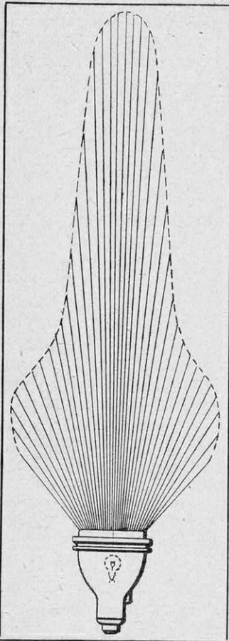
FIG. 2. — COMMENT LE PROJECTEUR MODIFIE LA COURBE POLAIRE D'UNE LAMPE
