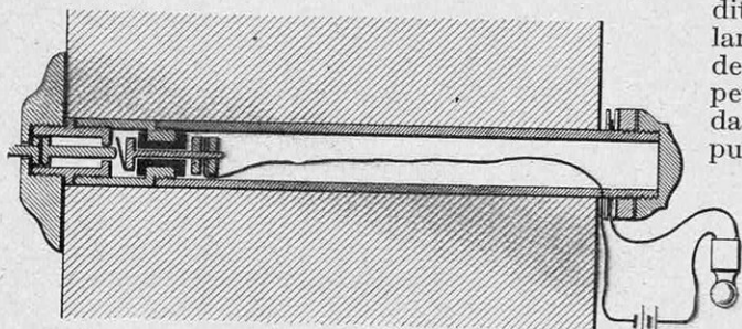
CE BOUTON DE SONNERIE, VISSÉ SUR LE TUBE QUI TRAVERSE LE MUR, ET SERRÉ PAR L'ÉCROU SITUÉ À L'EXTREMITÉ OPPOSÉE DU TUBE, NE PEUT ÊTRE DÉMONTÉ DE L'EXTÉRIEUR
