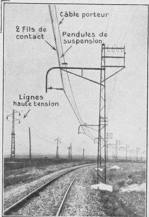
FIG. 14. — LIGNE CATÉNAIRE A COURANT CONTINU A 3.000 VOLTS ET LIGNE A HAUTE TENSION DES CHEMINS DE FER DU MAROC
