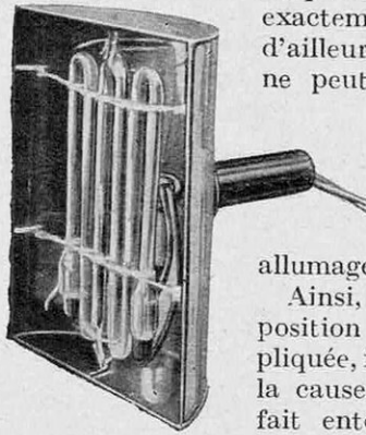
LAMPE BALADEUSE AU NÉON POUR L'EXAMEN STRO- BOSCOPIQUE
