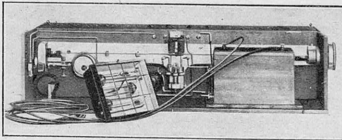
INSTALLATION COMPLÈTE DU STROBOSCOPE A LAMPE BALADEUSE AU NÉON
