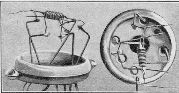
FIG. 1. - ASPECT GÉNÉRAL DE LA NOUVELLE LAMPE
