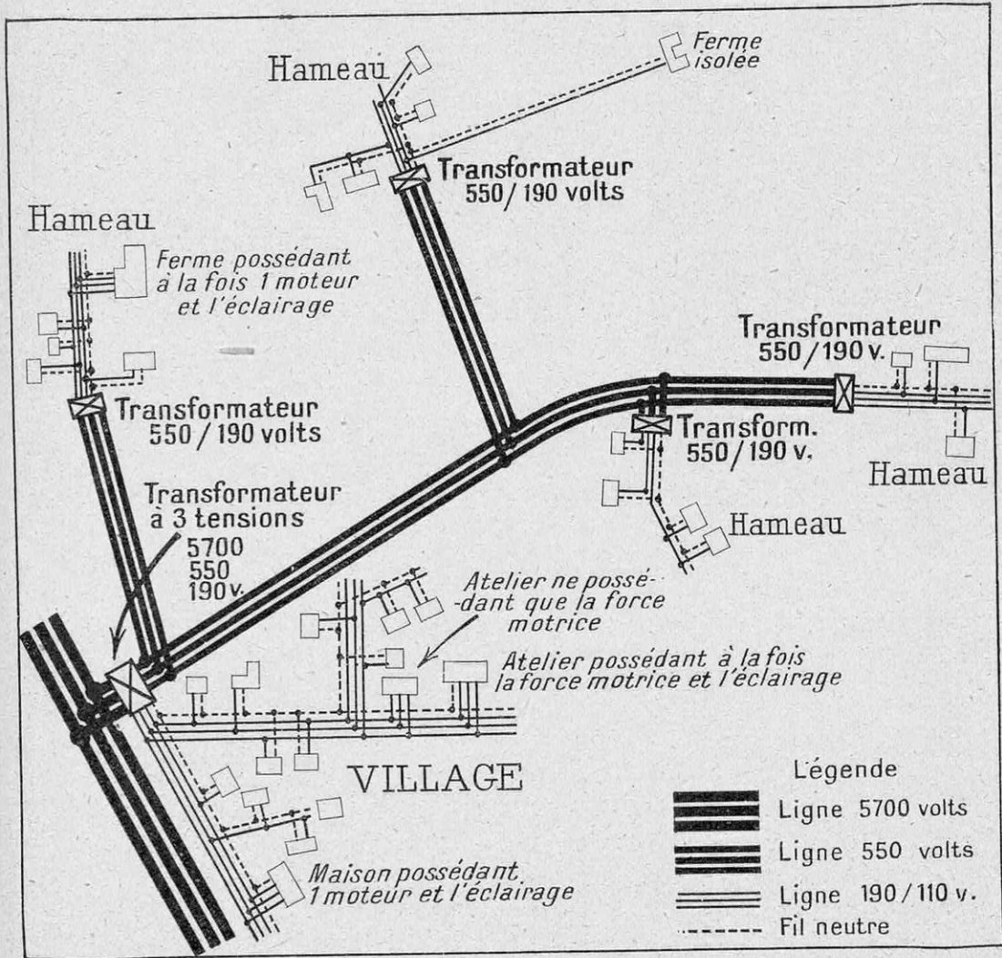
FIG. 15. — SCHEMA DE LA DISTRIBUTION D'ENERGIE ELECTRIQUE DANS LES CAMPAGNES PAR L'EMPLOI DES TRANSFORMATEURS A TROIS TENSIONS
