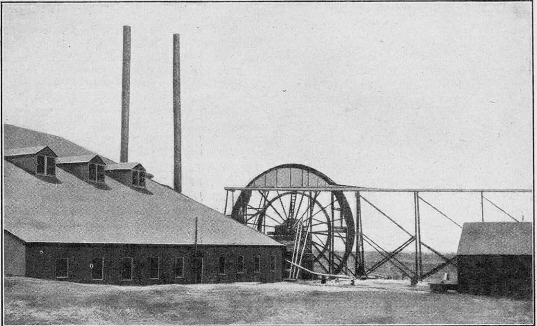
ROUE REMONTANT LES « TAILINGS » ET CANAL D'ÉVACUATION A LA MINE WEMMER Les « tailings » sont les résidus du minerai après son traitement par le mercure.
