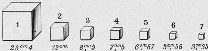
FIG. 7. — LE VOLUME RELATIF DES SEPT SELS PRINCIPAUX CONTENUS DANS UNE TONNE D'EAU DE MER
