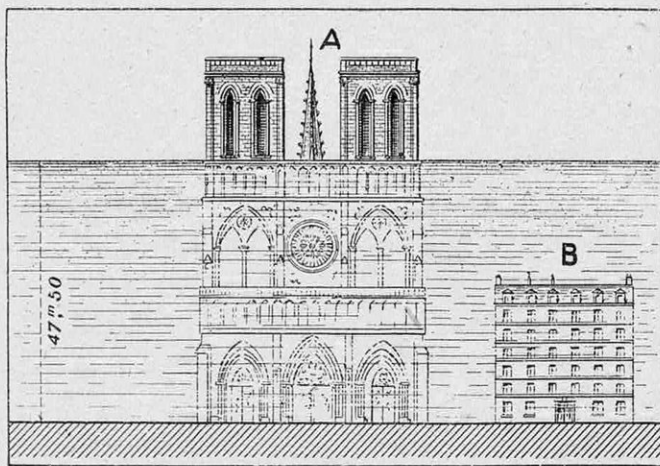
FIG. 10. — ÉTENDUE SUR LA TERRE ENTIÈRE, LA MASSE DES SELS CONTENUS DANS L'OcéAN Y FORMERAIT UNE COUCHE DE 47 M. 50 D'ÉPAISSEUR
