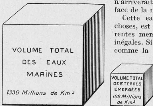
FIG. 1. - IMPORTANCES RELATIVES DU VOLUME DES EAUX OCÉANIQUES ET DE CELUI DES TERRES ÉMERGÉES
