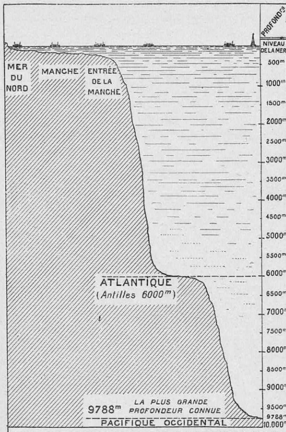
FIG. 3. — QUELQUES PROFONDEURS OCÉANIQUES
