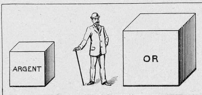
FIG. 11. — LES VOLUMES D'ARGENT ET D'OR, EXTRAITS DE LA MER, QUI REVIENDRAIENT, APRÈS PARTAGE ÉGAL, À CHACUN DES 1.500 MILLIONS D'HABITANTS DE LA TERRE
