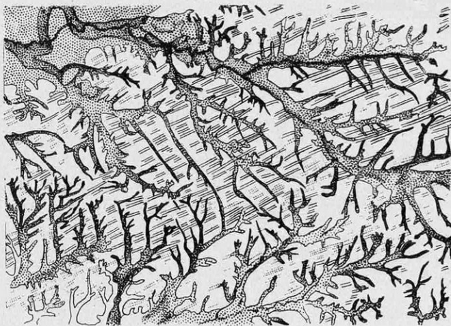
PLAN DES FILONS AURIFÈRES DE BENDIGO (AUSTRALIE)
