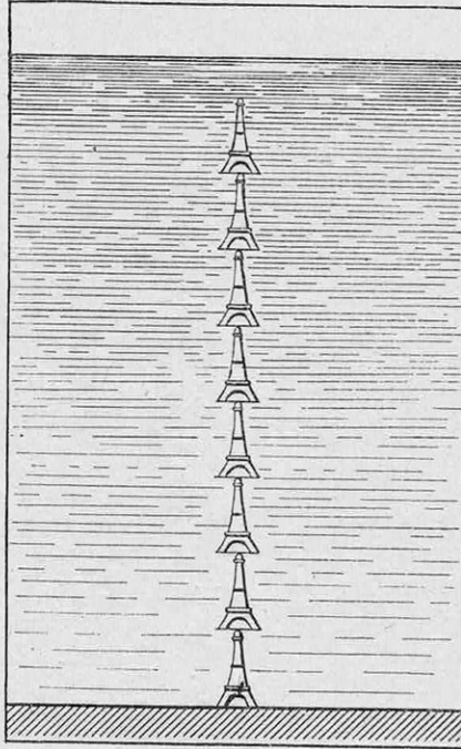
FIG. 2. — ÉTENDUES EN NAPPE UNIFORME SUR LA TERRE ENTIÈRE, LES EAUX DES MERS Y FORMERAIENT UNE COUCHE DE 2.600-MÈTRES, DONT L'ÉPAISSEUR DÉPASSERAIT LA HAUTEUR DE HUIT TOURS EIFFEL SUPERPOSÉES
