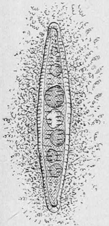
FIG. 12. — GRANDE DIATOMÉE VERTE Elle est entourée d'un amas de « Spirochaete plicatilis » attirés par le dégagement d'oxygène provoqué par la lumière.
