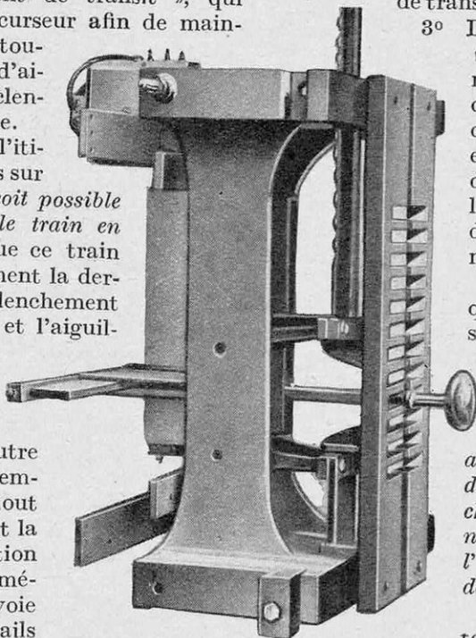
FIG. 4. - ÉLÉMENT SÉLECTEUR D'UN COMBINATEUR
