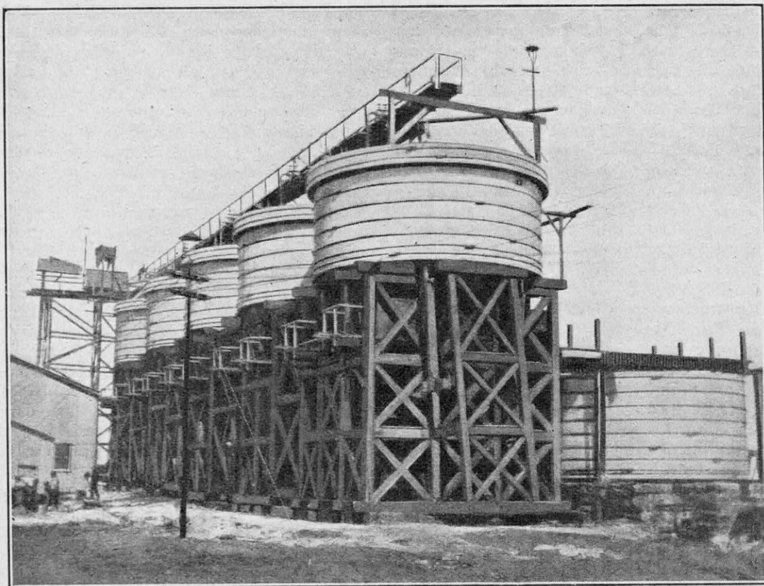
GRUPE DE CUVES DE CYANURATION DE LA « NEW COMET » (TYPE A DEUX ÉTAGES)
