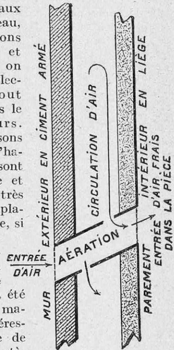
COUPE D'UN MUR PAR UN CAISSON D'AÉRATION
