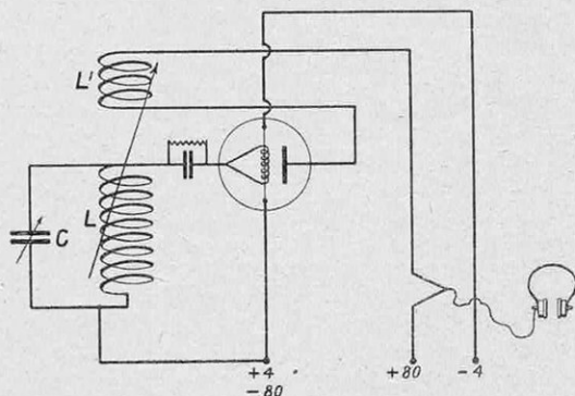
FIG. 6. — MONTAGE ORDINAIRE D'UNE LAMPE DÉTECTRICE A RÉACTION
