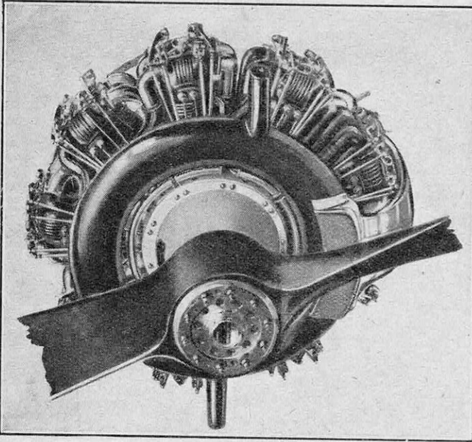
FIG. 6. — MOTEUR SALMSON DE 500 CV, A DIX-HUIT CYLINDRES A REFROIDISSEMENT PAR EAU, A DEUX COURONNES ACCOLÉES DE NEUF CYLINDRES CHACUNE
