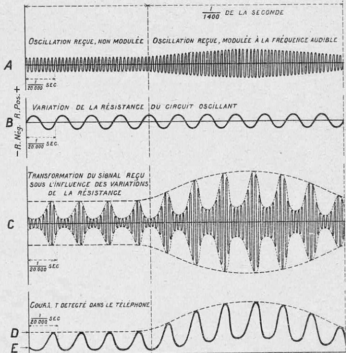
FIG. 9. — LA SUPER-RÉACTION CONSERVE LA MODULATION Côté gauche représente les oscillations reçues, non modulées; côté droit, mêmes oscillations, mais modulées. Les impulsions unilatérales E s'additionnent dans le téléphone et créent un courant modulé D.
