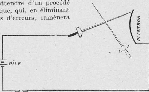
FIG. 1. — VUE D'UN SEUL CIRCUIT, MONTRANT QUE LE CONTACT DES DEUX ÉPÉES N'ENTRAÎNE AUCUNE PERTURBATION DANS CE CIRCUIT
