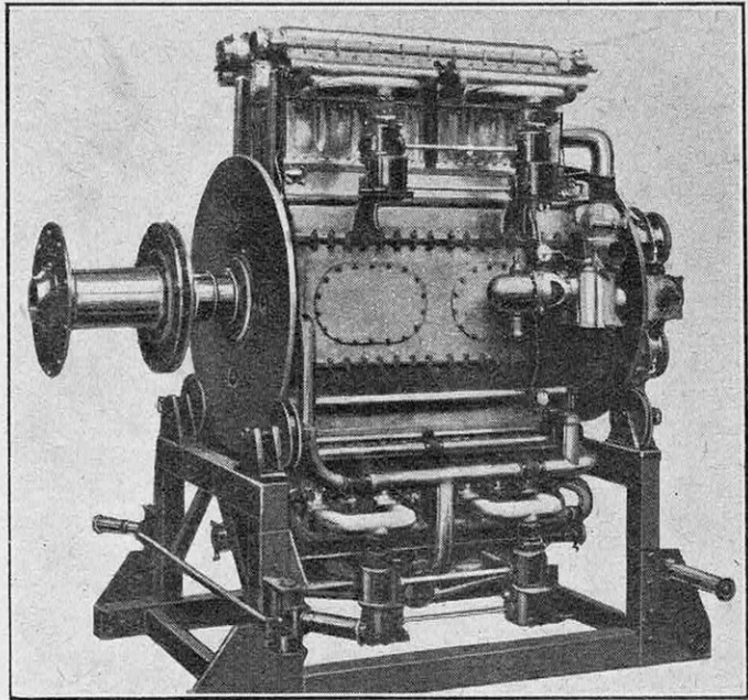
FIG. 5. — MOTEUR BRÉGUET DE 1.000 CV, A TRENTE-DEUX CYLINDRES SUR QUATRE RANGÉES DE HUIT CYLINDRES PARALLÈLES, COMMANDANT CHACUNE UN VILEBREQUIN, DEUX RANGÉES EN HAUT ET DEUX RANGÉES EN BAS, INVERSÉES
