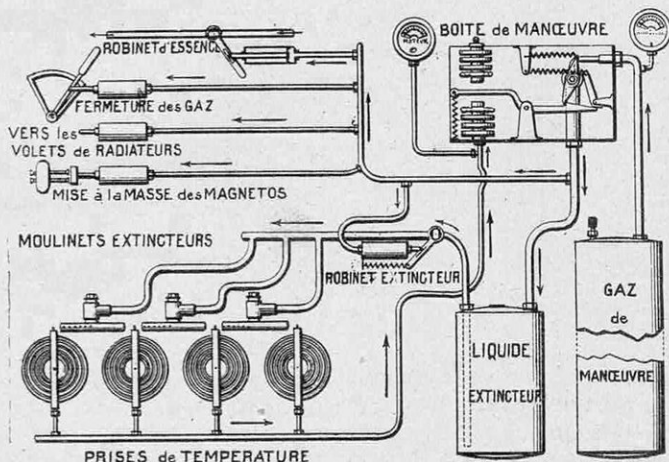
FIG. 1. — ENSEMBLE SCHÉMATIQUE DE L'« AVERTISSEUR- EXTINGUEUR » AUTOMATIQUE BÉCHARD
