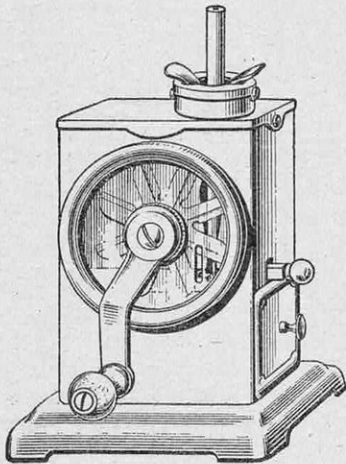
VUE EXTERIEURE DE LA MACHINE A TAILLER LES CRAYONS
