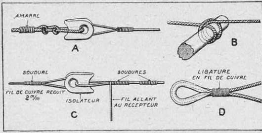
PLANCHE 8. — DÉTAILS D'ASSEMBLAGE DE L'ANTENNE
