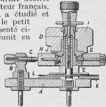
CONDENSATEUR SHUNTÉ PAR UNE RÉSISTANCE RÉGLABLE, LA CAPACITÉ DE DÉTECTION ÉTANT ELLE-MÊME VARIABLE
