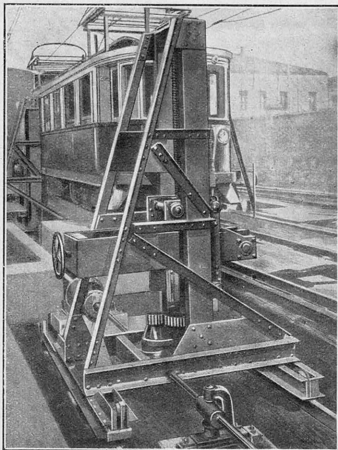
DÉTAIL D'UN VÉRIN ÉLECTRO-MAGNÉTIQUE
