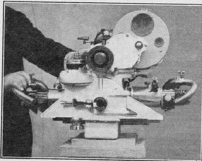
FIG. 13. — MOTEUR DE DÉMARRAGE A EXPLOSIONS, DEUX CYLINDRES, SYSTÈME TAMPIER
