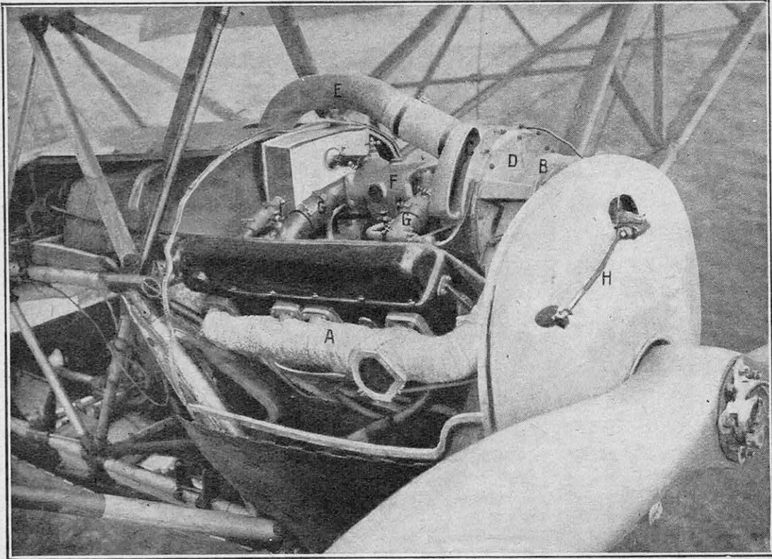
FIG. 8. — MONTAGE DU TURBO-COMPRESSEUR RATEAU SUR LE MOTEUR HISPANO, 300 CV, DE L'AVION GOURDOU DU RECORD D'ALTITUDE (12.000 MÈTRES)
