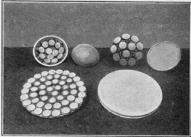
« BALLES » ET « BASSINS » POUR LE TRAVAIL DU VERRE Suivant la forme des surfaces à obtenir, on place les pièces de verre sur des surfaces planes, convexes ou concaves, et, par frottement sur une forme complémentaire, avec interposition d'abrasif de plus en plus fin, on leur donne un poli parfait.
