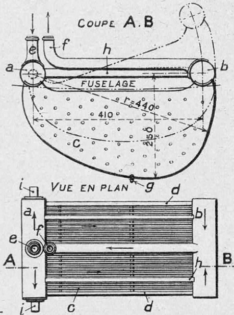
FIG. 11. — SCHÉMA DU RADIATEUR LAMBLIN A LAMES, EN PARTIE ESCAMOTABLE Les flèches indiquent le trajet de l'eau. e, arrivée de l'eau ; f, départ ; a et b, collecteurs ; c, lames d'eau constituées par deux parois en cuivre de quelques dixièmes de millimètre.
