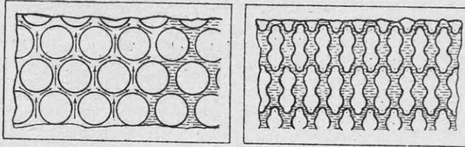
FIG. 12. — ÉLÉMENT DU RADIATEUR « NID D'ABEILLES », A TUBES CYLINDRIQUES ORDINAIRES, A GAUCHE, ET TUBES OVALES ET GAUFRÉS, A DROITE. L'EAU PASSE ENTRE LES TUBES ET L'AIR DEDANS
