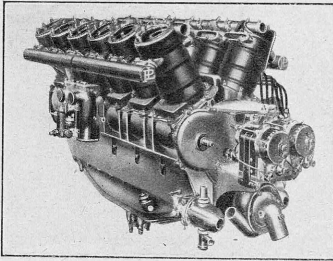
FIG. 9 — MOTEUR PANHARD-LEVASSOR, DE 500 CV, A FOURREAUX DISTRIBUTEURS EN ACIER
