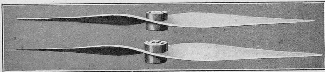
FIG. 1. — HÉLICE MÉTALLIQUE LEVASSOR (LICENCE REED) EN DURALUMIN
