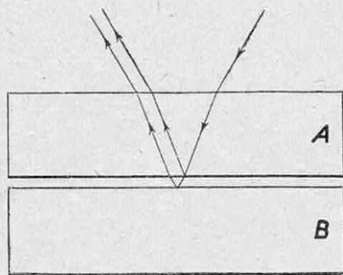
COMMENT SE PRODUISENT LES INTERFÉRENCES LUMINEUSES
