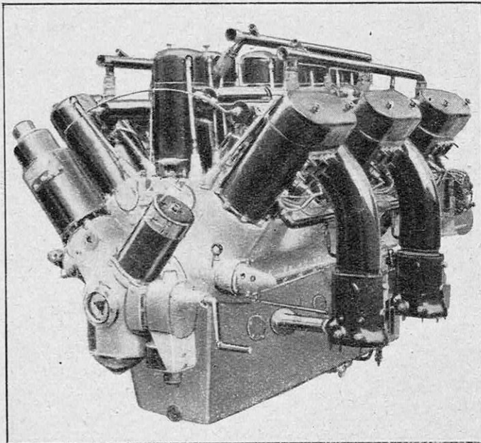
FIG. 4. — MOTEUR FARMAN, 600-700 CHEVAUX, DIX-HUIT CYLINDRES
