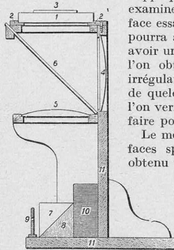
DISPOSITIF POUR L'OBSERVATION DES FRANGES LUMINEUSES
