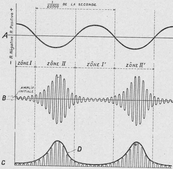
FIG. 11. — PRINCIPE DE LA SUPER-RÉACTION
