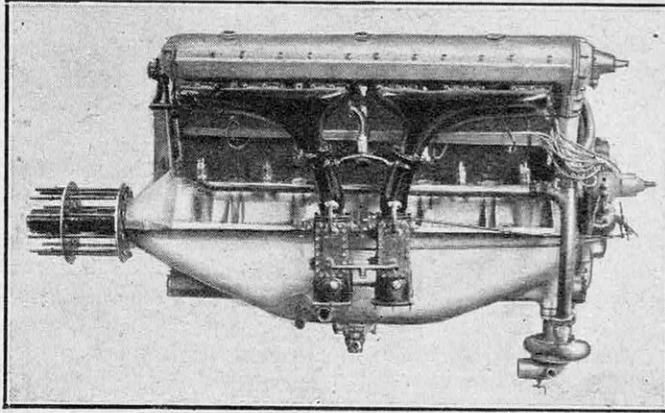
FIG. 2. — MOTEUR RENAULT, 600 CV, COMPORTANT DOUZE CYLINDRES EN V
