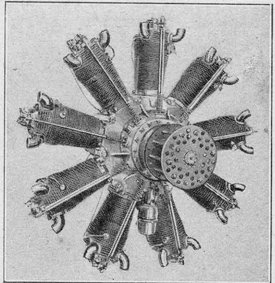
FIG. 7. — MOTEUR GNOME-RHONE JUPITER. 400 CV, A REFROIDISSEMENT PAR AIR 9 cylindres en étoile. Alésage : 146 millimètres ; course : 190 millimètres ; poids : 350 kilogrammes ; puissance : 400 CV à 1.700 tours.
