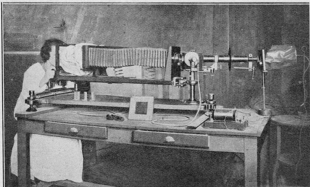
FIG. 3. — LE SPECTROGRAPHE A « INFRA-ROUGE »
