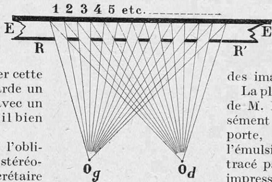
COMMENT, AU MOYEN D'UNE SEULE PLAQUE, ON PEUT RÉALISER LA VISION EN RELIEF
