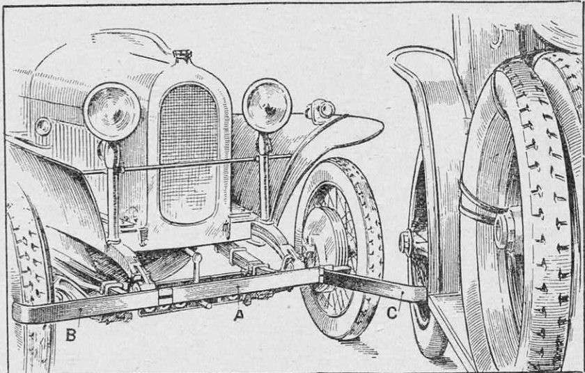
SYSTÈME DE PARE-CHOC AVEC DÉCLENCHEMENT AUTOMATIQUE DES EXTRÉMITÉS MOBILES
