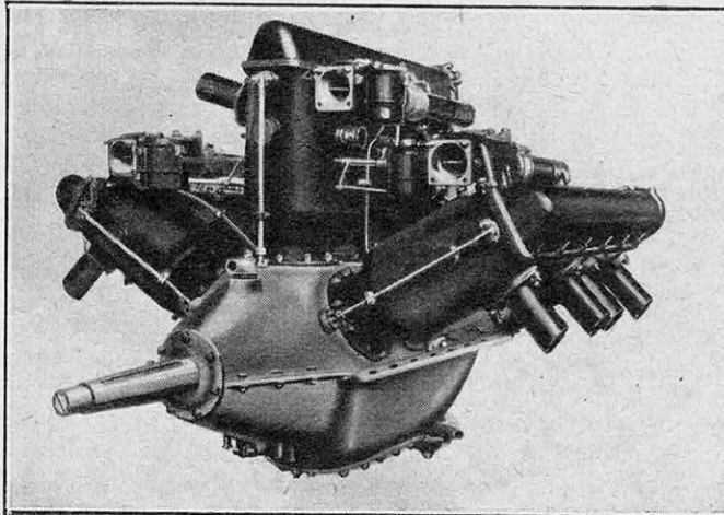
FIG. 3. — MOTEUR HISPANO-SUIZA, 450-600 CV, DOUZE CYLINDRES EN TROIS RANGÉES DE 4 A 60°
