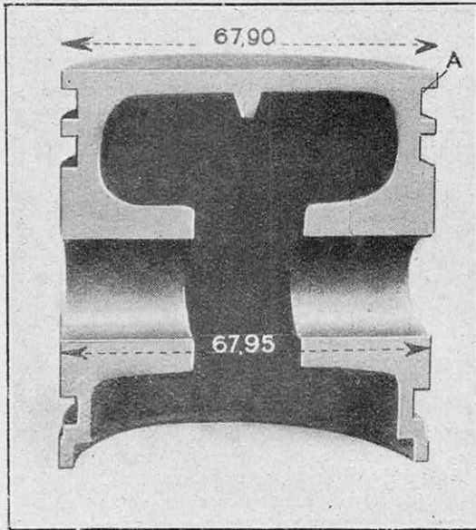
COUPE D'UN PISTON EN FONTE POUR UN MOTEUR DE 68 MILLIMÈTRES D'ALÉSAGE
