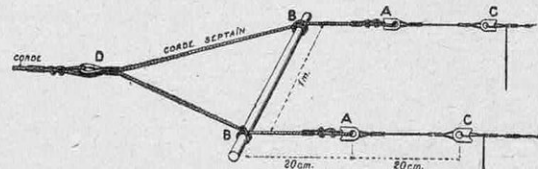
FIG. 9. — ANTENNE BIFILAIRE
