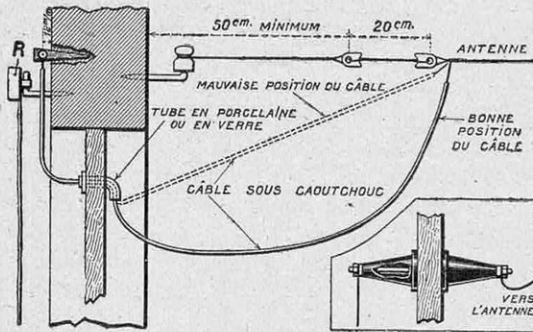
FIG. 10. — ENTRÉES DU POSTE
