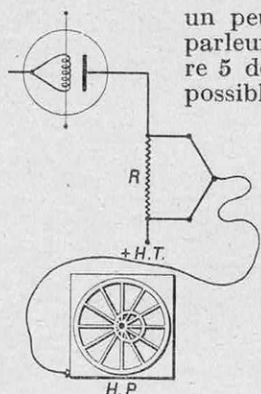
FIG. 5. — MONTAGE DU HAUT-PARLEUR ÉLECTROSTATIQUE APRÈS LA LAMPE AMPLIFICATEUR
