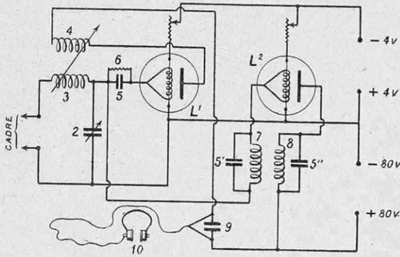
FIG. 7. — SUPER-RÉACTION A DEUX LAMPES
