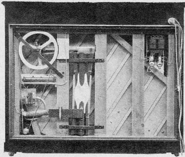
VUE DE DOS DE L'APPAREIL AUTOMATIQUE S'ADAPTANT SUR UN PIANO ORDINAIRE
