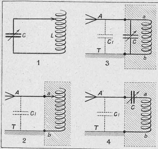
PLANCHE 2. — ANALOGIE ENTRE UN CIRCUIT OSCILLANT ET UN CIRCUIT D'ANTENNE
