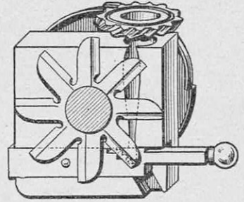
VUE INTERIEURE DE LA MACHINE MONTRANT LES LAMES EN ÉTOILE ET LE LOGEMENT DU CRAYON
