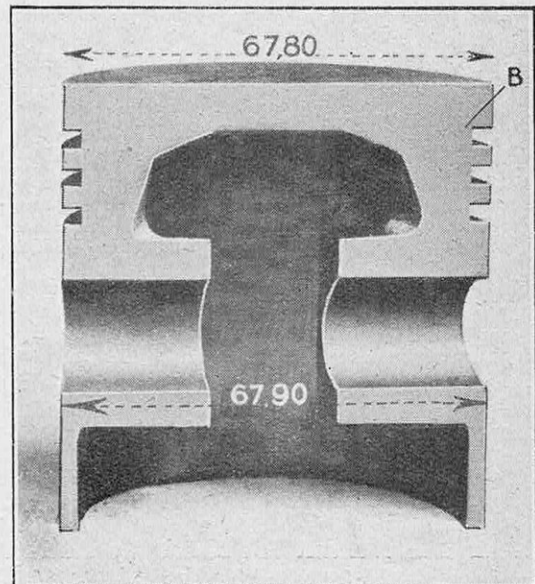
COUPE D'UN PISTON EN ALLIAGE ALPA X, POUR UN MOTEUR DE 68 MILLIMÈTRES D'ALÉSAGE
