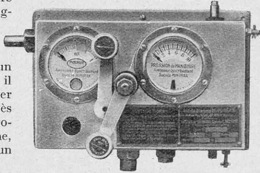
FIG. 2. — VUE EXTÉRIEURE DE LA BOÎTE DE MANŒUVRE
