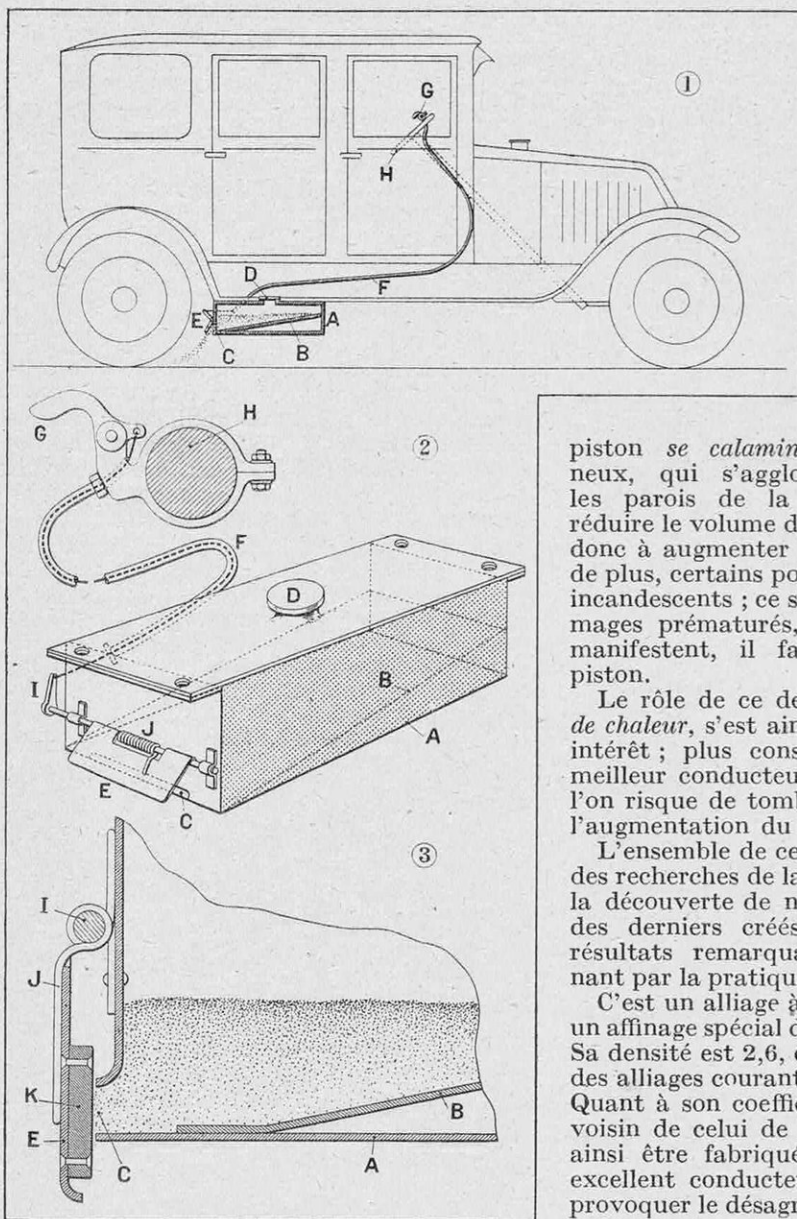
DÉTAILS D'INSTALLATION DE SABLIERES SUR UNE AUTOMOBILE
