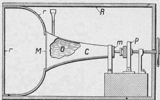
FIG. 1. — HAUT-PARLEUR A DEUX MEMBRANES RÉUNIES PAR UNE COLONNE LIQUIDE r' , paroi de résonance; r , petit pavillon; M , membrane reproductrice; O , liquide transmettant les vibrations du m à M ; m , membrane motrice; P , électrociment du haut-parleur.
