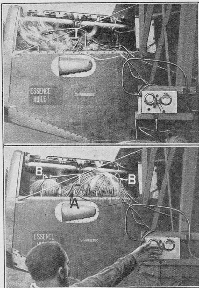
FIG. 4. — INSTALLATION ET FONCTIONNEMENT A MAIN DU DISPOSITIF BÉCHARD SUR UN AVION ANSALDO-FIAT
