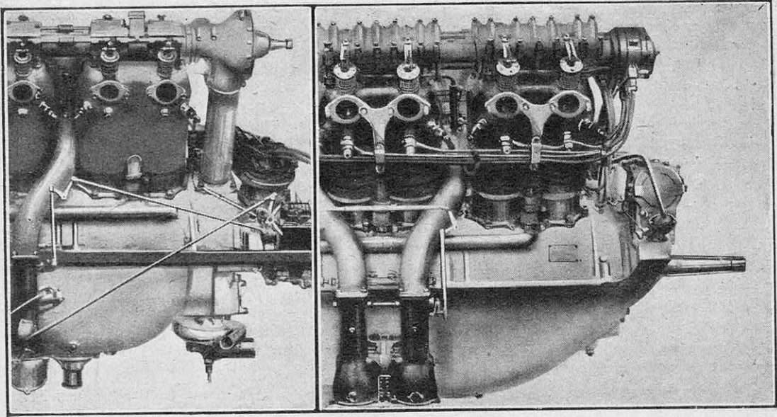
FIG. 10. — MOTEUR LORRAINE-DIÉTRICH, 370 CV (A GAUCHE), TRANSFORMÉ EN 400 CV (A DROITE) Les modifications visibles portent sur : le carter d'arbre à cames (étanchéité du graissage), le chemisage des cylindres (chemise légèrement ondulée se prêtant mieux aux dilatations), l'installation du démarrage à air carburé, le réchauffage du corps des carburateurs, la fixation des collerettes des ressorts de soupapes.
