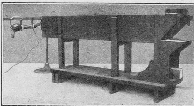
PHOTOGRAPHIE DE L'APPAREIL A EXAMINER LES FRANGES. A GAUCHE, LA SOURCE DE LUMIERE MONOCHROMATIQUE. On reconnaît, sur la partie droite, le dispositif dont le schéma est indiqué à la page précédente.
