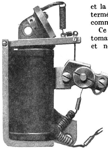
FIG. 5. — L'ÉLECTRO-AIMANT DU COMMUTATEUR ROTATIF
