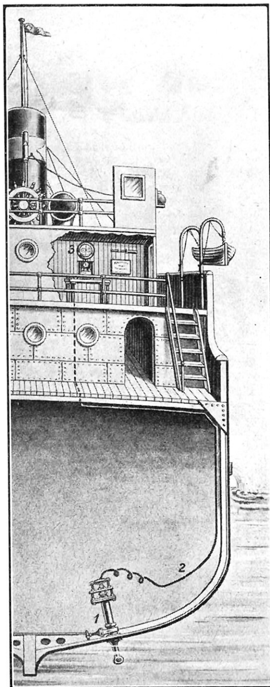
FIG. 2. — INSTALLATION GÉNÉRALE DU LOCH ÉLECTRIQUE A BORD D'UN NAVIRE
