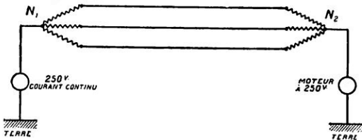
FIG. 2. — MONTAGE POUR RÉSEAUX TRIPHASÉS
