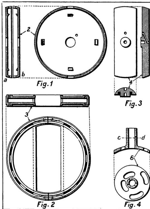
PLANCHE 2. — DÉTAIL DES PIÈCES INTÉRIEURES DU MOTEUR SPHÉRIQUE
