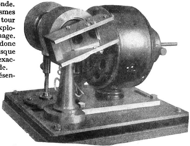
FIG. 8. — GROUPE MOTEUR ET PORTE-PRISMES
