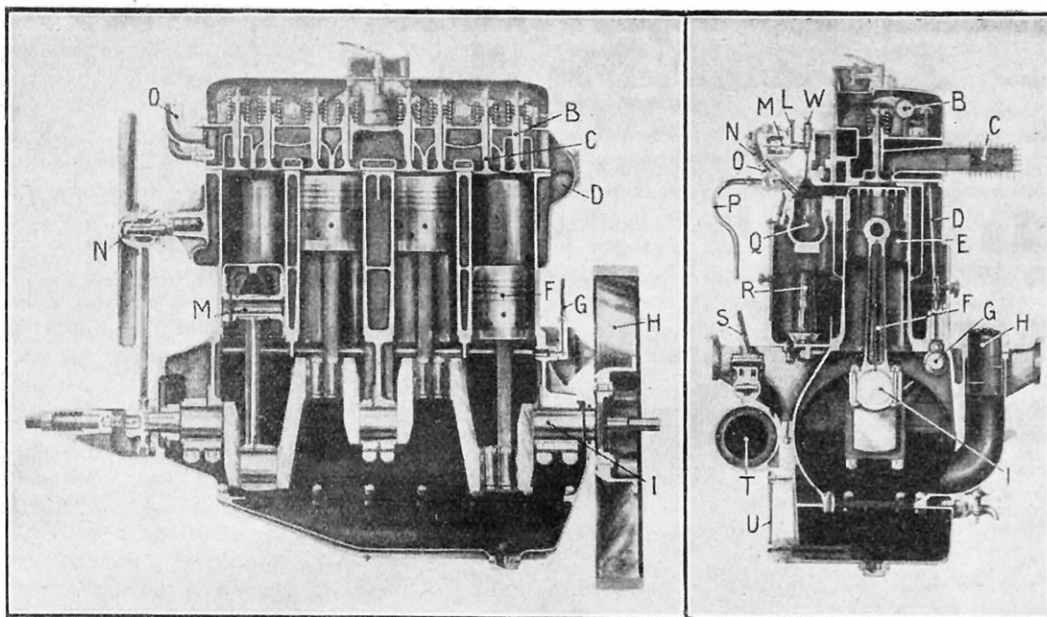
COUPE EN LONG ET EN TRAVERS DU MOTEUR ITALIEN BAGNULO
