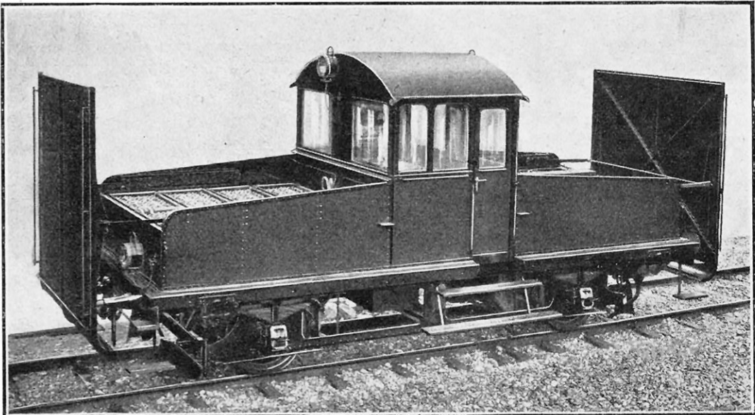
LOCOMOTIVE POUR VOIE NORMALE COMPORTANT DEUX MOTEURS DE 100 CHEVAUX
