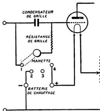
SCHÉMA DE CONSTRUCTION D'UN COMMUTATEUR SIMPLE DE RÉSISTANCE DE GRILLE
