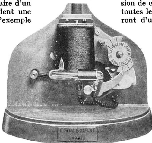
TÉLÉRUPTEUR-SÉLECTEUR EMPLOYÉ POUR LA COMMANDE A DISTANCE SANS FIL PILOTE ET PAR COURANT A BAS VOLTAGE (Côté télérupteur proprement dit.)
