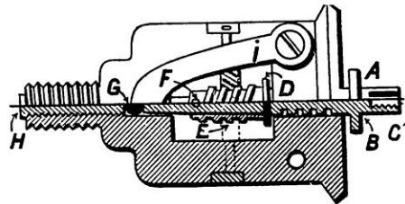
FIG. 5. — LA BOÎTE DE CONTACT DU LOCH C'est la coupe de la boîte A, déjà représentée sur la planche 4, à plus petite échelle : A, axe porte-hélice du loch ; B, bride ; C, filetage pour la vis de fixation ; D, support du ressort I ; E et F, vis sans fin en prise directe ; G, bille du palier ; H, filetage de l'écrou de serrage B (fig. 4, à droite).
