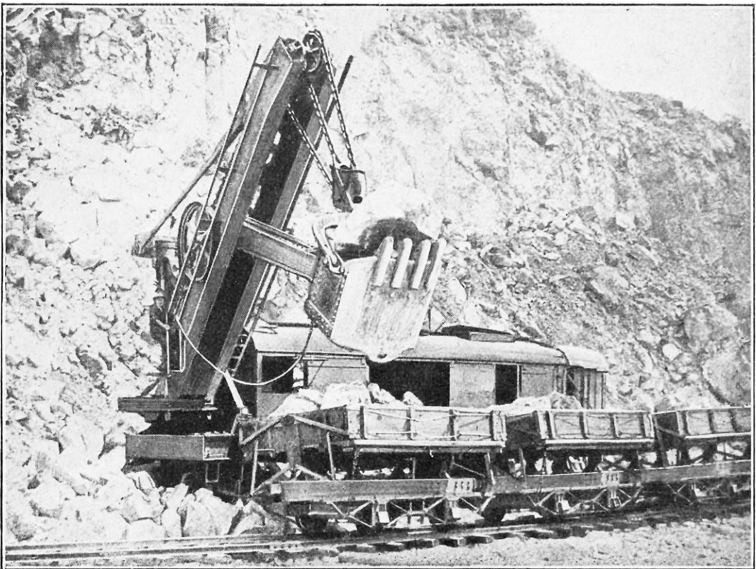
FIG. 3. — PELLE ROTATIVE D'EXCAVATION A DÉBIT TRÈS IMPORTANT Cet appareil, très robuste, est surtout employé pour le creusement des tranchées de voies ferrées.
