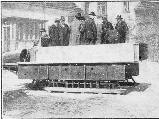
VUE LATÉRALE DE L'AUTOMOBILE A PATINS
