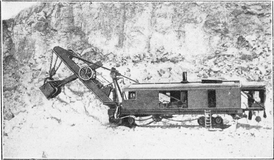
FIG. 2. — TYPE DE PELLE ROTATIVE ACTIONNÉE PAR LA VAPEUR L'ensemble repose sur une section de voie ferrée par l'intermédiaire de deux bogies.
