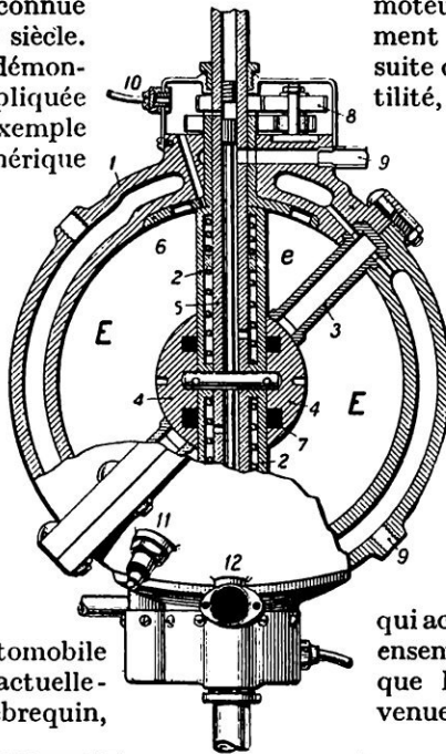
FIG. 1. — COUPE ET VUE EXTÉRIEURE PARTIELLE DU NOUVEAU MOTEUR ROTATIF SPHÉRIQUE A EXPLOSION
