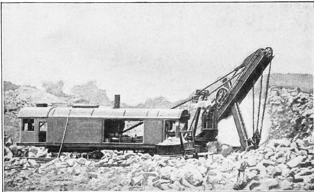
FIG. 4. — PELLE ROTATIVE A VAPEUR AMÉRICAINE DU TYPE « BUCYRUS »
