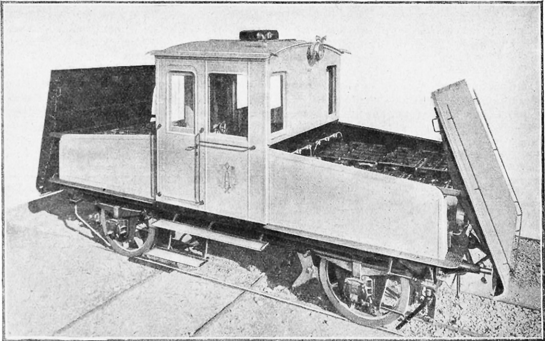
LOCOMOTIVE DE 25 TONNES POUR CHANTIERS, D'UNE PUISSANCE DE 110-120 CHEVAUX VITESSE : 12-25 KILOMÈTRES-HEURE; TENSION : 330 VOLTS
