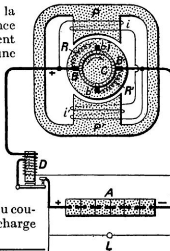
FIG. 4. — PETITE DYNAMO A QUATRE BALAIS, SYSTÈME KIRBY-SMITH
