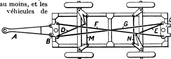
DISPOSITIF D'UNE REMORQUE A PALONNIERS A, timon d'attelage ; B C, palonniers ; D E F G, tiges de liaison des palonniers ; M N, barres d'accouplement des roues.
