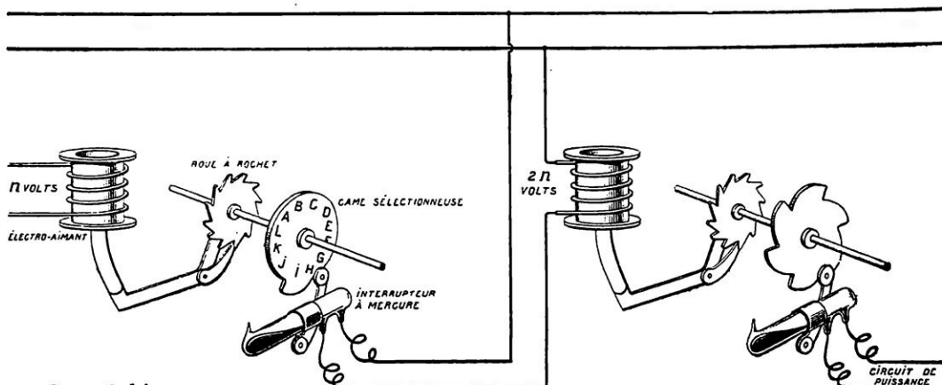
FIG. 9 ET 9 bis. — TÉLÉRUPTEURS A CAME SÉLECTIVE MONTÉS EN SÉRIE POUR PERMETTRE, CELUI DE GAUCHE, DE SÉLECTIONNER LES APPAREILS A COMMANDER, CELUI DE DROITE, D'EFFECTUER LES COMMANDES
