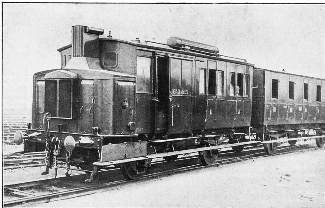
ASPECT GÉNÉRAL DE L'AUTOMOTRICE, SYSTÈME SCHNEIDER, ADOPTÉE PAR LES CHEMINS DE FER DE L'ÉTAT
