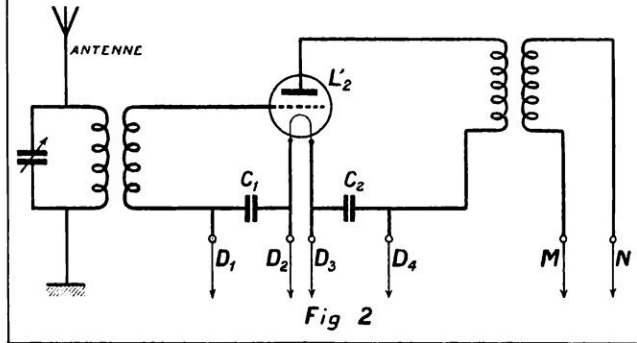
SCHÉMAS DE MONTAGE D'UN APPAREIL TRANSFORMÉ POUR LA DOUBLE AMPLIFICATION
