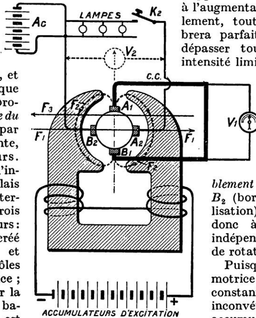
FIG. 2. — LA DYNAMO A QUATRE BALAIS EN QUADRATURE (90 DEGRÉS)
