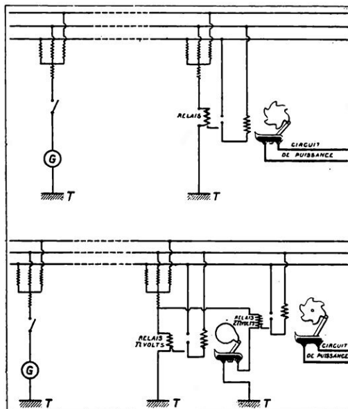
FIG. 10 ET 11. — APPLICATION DU COURANT CONTINU DE 12 VOLTS ET DE LA SÉLECTION PARTIELLE OU TOTALE
