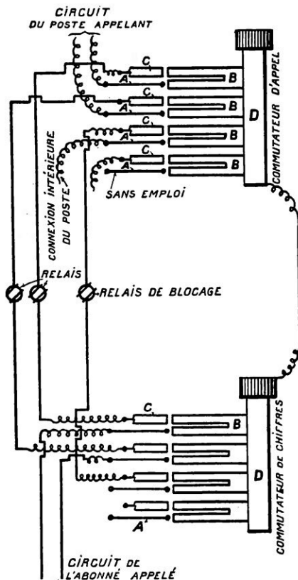
FIG. 2. — DÉTAIL DES COMMUTATEURS ROTATIFS
