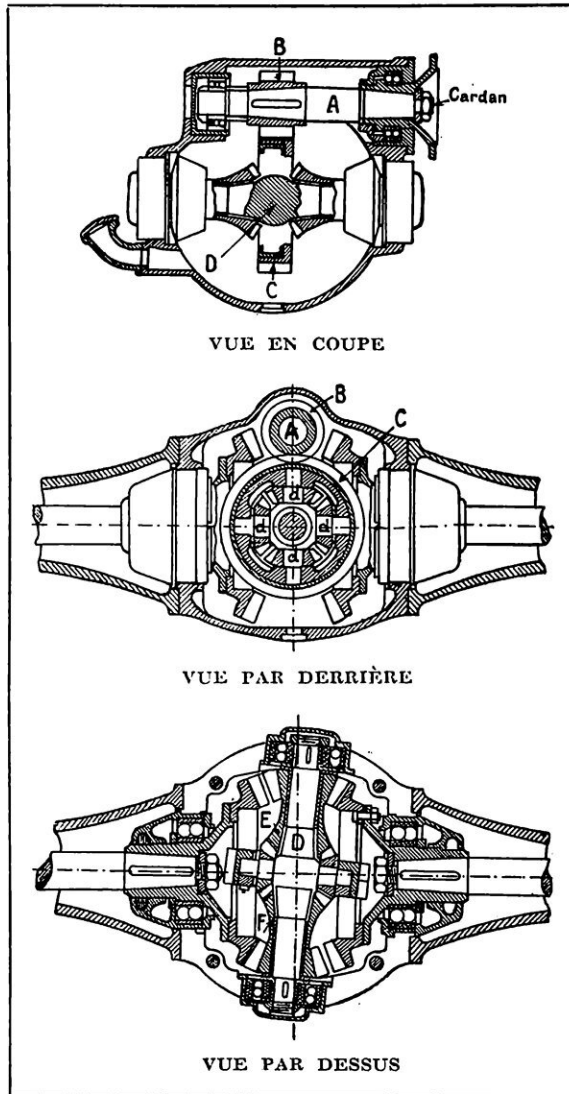
A, arbre de commande ; B, pignon de commande avec une roue C fixée sur les extrémités des quatre branches du croisillon ; E, F, pignons fous sur l'arbre D.
