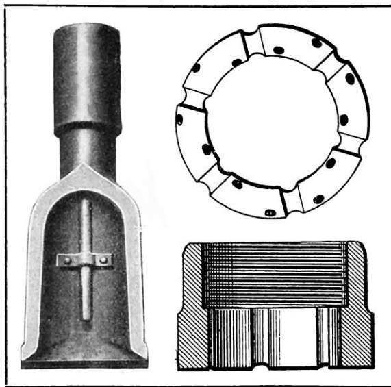
FIG. 2. — OUTILS D'ATTAQUE DES TERRAINS EMPLOYÉS DANS LES SONDAGES
