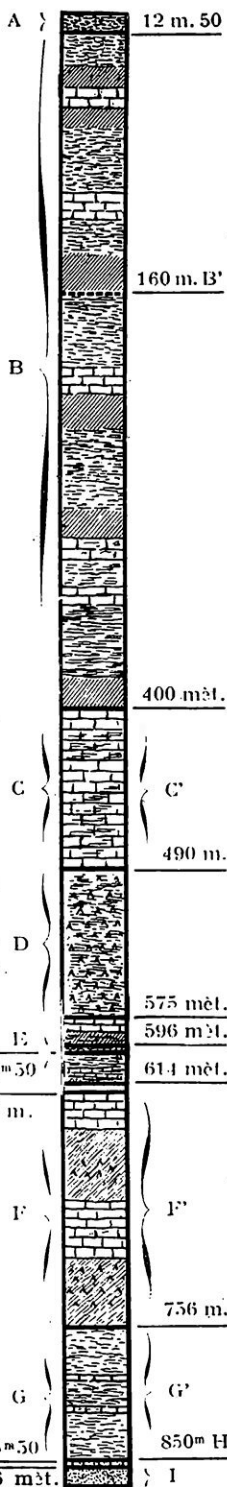
FIG. 8. — COUPE GÉOLOGIQUE D'UN TERRAIN PÉTROLIFÈRE, PRÈS DE CLERMONT-FERRAND
