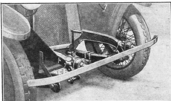
PARE-CHOC AVANT POUR VOITURE AUTOMOBILE
