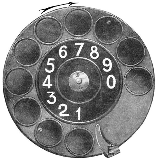
FIG. 6. — LE DISQUE D'APPEL PLACÉ SUR LE PIED DE L'APPAREIL TÉLÉPHONIQUE
