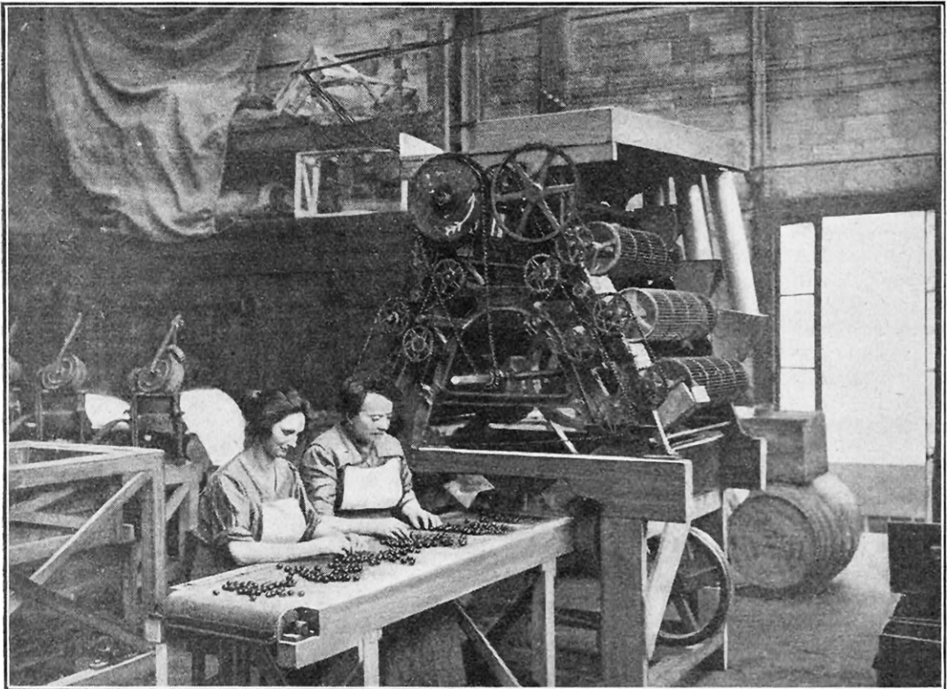
VUE DE COTÉ DE LA MACHINE, AVEC LE TAPIS ROULANT SUR LEQUEL TOMBENT LES CERISES ET OU SE FAIT LE TRI
