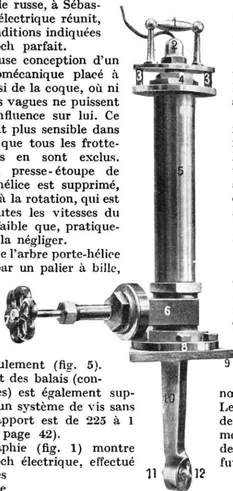
FIG. 3. — VUE D'ENSEMBLE DU LOCH ÉLECTRIQUE.
