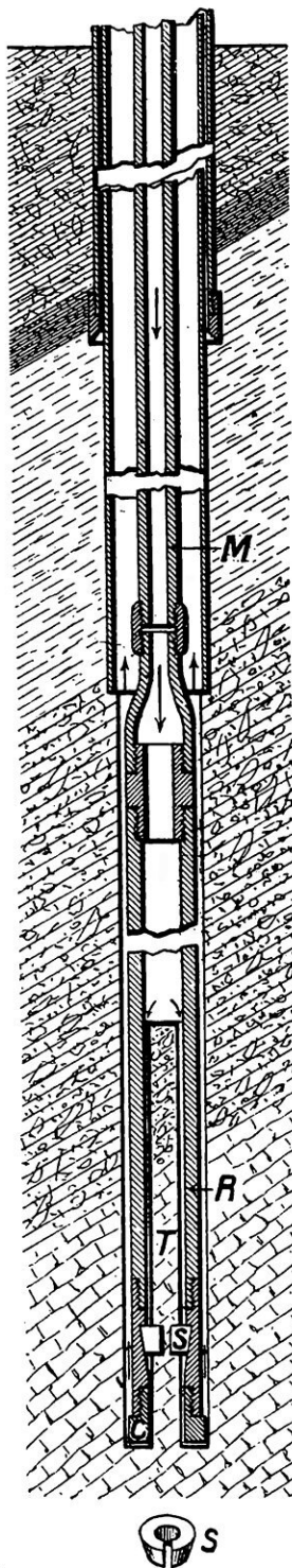
FIG. 3. — MODE D'ACTION D'UNE COURONNE, AVEC PRISE DE « CAROTTE »
