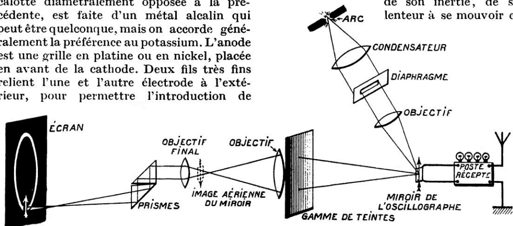
FIG. 12. — DESSIN SCHÉMATIQUE MONTRANT LA MARCHÉ DES RAYONS LUMINEUX POUR REPRODUIRE, A L'ARRIVÉE, LA COURONNE LUMINEUSE SUR UN ÉCRAN
