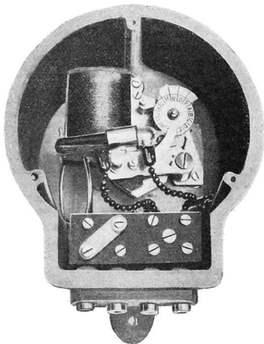
TÉLÉRUPTEUR-SÉLECTEUR POUR COMMANDE A DISTANCE PAR FIL PILOTE
