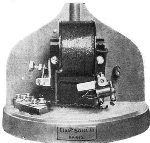
TÉLÉRUPTEUR - SÉLECTEUR EMPLOYÉ POUR LA COMMANDE A DISTANCE SANS FIL PILOTE ET PAR COURANT A BAS VOLTAGE (Vue côté relais.)
