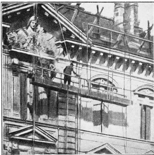
LA VAPEUR A HAUTE PRESSION DÉCRASSE SANS USER LA PIERRE
