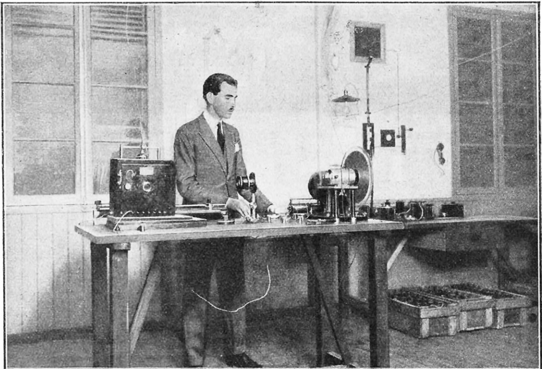
FIG. 1. — ENSEMBLE DES APPAREILS TRANSMETTEURS D'UN POINT LUMINEUX
