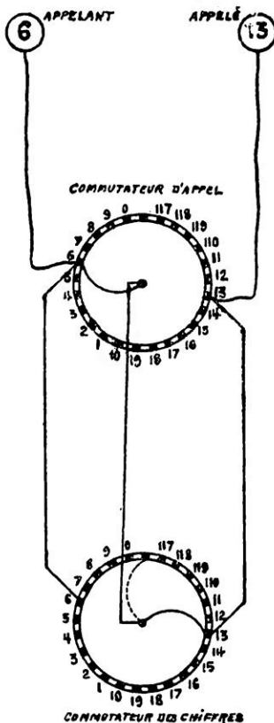
FIG. 7. — SCHEMA DE MISE EN COMMUNICATION DES DEUX ABONNÉS 6 ET 13.
