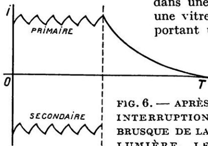
FIG. 6. — APRÈS INTERRUPTION BRUSQUE DE LA LUMIÈRE, LE COURANT INDUIT DANS LE SECONDAIRE DU TRANSFORMATEUR « T » (FIG. 3) CESSE BRUSQUEMENT, TANDIS QUE, DANS LE PRIMAIRE, ON RECUEILLE DU COURANT CONTINU D'ALLURE DÉCROISSANTE
