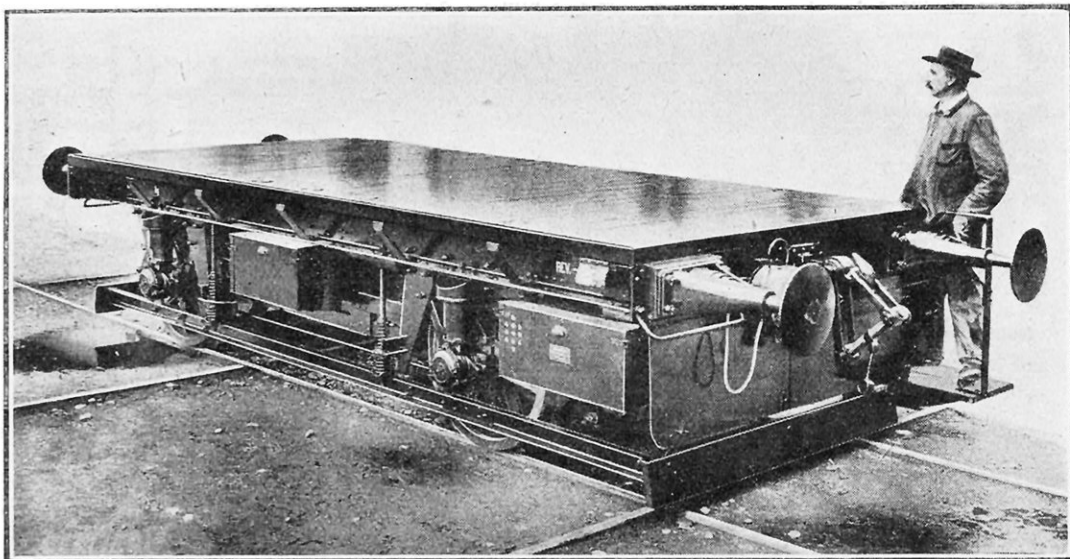
TRACTEUR A PLATE-FORME DE 8 TONNES 5 ; PUISSANCE : 20 CHEVAUX ; VITESSE : 5-8 KILOMÈTRES-HEURE ; TENSION : 280 VOLTS ; LIMITE DE CHARGE : 10 TONNES
