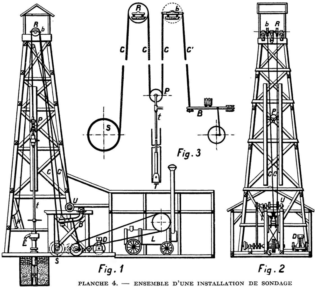
PLANCHE 4. — ENSEMBLE D'UNE INSTALLATION DE SONDAGE
