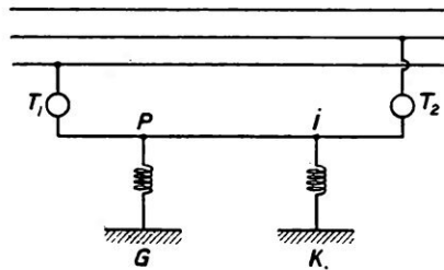
FIG. 8. — CAS OU LES RELAIS N'OFFRENT PAS UNE SELF-INDUCTION SUFFISANTE
