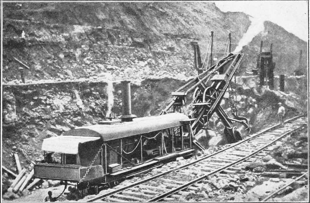
FIG. 5. — PELLE ROTATIVE A VAPEUR EMPLOYÉE POUR LES TRAVAUX D'EXCAVATION DE LA DERNIÈRE SECTION DU CANAL DE PANAMA
