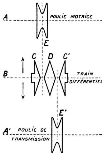
SCHÉMA DE LA TRANSMISSION PAR COURROIE ARTICULÉE
