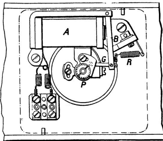
FIG. 3. — LE COMMUTATEUR ROTATIF VU EN PLAN
