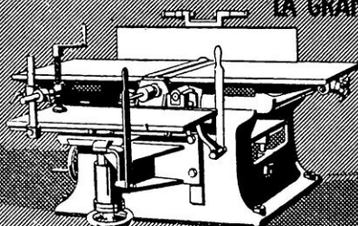
RABOTEUSE - DEGAUCHISSEUSE MORTAISEUSE DE 250%
