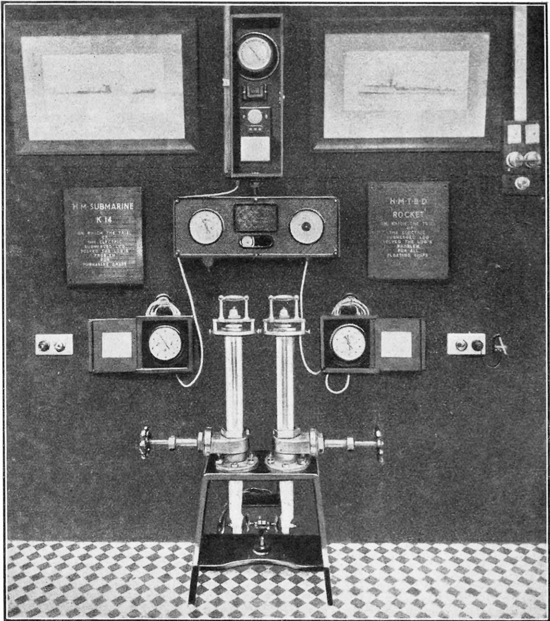
FIG. 7. — STAND DES LOCHS ÉLECTRIQUES SOUS-MARINS DU CAPITAINE CHERNIKEEFF, A L'EXPOSITION INTERNATIONALE DE L'OLYMPIA (LONDRES, 1923)
