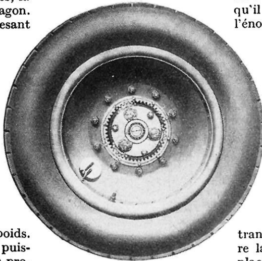
DISPOSITIF DE DÉMULTIPLICATION DANS LE MOYEU MÊME D'UNE ROUE DE CAMION
