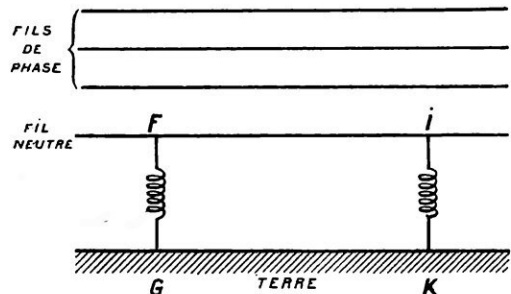
FIG. 5. — MONTAGE SPÉCIAL LA OU EXISTE UN FIL D'ÉQUILIBRE OU FIL NEUTRE
