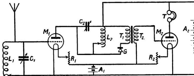
DISPOSITION D'UN CIRCUIT RÉCEPTEUR DANS LEQUEL UNE LAMPE EST UTILISÉE COMME AMPLIFICATEUR A HAUTE FRÉQUENCE
