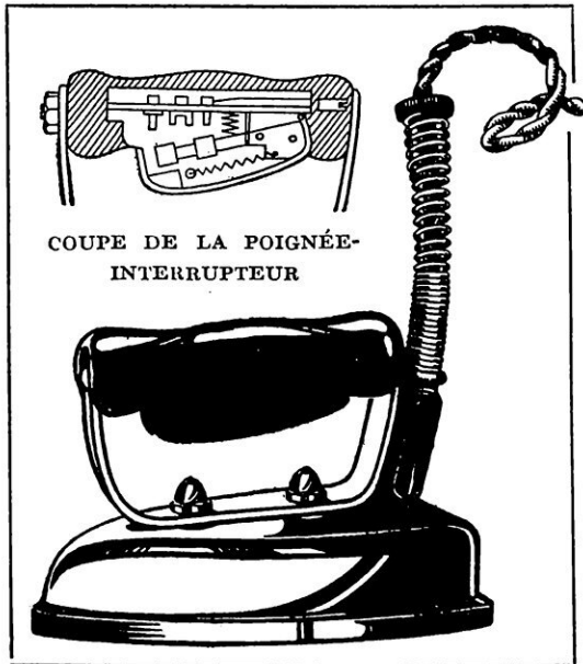
IL SUFFIT DE SAISIR OU LACHER LA POIGNÉE POUR METTRE LE FER SOUS TENSION OU, AU CONTRAIRE COUPER SON ALIMENTATION
