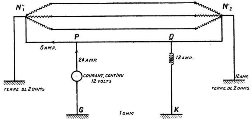
FIG. 6. — CAS OÙ LES CONDUCTEURS « N_1'' P , P Q ET Q N_2'' » POSÈSENT UNE RÉSISTANCE OHMIQUE D'UNE CERTAINE IMPORTANCE
