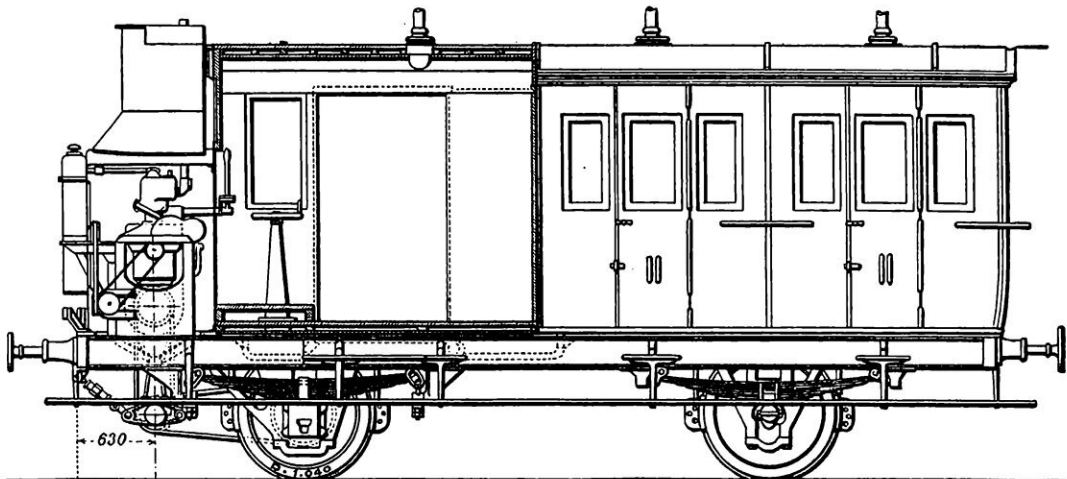
COUPE D'UNE VOITURE DE L'ÉTAT TRANSFORMÉE EN AUTOMOTRICE (SYSTÈME SCHNEIDER) On voit, de gauche à droite : le moteur et sa transmission par chaîne, le poste du conducteur, un compartiment à bagages, deux compartiments ordinaires de seconde classe pour voyageurs.
