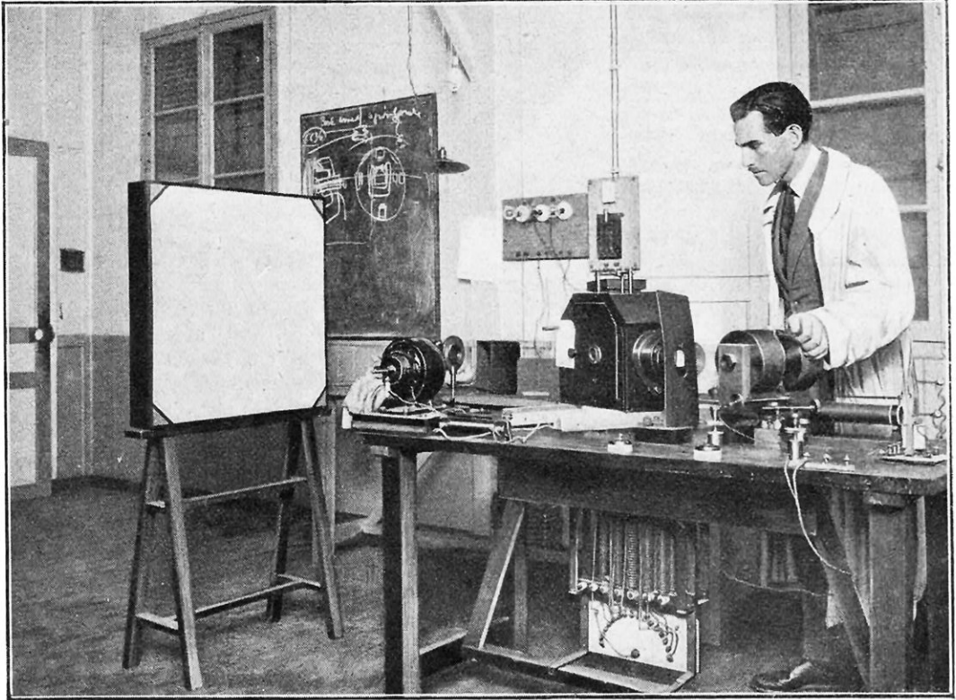
FIG. 10. — ENSEMBLE DES APPAREILS CONSTITUANT LE POSTE RÉCEPTEUR
