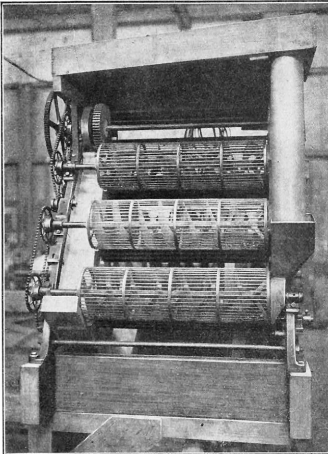
VUE DE FACE DE LA MACHINE, MONTRANT LES VIS D'ARCHIMÈDE A L'INTÉRIEUR DES CYLINDRES EN CAGE D'ÉCUREUIL
