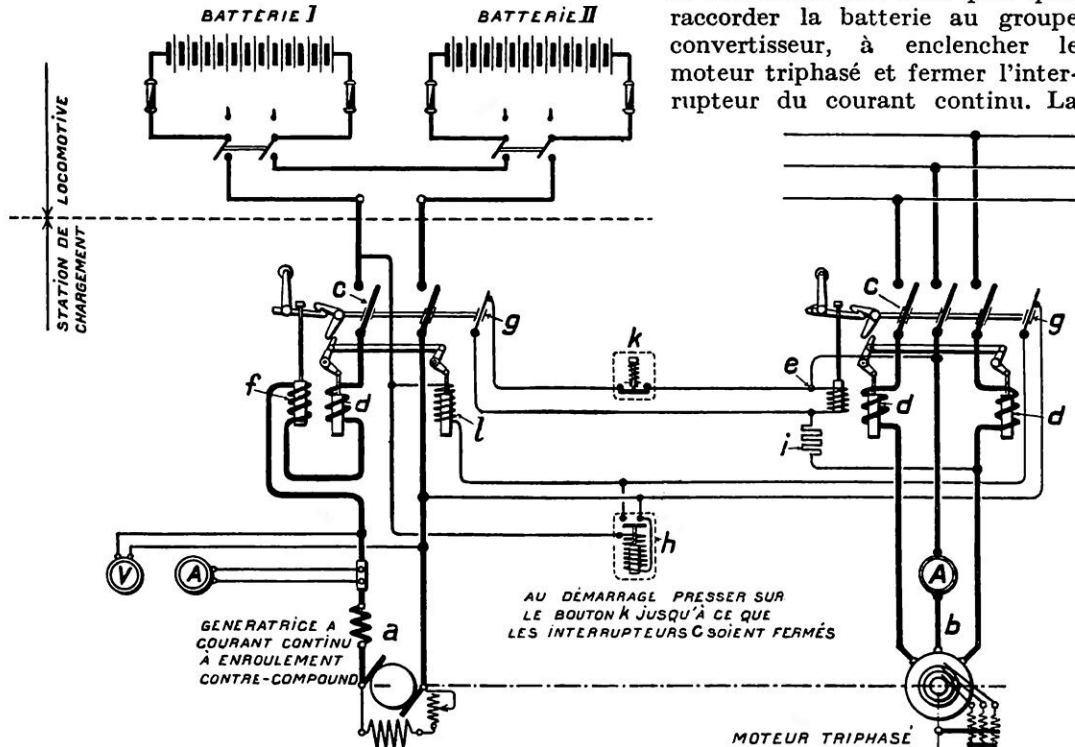
SCHEMA D'UNE STATION MODERNE DE CHARGEMENT AUTOMATIQUE DES ACCUMULATEURS SYSTEME OERLIKON
