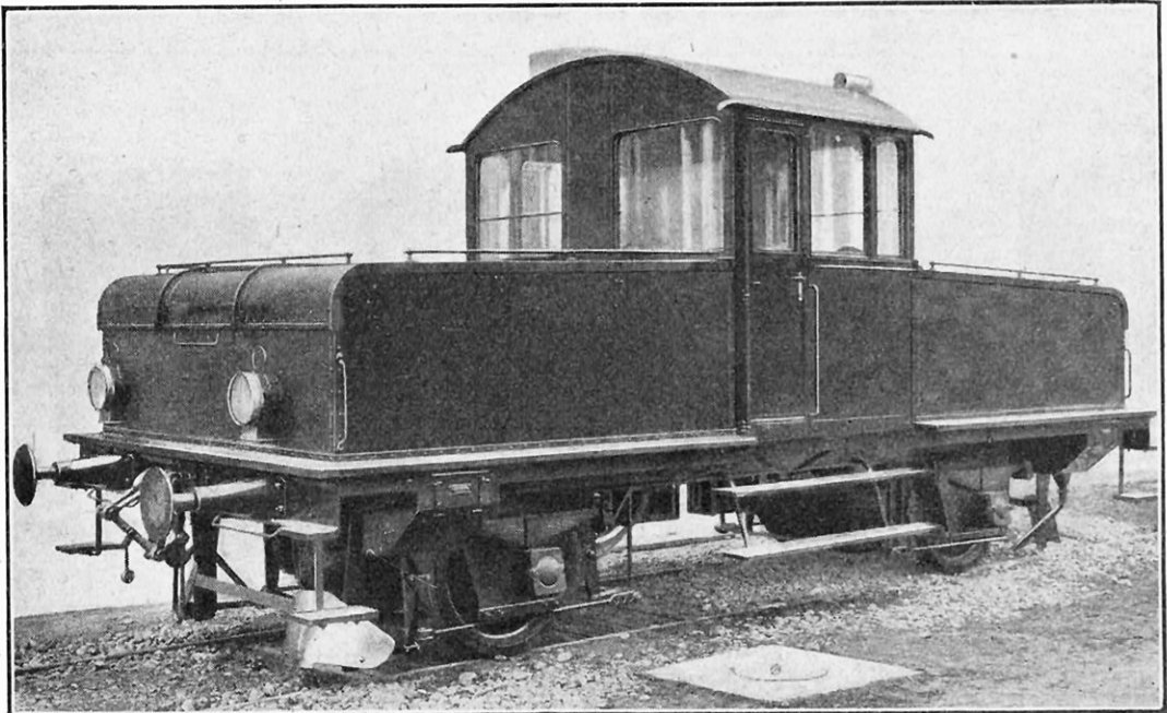
LOCOMOTIVE DE 10 TONNES POUR TRAINS DE CHANTIERS, D'UNE PUISSANCE DE 16 CHEVAUX VITESSE : 5-9 KILOMÈTRES-HEURE ; TENSION : 180 VOLTS
