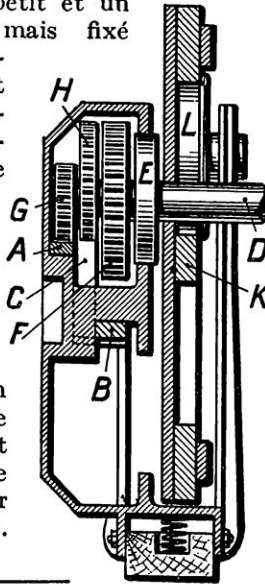
DÉTAIL DE LA BOITE DE VITESSES
