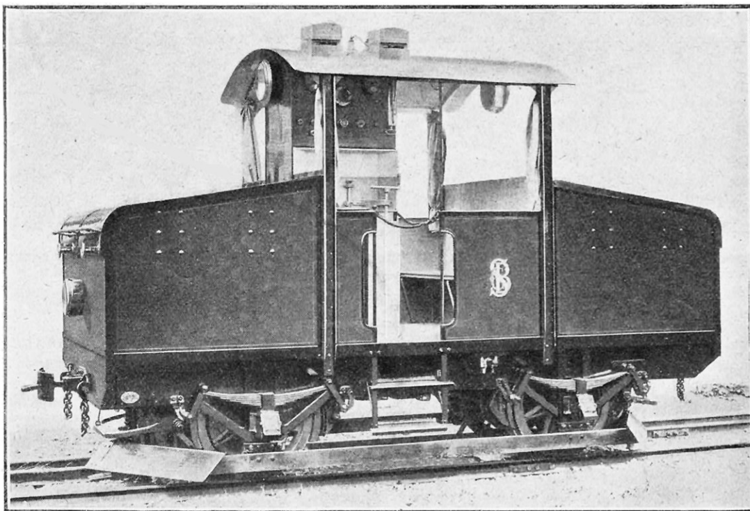
LOCOMOTIVE POUR VOIE ÉTROITE, DE 12 TONNES ET DE 50 CHEVAUX ; VITESSE : 10-15 KILOMÈTRES-HEURE ; TENSION : 300 VOLTS
