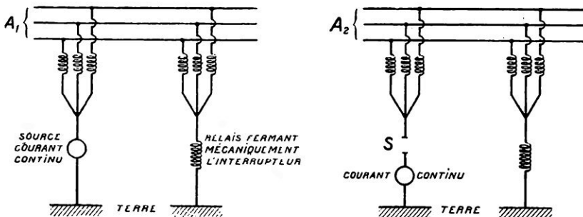
FIG. 7. — UNE ÉMISSION DE COURANT FAITE DANS LE RÉSEAU « A_1 » PEUT DONNER NAISSANCE A UNE ÉMISSION DANS LE RÉSEAU « A_2 », PAR LA FERMETURE DE L'INTERRUPTEUR « S », SANS QUE « A_1 » EN SOIT INFLUENCÉ NI SE TROUVE, EN QUELQUE SORTE, RELIÉ ÉLECTRIQUEMENT A « A_2 »
