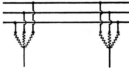
FIG. 4. — MONTAGE AVEC BOBINES DE SELF
