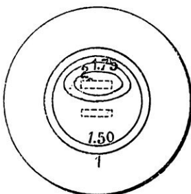
FIG. 13. — ÉTUDE DES VIBRATIONS D'UNE MEMBRANE TÉLÉPHONIQUE, D'APRÈS M. KENNELY
