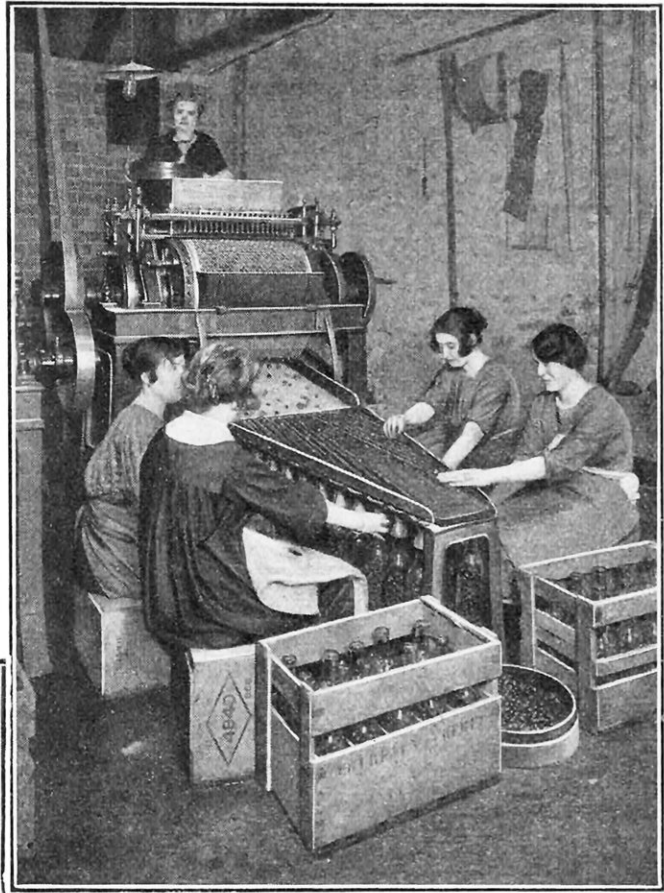
FIG. 10. — DÉNOYAUTEUSE NAVARRE EN PLEINE ACTION
