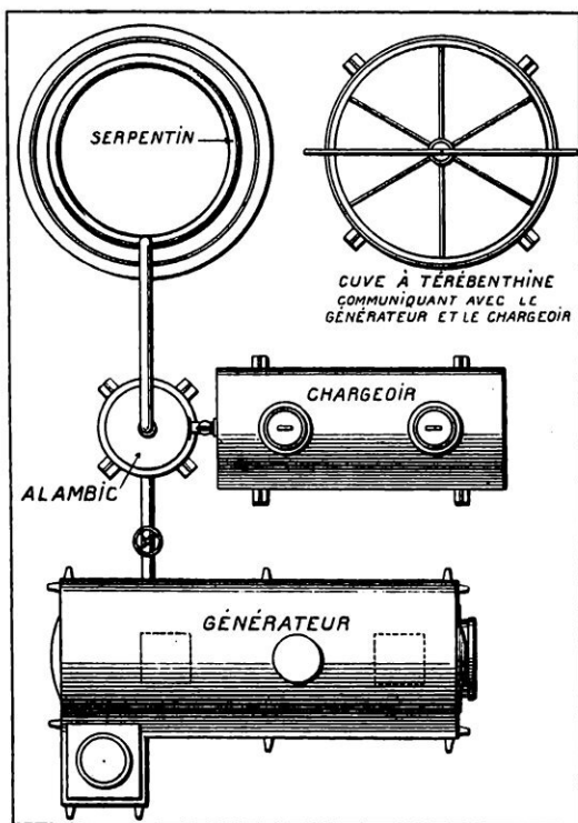
FIG. 4. — VUE D'ENSEMBLE DE L'APPAREIL DE DISTILLATION DALBOUZE
