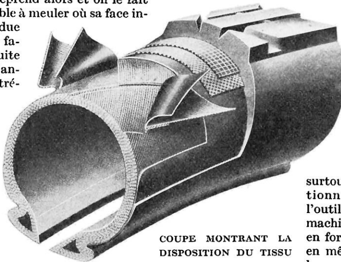
DU CROISSANT D'UN PNEUMATIQUE DUNLOP
