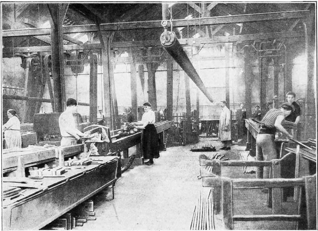
BANC A ÉTIRER LES FILS DE MAGNÉSIUM ET LES FILS D'AUTRES MÉTAUX LÉGERS
