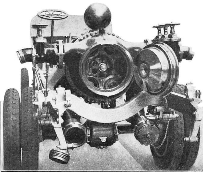
VUE ARRIÈRE DE LA POMPE AUTOMOBILE
