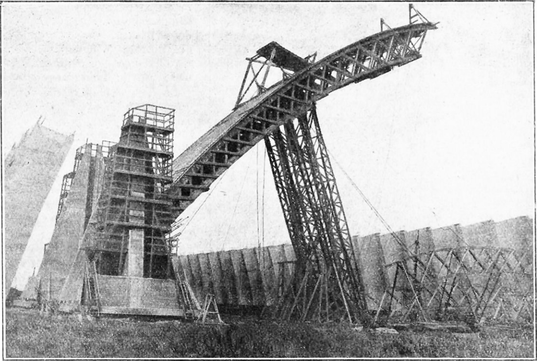
FIG. 8. — MISE EN PLACE D'UN ÉLÉMENT DE CINTRE DU GIGANTESQUE HANGAR Cet élément est maintenu, pendant l'opération, par une bigue que soulèvent des vérins hydrauliques.
