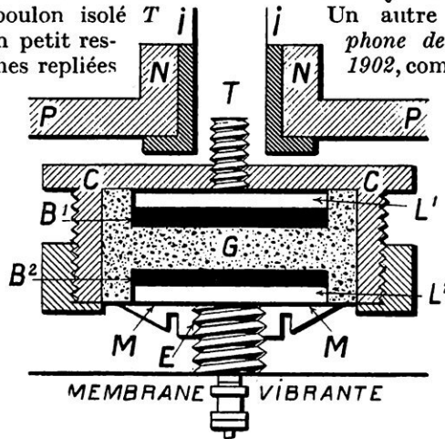
FIG. 8. — DÉTAILS DU MICROPHONE « SOLID-BACK »
