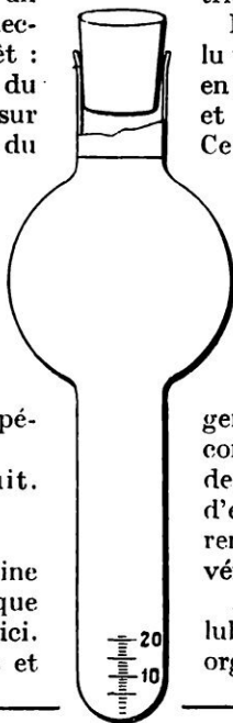
FIG. 1. — APPAREIL POUR LE DOSAGE DES IMPURETÉS DE LA RÉSINE
