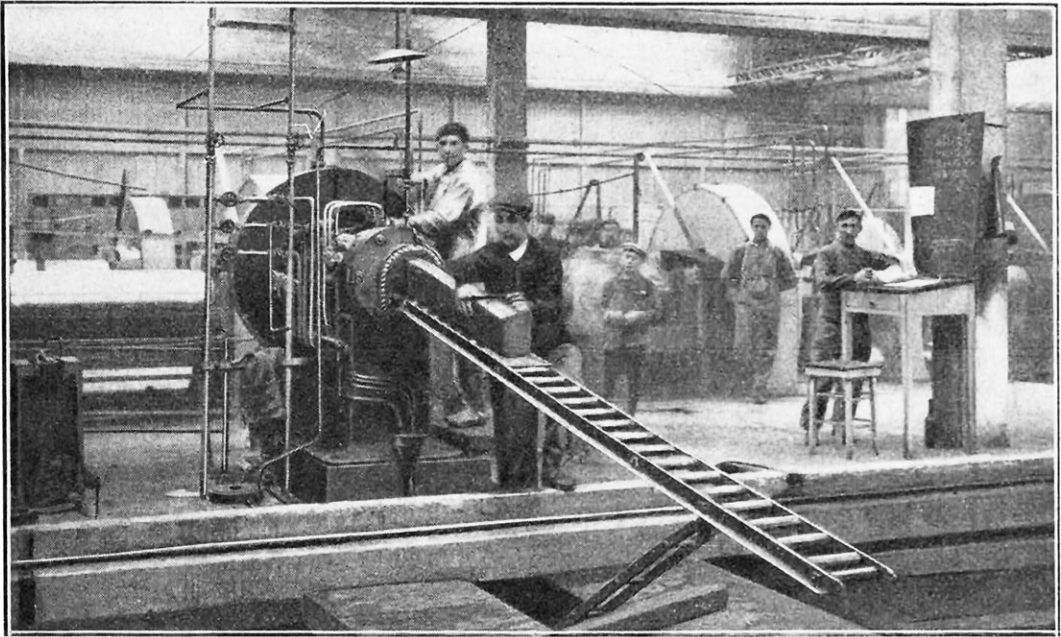
LE BANDAGE SORT, MOULÉ, DE LA BOUDINEUSE, GLISSE SUR UN PLAN INCLINÉ MUNI DE ROULEAUX ET TOMBE DANS LE BASSIN DE REFROIDISSEMENT
