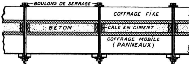
FIG. 10. — FRAGMENT D'UNE COUPE DE LA VOÛTE ENTRE SES COFFRAGES
