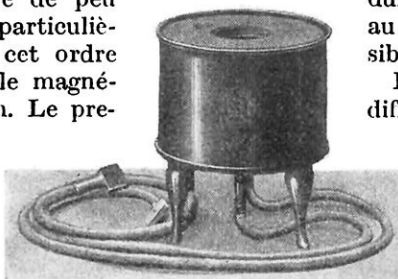
FOUR ÉLECTRIQUE A RÉSISTANCES MÉTALLIQUES POUR PETITE PRODUCTION DE MÉTAUX LÉGERS (TEMPÉRATURE : 1.000 DEGRÉS)
