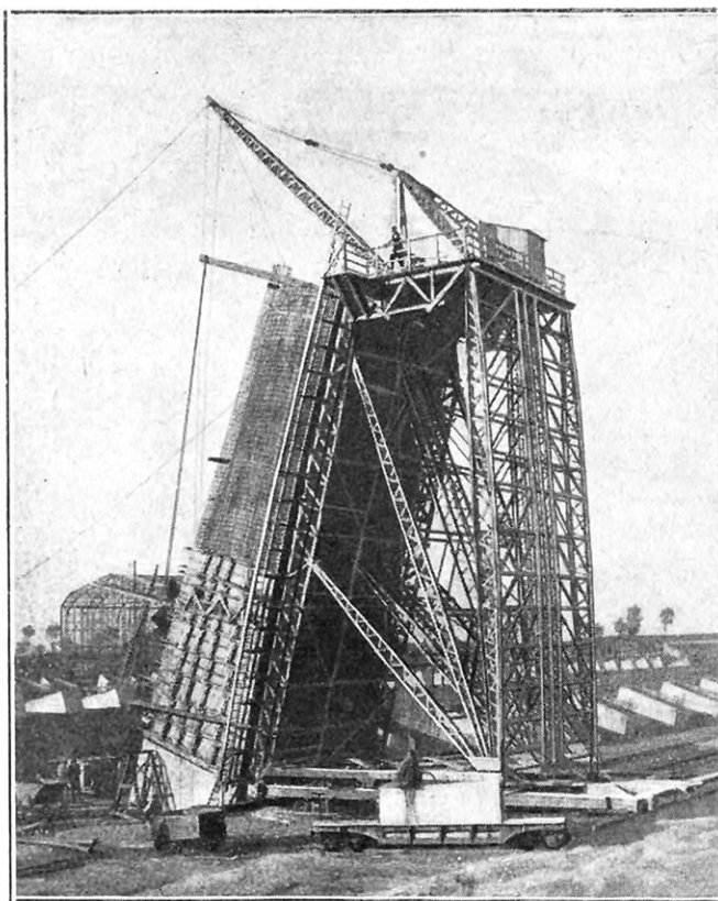
FIG. 6. — ÉCHAFAUDAGE QUI PERMET DE CONSTRUIRE L'ORIGINE DE LA VOUTE JUSQU'À 17 MÈTRES DE HAUTEUR
