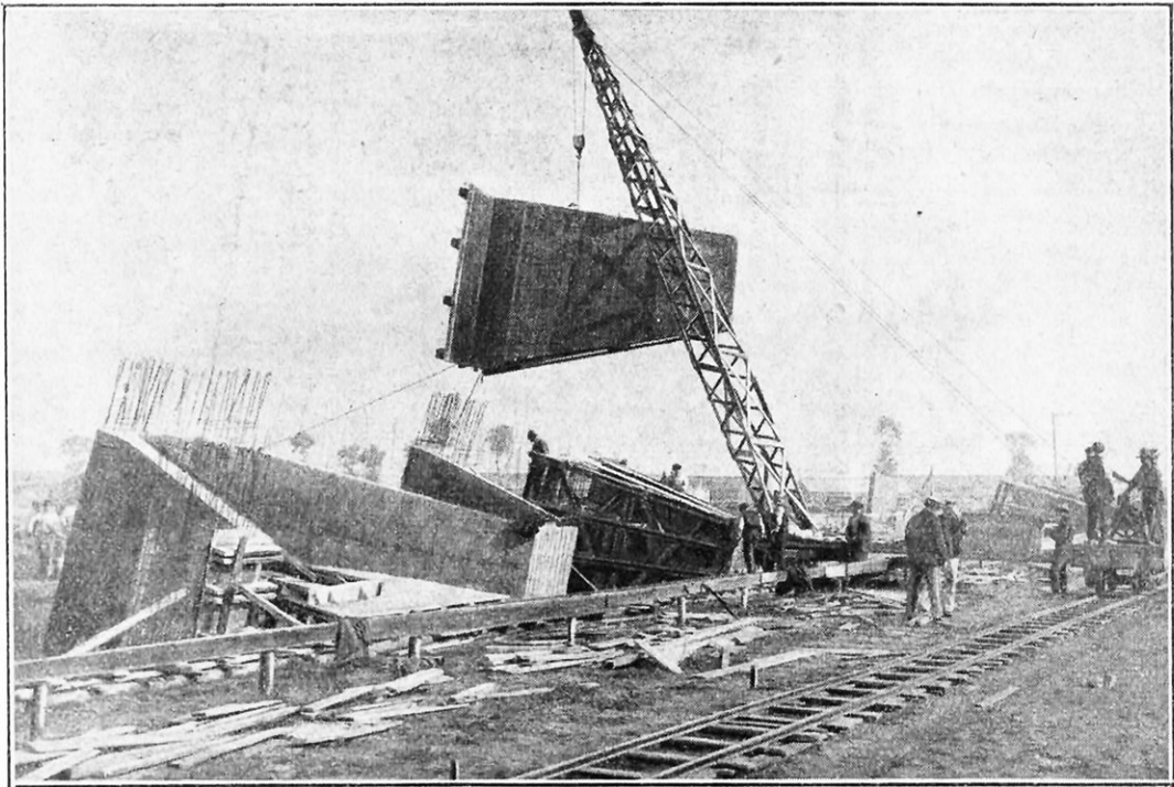
FIG. 4. — CONSTRUCTION DE L'ORIGINE DE LA VOUTE D'UN HANGAR
