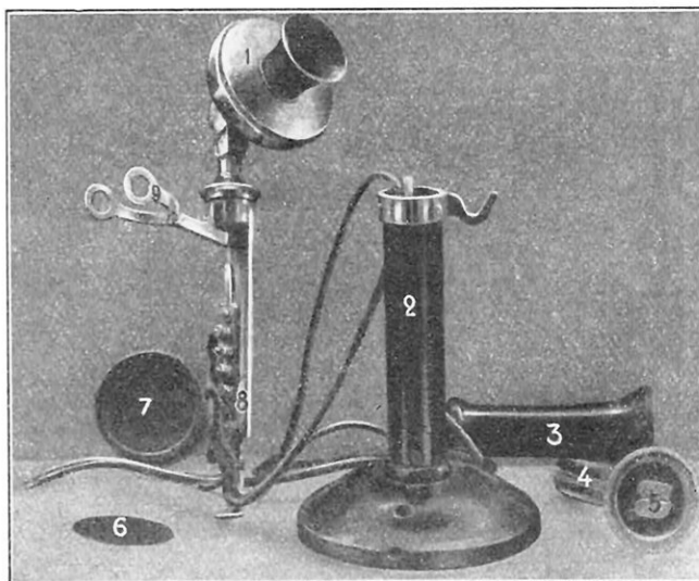
FIG. 22. — POSTE MOBILE TYPE « MT », DÉMONTÉ
