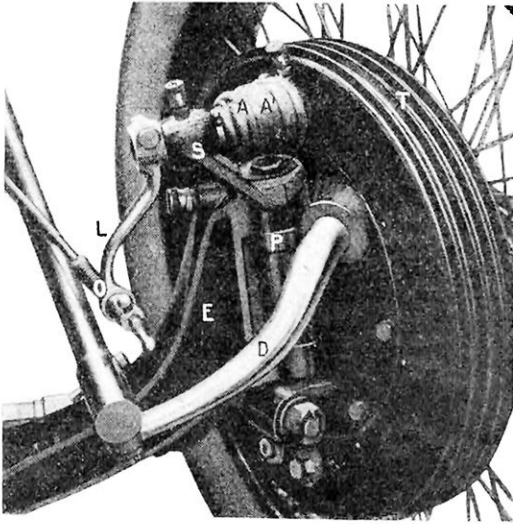
LE FREIN AVANT SYSTÈME L. BOLLÉE
