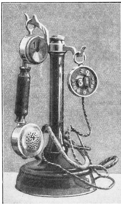
FIG. 20. — POSTE MOBILE ERICSSON Le récepteur indépendant a été démonté pour montrer, en 2, l'aimant permanent et, en 3, les bobines. — 1, récepteur du combiné ; 4, transmetteur microphonique du poste mobile.
