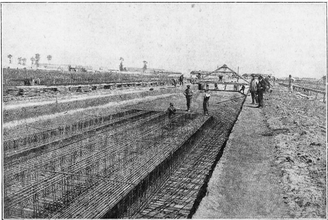
FIG. 3. — CONSTRUCTION D'UNE FONDATION SERVANT DE POINT D'APPUI A LA VOÛTE On remarque la disposition très compliquée du réseau métallique qui sera noyé dans le béton.
