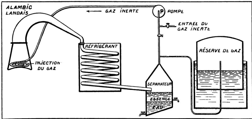
FIG. 6. — VUE SCHÉMATIQUE D'UN APPAREIL A DISTILLATION DANS UN GAZ INERTE
