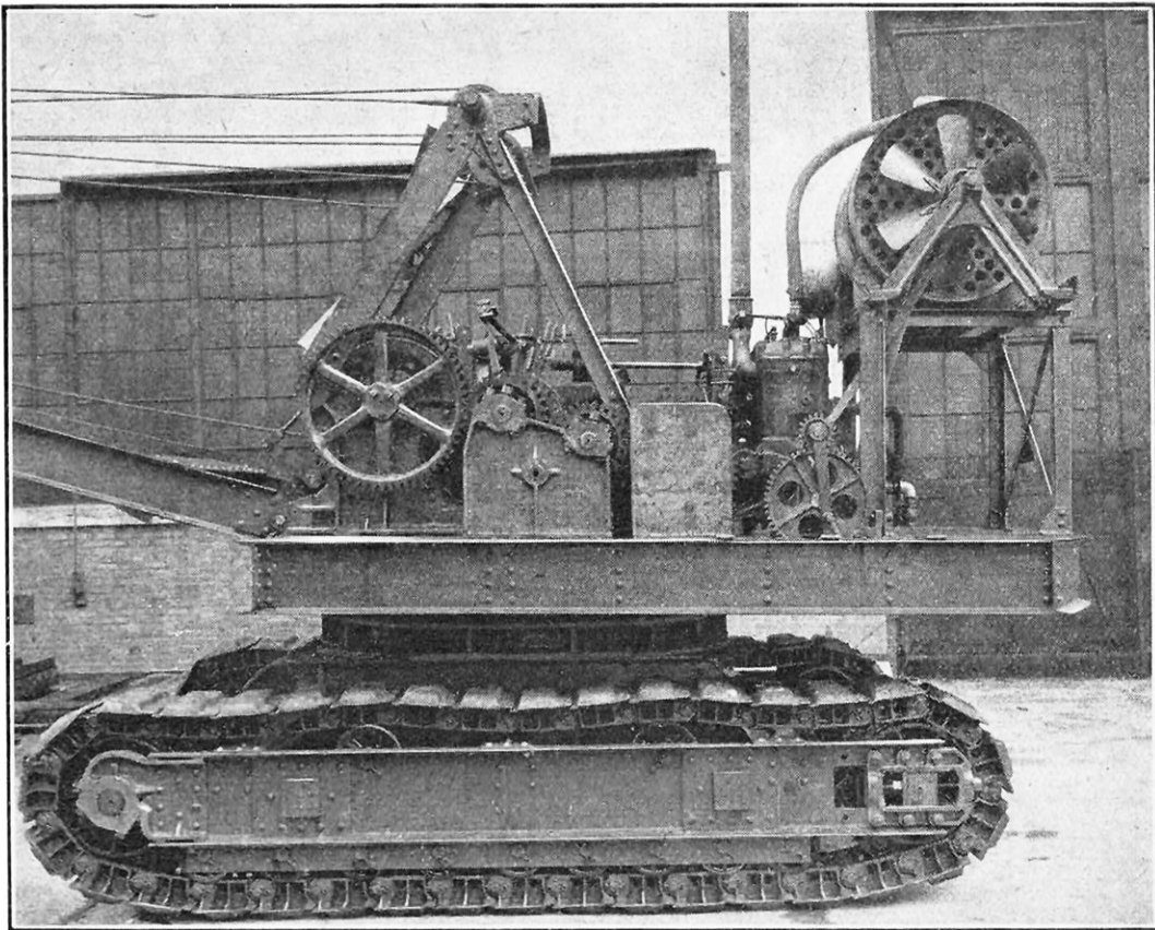
VUE LATÉRALE DE LA MACHINERIE, DU COTÉ OPPOSÉ AUX COMMANDES
