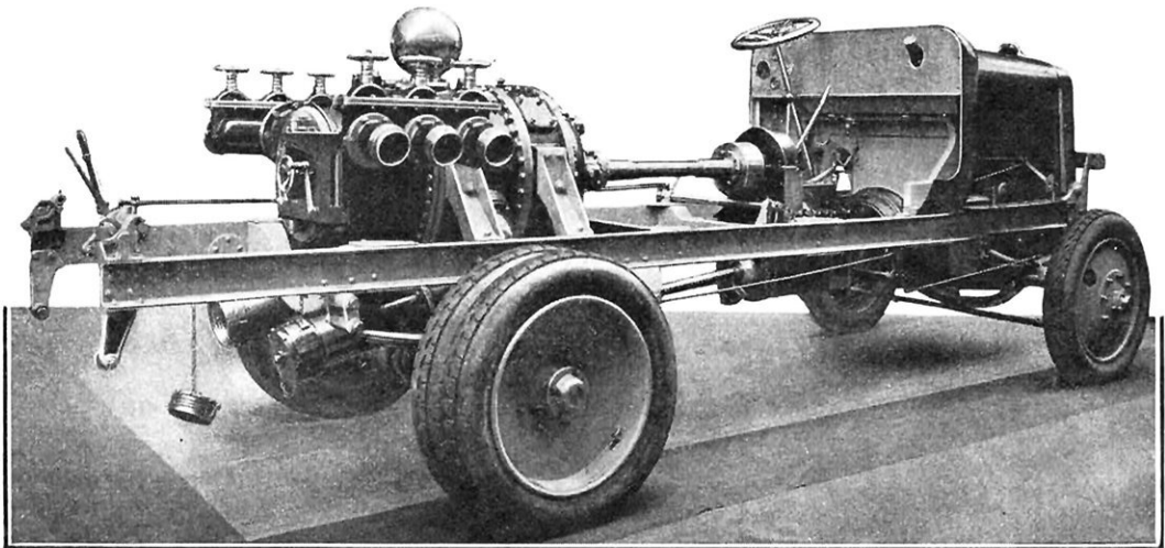
VUE LATÉRALE DE LA POMPE A INCENDIE A GRANDE PUISSANCE
