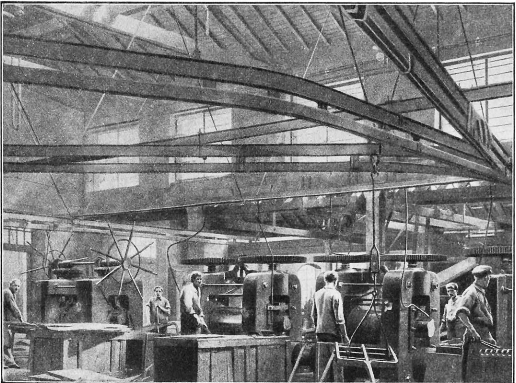
ATELIER DES LAMINOIRS SPÉCIAUX POUR LA TOLE DE MÉTAL LÉGER
