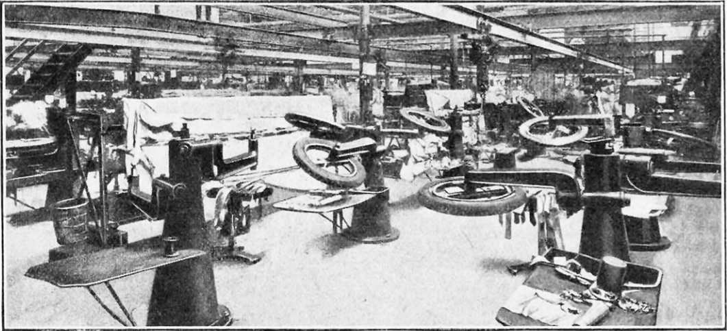
ATELIER DE MONTAGE ET DE DÉGOMMAGE DES CARCASSES D'ENVELOPPES DE PNEUS
