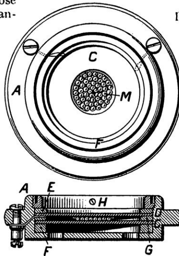
FIG. 7. — MICROPHONE BERTHON . D , C , plaques de charbon serrées entre trois anneaux de caoutchouc EFG ; M , grenaille de charbon serrée entre les deux plaques D et C ; A , boîtier. — Au-dessus, vue en plan ; en bas, coupe.
