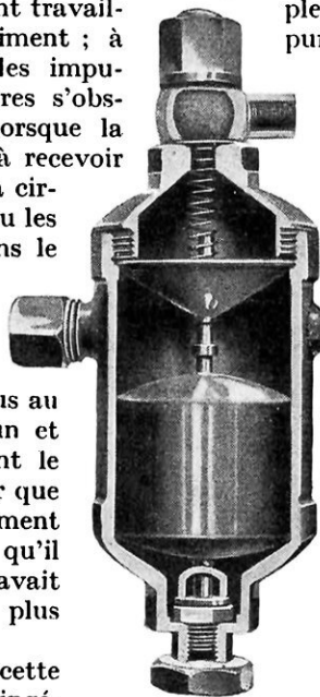
VUE INTÉRIEURE DU FILTRE
