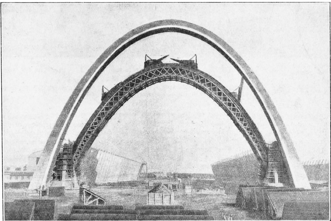
FIG. 11. — LE PREMIER ÉLÉMENT DE LA VOÛTE EST COMPLÈTEMENT TERMINÉ
