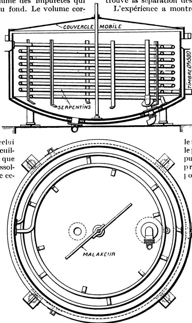
FIG. 2. — ÉLÉVATION ET PLAN D'UNE CUVE A TÉRÉBENTHINE
