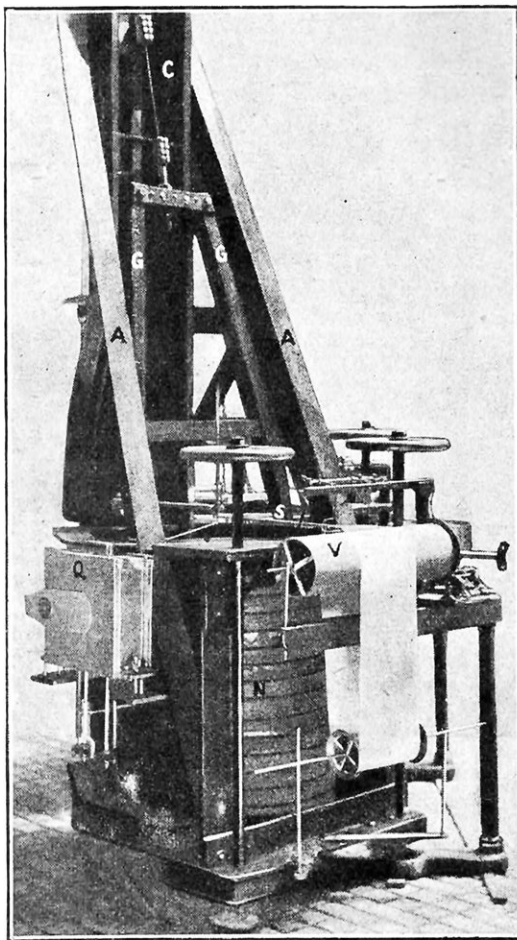
LE SISMOGRAPHE DE L'OBSERVATOIRE DU PARC SAINT-MAUR QUI A ENREGISTRÉ LE GRAND TREMBLEMENT DE TERRE DU CHILI DONT NOUS REPRODUISONS LE SISMOGRAMME, PAGE 102.
