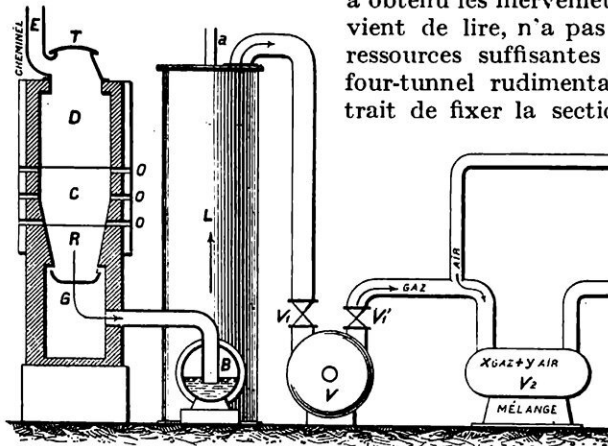
SCHÉMA DU GAZOGÈNE QUI ALIMENTE LE FOUR A PORCELAINÉ
