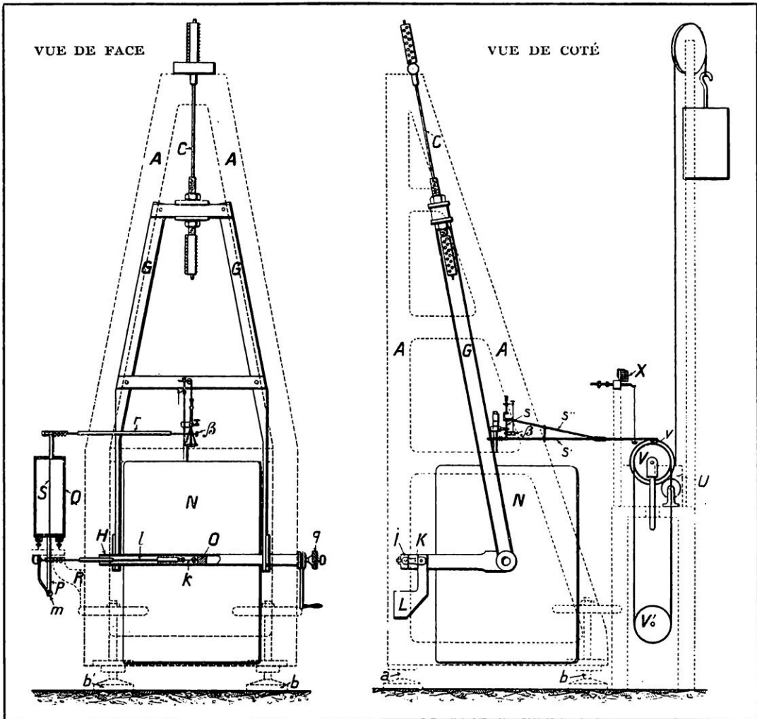
SCHÉMAS D'UN SISMOGRAPHE DU TYPE MAINKA AMORTI, DERNIER MODÈLE
