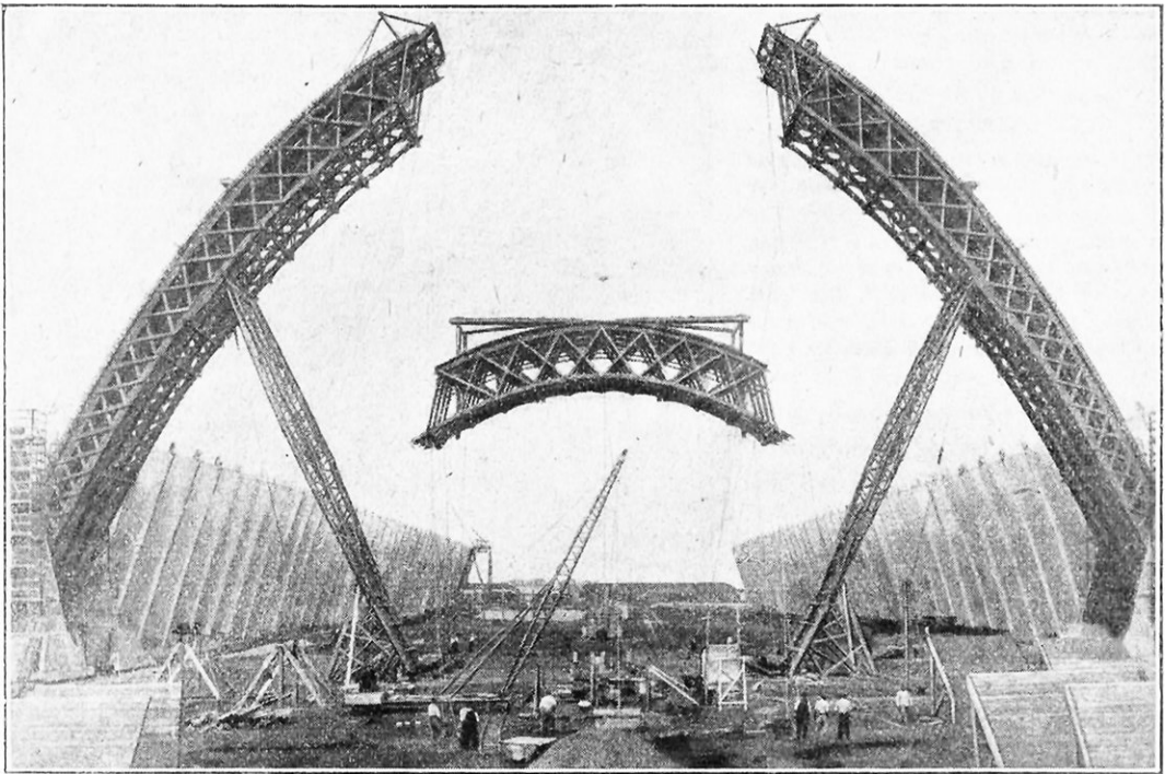
FIG. 9. — MISE EN PLACE DE LA CLÉ DU CINTRE (ARRIVÉE A MI-HAUTEUR) Les deux premiers arcs du cintre, soutenus dans l'espace par deux bigues, servent de points d'appuis pour soulever la clé du cintre à l'aide de câbles et de puissants cabestans.
