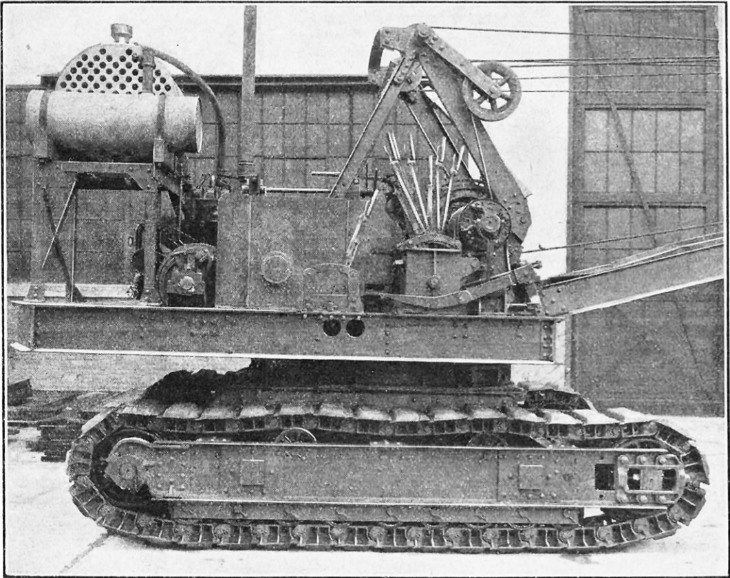
VUE LATÉRALE DES APPAREILS MOTEURS, LA CABINE ÉTANT ENLEVÉE
