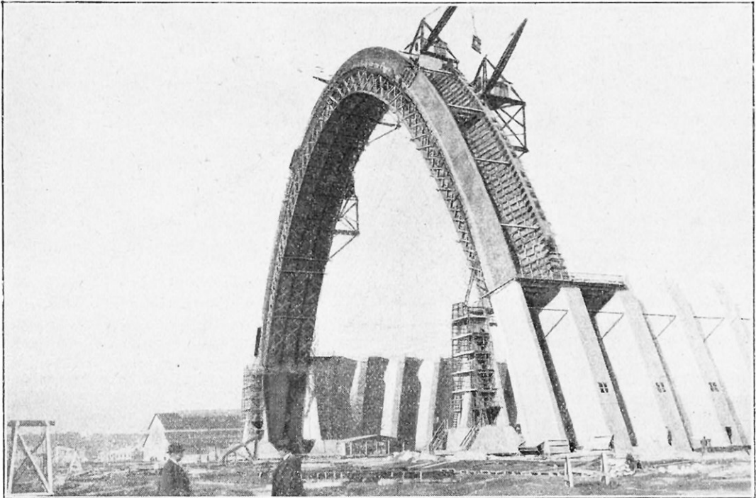
FIG. 12. — CONSTRUCTION DU DEUXIÈME ÉLÉMENT DE VÔUTE QUI CONSTITUE, EN RÉALITÉ, AVEC LE PRÉCÉDENT, LE PREMIER ÉLÉMENT « ZORÈS »
