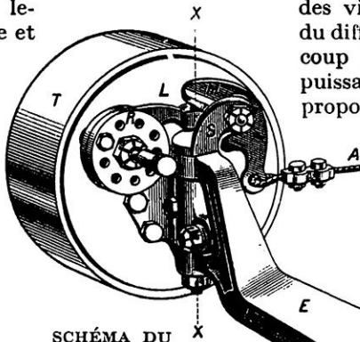
SCHÉMA DU FREIN SYSTÈME SLIM
