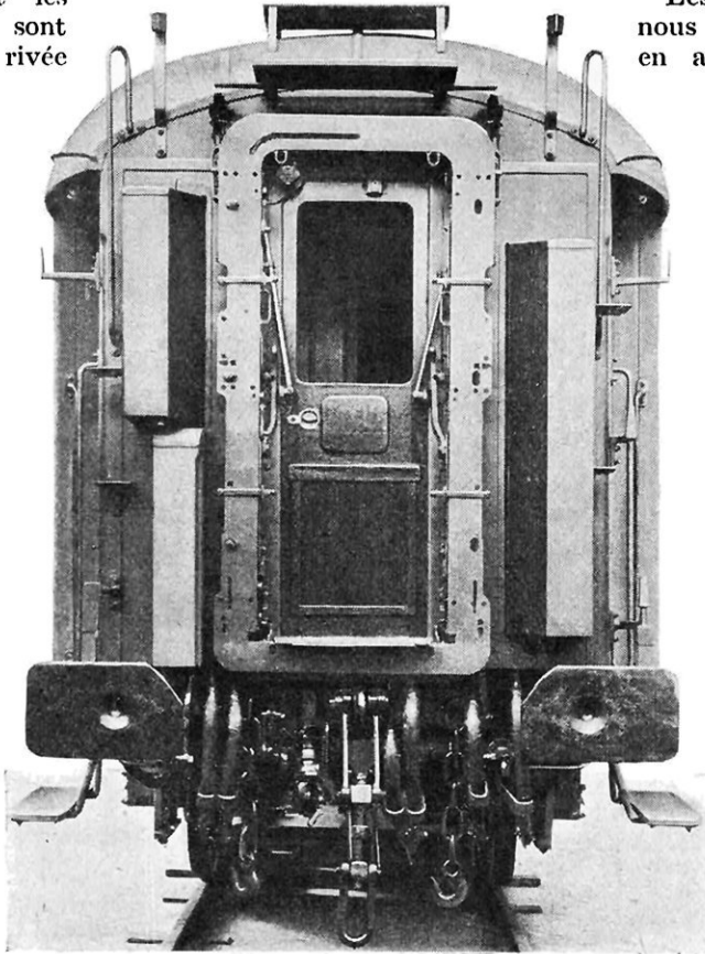
VUE AVANT DE L'UNE DES NOUVELLES VOITURES-LITS Les appareils d'attelage et de choc sont nettement visibles, ainsi que le soufflet qui relie les voitures deux à deux.
