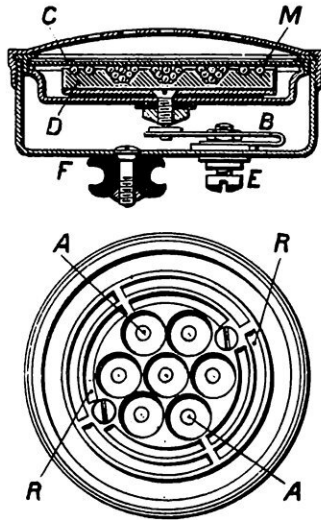
FIG. 10. — CAPSULE MICROPHONIQUE AMOVIBLE 1910
