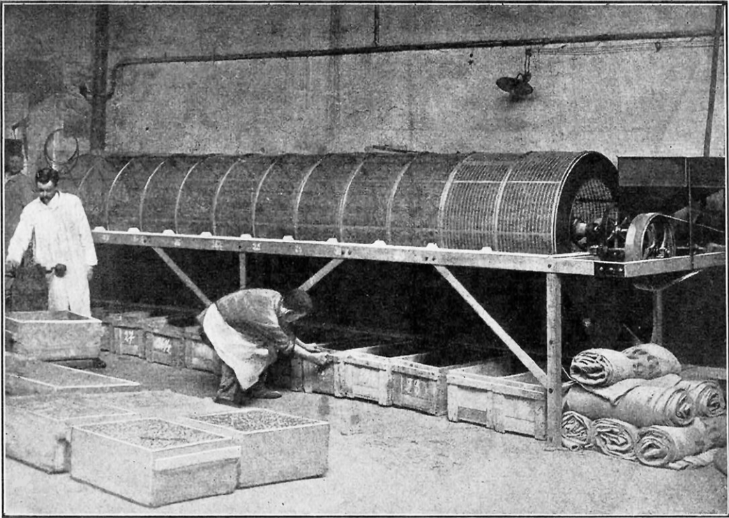
FIG. 3. — GRAND APPAREIL CRIBLEUR CLASSANT LES POIS EN CINQ CATÉGORIES Suivant leur grosseur, les pois tombent dans des caisses placées sous le cribleur et sont automatiquement classés en extra-fins, fins, mi-fins, moyens et gros.
