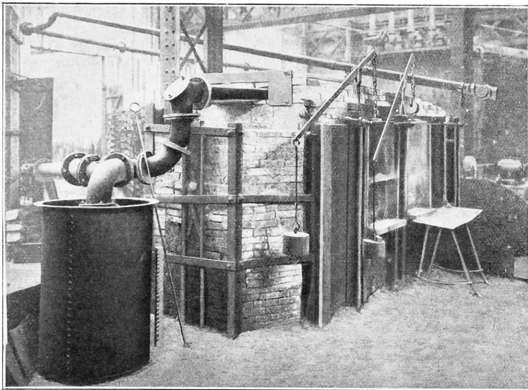
LE FOUR À PORCELAINÉ ALIMENTÉ AU GAZ DE BOIS VU DU CÔTÉ DU GAZOGÈNE
