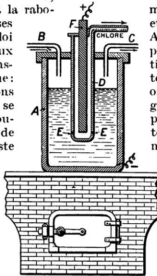
FOUR DE GRAETZEL POUR LA FABRICATION DU MAGNÉSIUM A, récipient en fonte placé sur un foyer ; B et C, tubes d'entrée et de sortie d'un gaz inerte ou réducteurs ; D, vase poreux ; E, orifices pour la circulation du sel fondu ; F, anode en graphite ; G, tube de dégagement du chlore formé par électrolyse.
