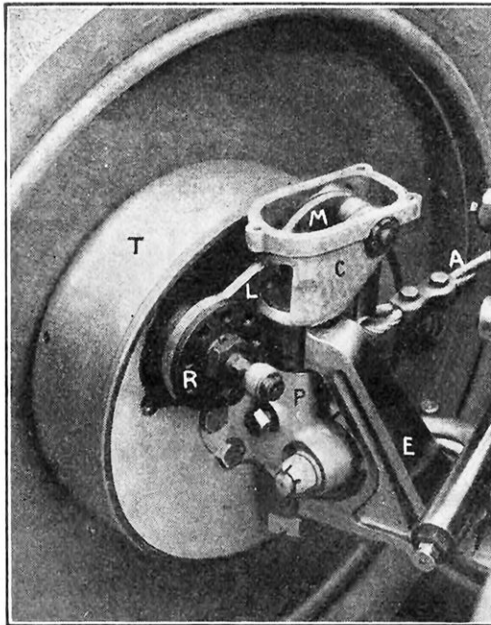
DISPOSITIF DU FREIN AVANT SLIM
