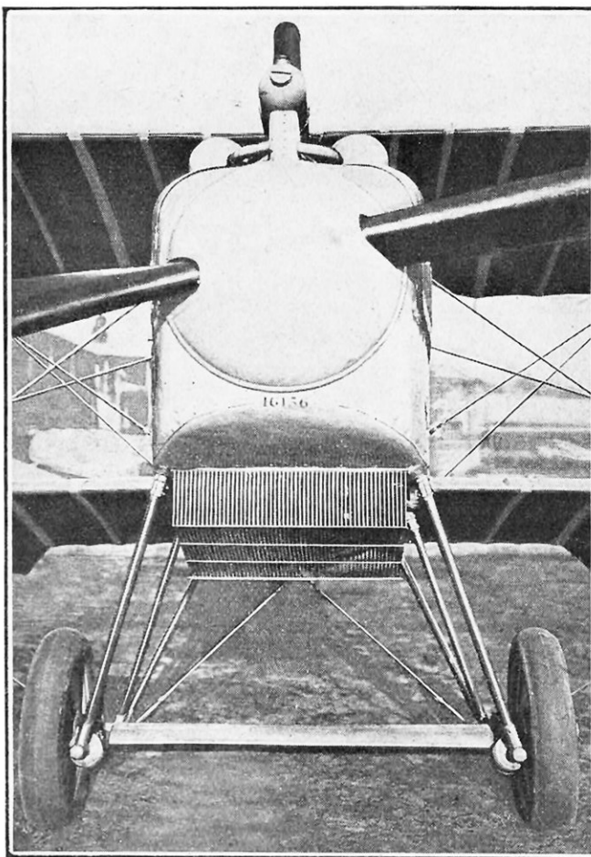
LE RADIATEUR A LAMELLES SE PLACE SOUS LE FUSELAGE
