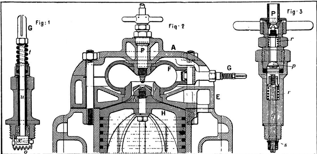
VUE EN COUPE DU MOTEUR A HUILES LOURDES ET DE SES ACCESSOIRES
