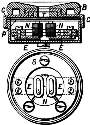
FIG. 2. — TÉLÉPHONE ADER B, pavillon ; T, trou central du pavillon ; A, excitateur en fer doux ; C, couvercle du boîtier ; P, plaque vibrante ; G, aimant circulaire ; E E, équerres en fer doux prolongeant les pôles de l'aimant ; N N bobines.
