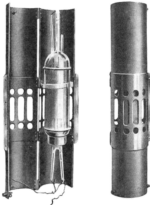
LAMPE D'ÉMISSION DE 5.000 VOLTS A gauche, l'étui ouvert; à droite, l'étui fermé.
