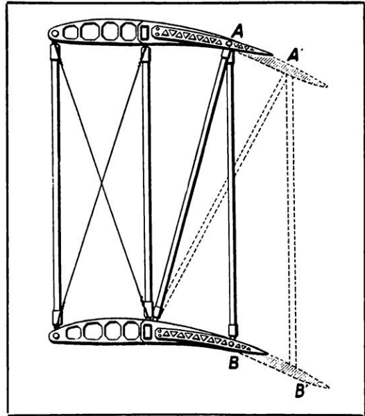
SCHÉMA DU DÉPLOIEMENT DE L'AILE
