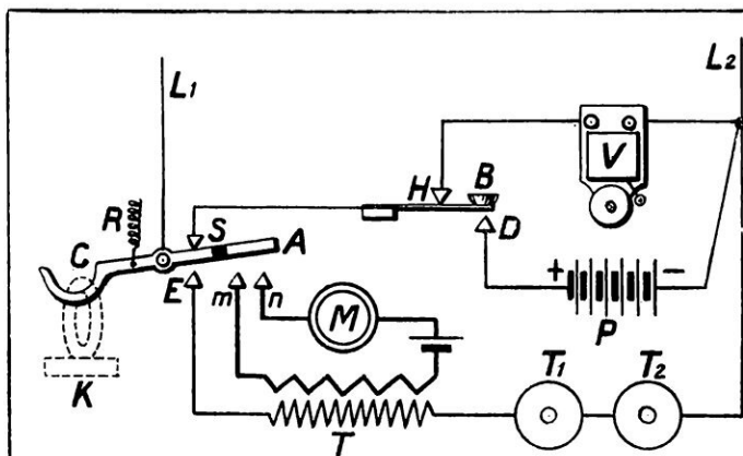
FIG. 16. — SCHEMA GÉNÉRAL DE L'INSTALLATION D'UN POSTE TÉLÉPHONIQUE URBAIN
