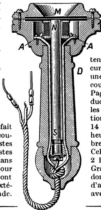
FIG. 1. — MODÈLE PRIMITIF DU TÉLÉPHONE BELL
