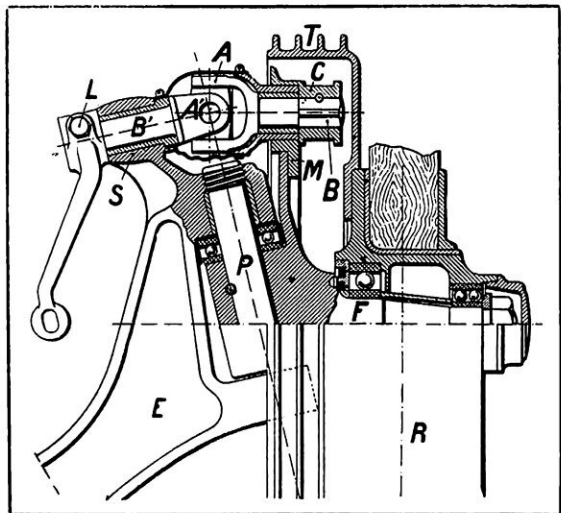
VUE EN COUPE DU FREIN L. BOLLÉE
