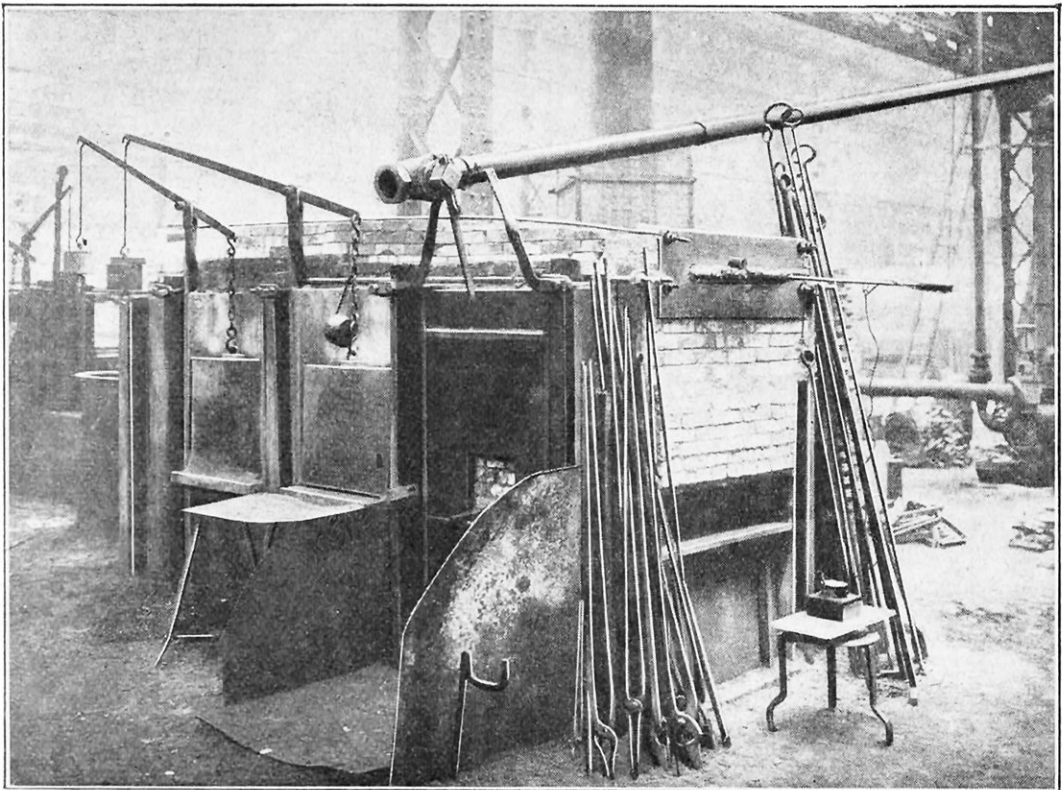
FACE DE TRAVAIL DU FOUR A PORCELAINES ALIMENTÉ AU GAZ DE BOIS
