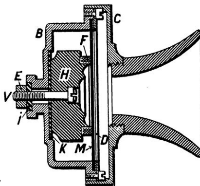
FIG. 9. — MICROPHONE « SOLID-BACK », MODÈLE 1902
