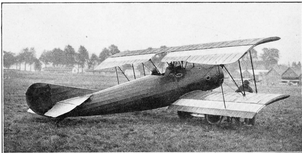
L'AVION BELLANGER-BILL A SURFACE VARIABLE PENDANT LES ESSAIS
