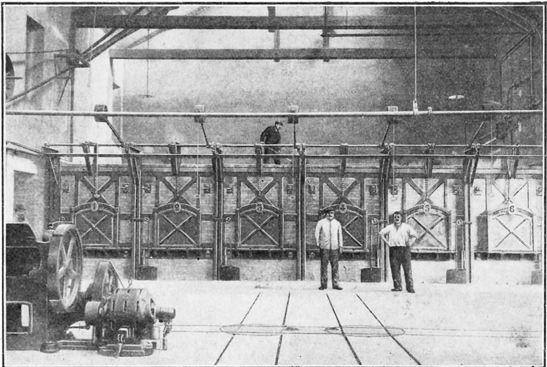
BATTERIE DE SIX FOURS A MOUFLE POUR LA RECUISSON DU MÉTAL LÉGER
