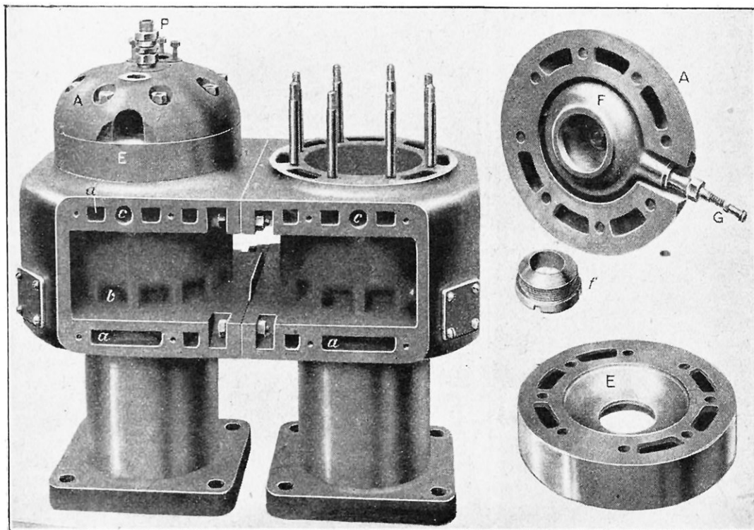
VUE INTÉRIEURE DES CYLINDRES DU MOTEUR DÉMONTÉ
