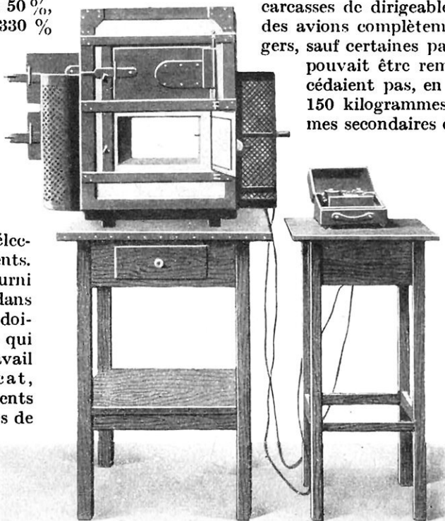
FOUR ÉLECTRIQUE A DOUBLE MOUFLE ET A RÉSTANCES GRAPHITIQUES POUR TEMPÉRATURES JUSQU'A 1.300°
