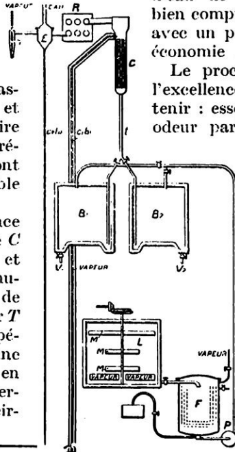
FIG. 7. — APPAREIL A DISTILLATION DANS LE VIDE
