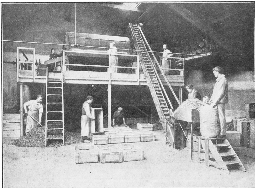
FIG. 1. — SALLE DE RÉCEPTION DES POIS DANS UNE FABRIQUE DE CONSERVES
