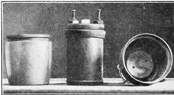
LA LAMPE SE DÉMONTE EN UN RIEN DE TEMPS
