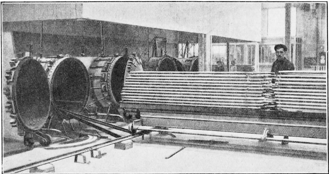
UN LOT DE CHAMBRES A AIR, MONTÉES SUR DES TUBES MÉTALLIQUES, VA ÊTRE INTRODUIT DANS L'UN DES AUTOCLAVES QUE L'ON VOIT SUR CETTE PHOTOGRAPHIE
