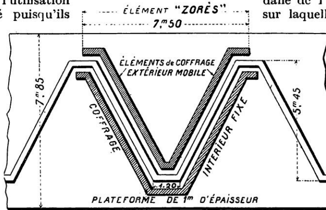
FIG. 2. — PROFIL DE LA VOÛTE D'UN HANGAR
