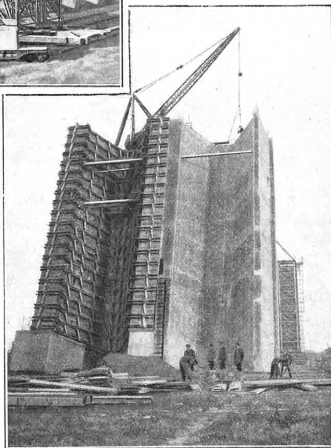
FIG. 7. — LA CONSTRUCTION DU PREMIER ÉLÉMENT DE 17 MÈTRES EST COMPLÈTEMENT TERMINÉE.
