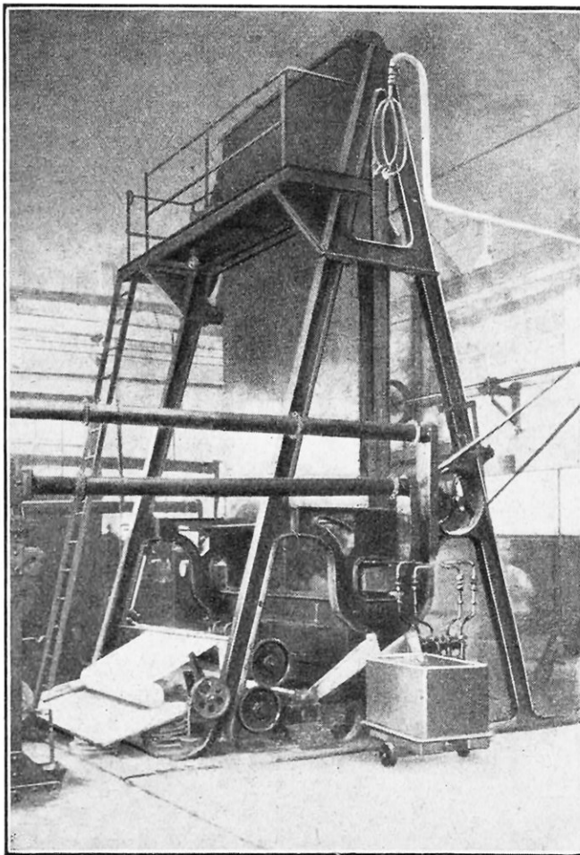
MACHINE A GOMMER LE TISSU « CORD »
