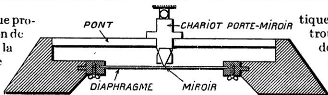
FIG. 12. — APPAREIL DE M. KENNELY POUR L'ÉTUDE DES PLAQUES VIBRANTES
