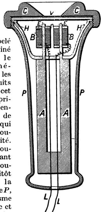
FIG. 3. — RÉCEPTEUR DU « MATÉRIEL TÉLÉPHONIQUE » TYPE « WESTERN ELECTRIC »
