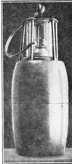
LA LAMPE DE MINEUR MONTÉE AVEC SON ACCUMULATEUR
