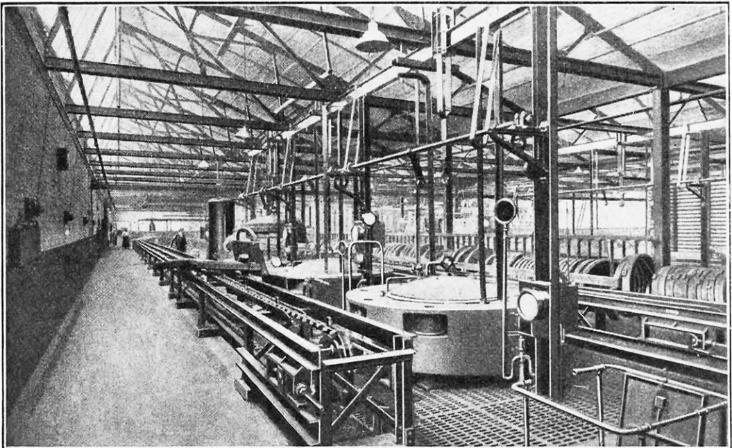
MONTÉS SUR LEUR CERCLE DE FER, LES BANDAGES SONT AMENÉS AUX AUTOCLAVES
