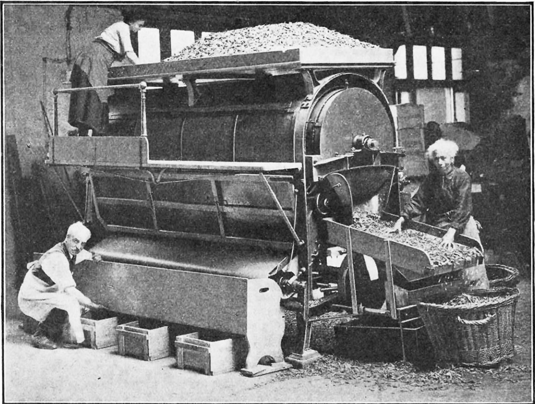
FIG. 2. — MACHINE A ÉCOSSEUR A GRAND RENDEMENT, SYSTÈME NAVARRE
