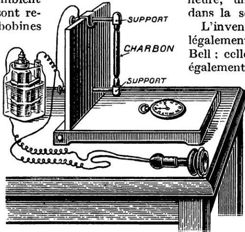
FIG. 4. — LE MICROPHONE HUGHES
