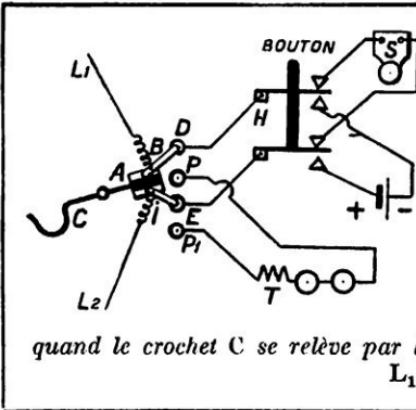
FIG. 17. — DISPOSITIF SEMBLABLE AU PRÉCÉDENT (FIG. 16) DANS LEQUEL LE LEVIER D'APPEL A ÉTÉ REMPLACÉ PAR UN BOUON
