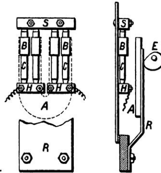
FIG. 6. — MICROPHONE P. BERT ET D'ARSONVAL . C , charbons verticaux ; S , barre supérieure en charbon ; B , chemise de fer doux entourant les charbons ; H , H , barres inférieures en charbon ; A , aimant en fer à cheval fixé sur une lame de laiton R ; E , came permettant d'approcher ou d'éloigner l'aimant A de la chemise B des charbons. — A gauche, vue en plan ; à droite, coupe.
