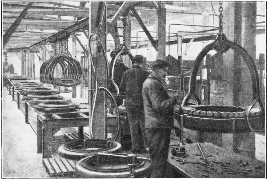
DÉMOULAGE DES PNEUS RAMENÉS DES AUTOCLAVES PAR UN RAIL AÉRIEN
