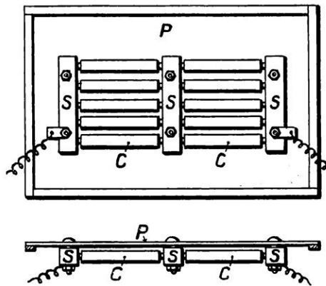
FIG. 5. — LE MICROPHONE ADER
