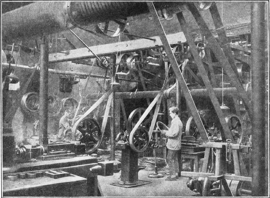
MACHINES A FABRIQUER LES RIVETS EN MÉTAL LÉGER
