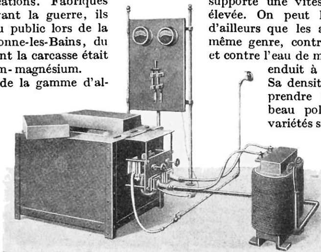
FOUR A CREUSET A RÉSISTANCES GRAPHITIQUES (1.500°) A droite est le transformateur et, au-dessus, le tableau portant les manettes, l'ampèremètre et le voltmètre.
