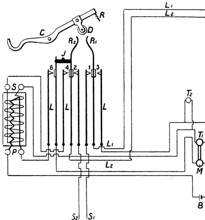
FIG. 18. — APPLIQUE MURALE, MODÈLE 1910
