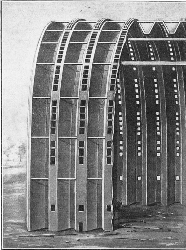
FIG. 1. — VUE PARTIELLE DE L'UN DES NOUVEAUX HANGARS A DIRIGEABLES DU PORT D'AVIATION D'ORLY
