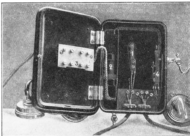
FIG. 14. — POSTE TÉLÉPHONIQUE MURAL ÉRICSSON 1, commutateur d'appel ; 2, condensateur ; 3, plaque de liaison entre les fils intérieurs et ceux venant de l'extérieur ; 4, commutateur actionné par le crochet extérieur 5.
