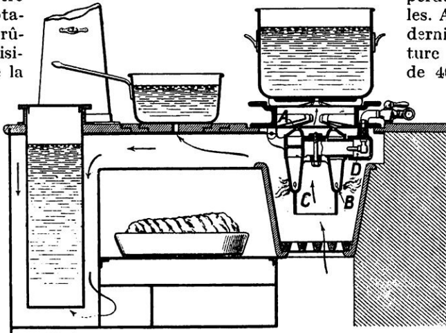
COUPE D'UNE CUISINIÈRE UTILISANT LE BRULEUR A GAZ
