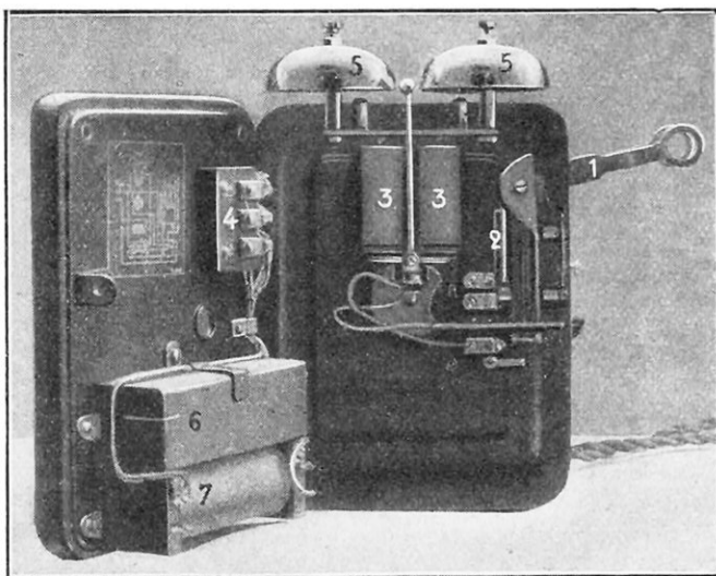
FIG. 19. — POSTE MURAL TYPE « MATÉRIEL TÉLÉPHONIQUE » 1, levier commutateur ; 2, ressorts du commutateur ; 3, bobines de la sonnerie magnétique ; 4, plots d'attache des fils ; 5, timbres de la sonnerie ; 6, condensateur ; 7, bobine transformatrice.
